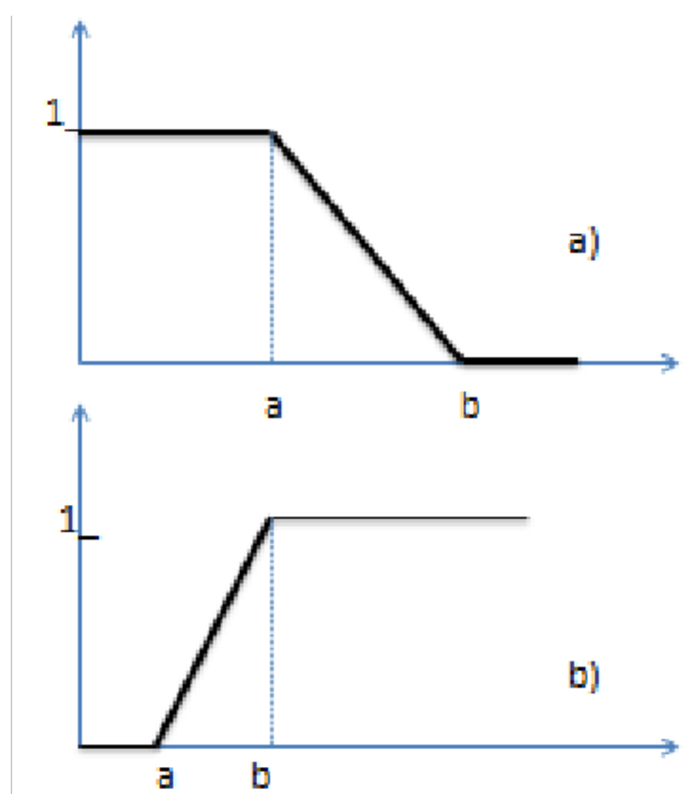
Рисунок 2 - Графики линейной Z-образной (a) и S-образной (b) функций принадлежности
