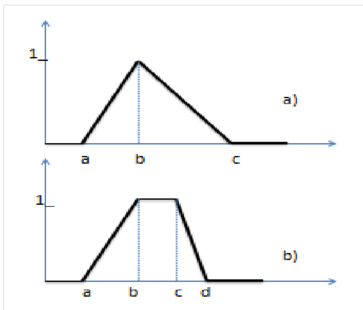
Рисунок 1 - Графики функций принадлежности треугольной (а), трапецевидной (b)
