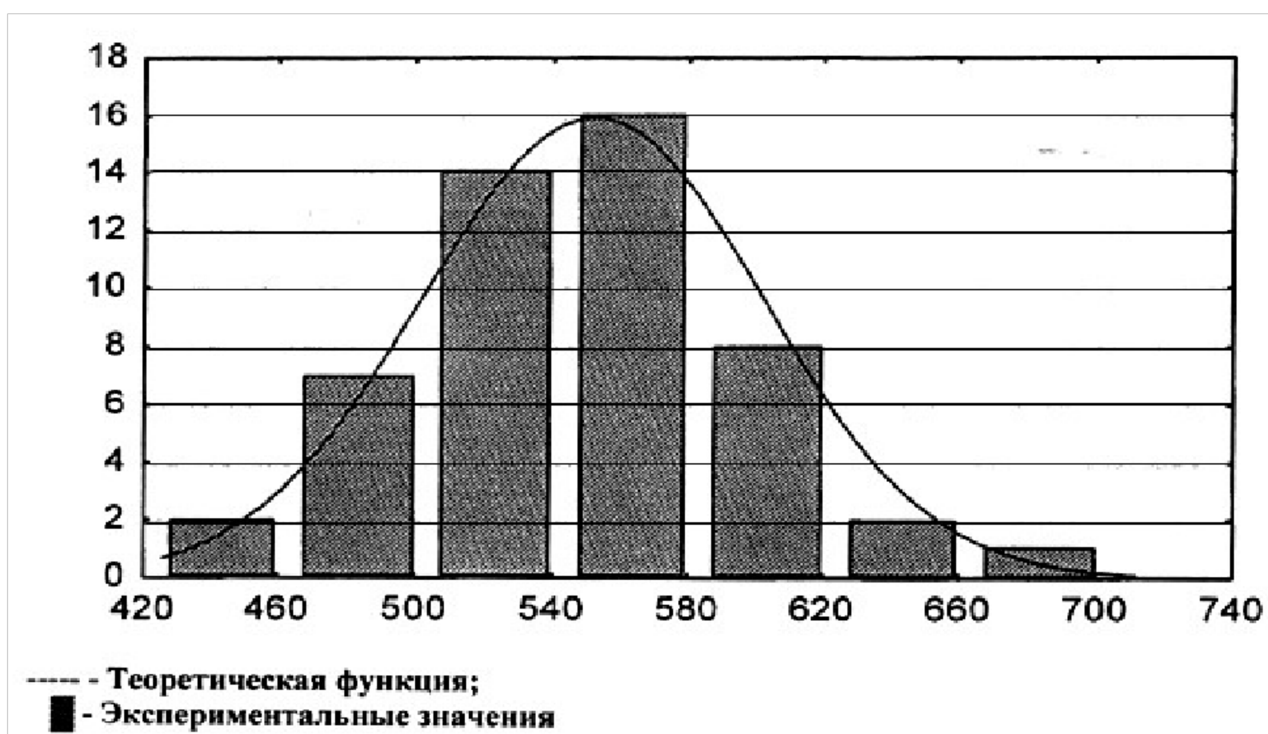
Рисунок 1 – Сравнение эмпирических и теоретических частот
