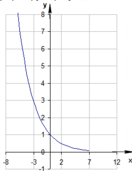
График функции y = a^x , если 0 < a < 1
