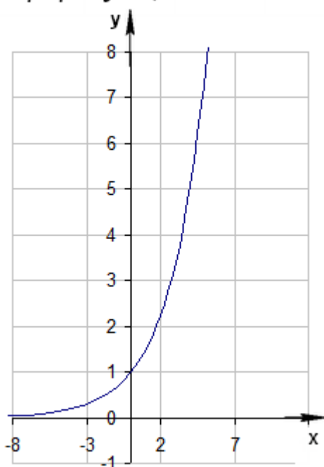
График y = a^x , если a > 1
