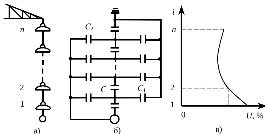
Рисунок 1.1 – Гирлянда подвесных изоляторов:
