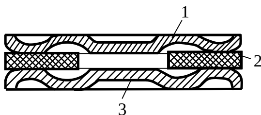
Рисунок 5.6 – Единичный искровой промежуток с неподвижной дугой
