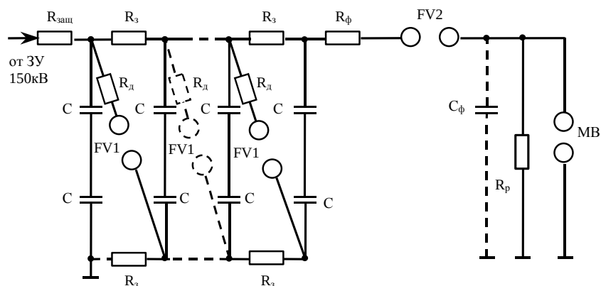
Рисунок 7.3 – Принципиальная схема генератора 750 кВ
