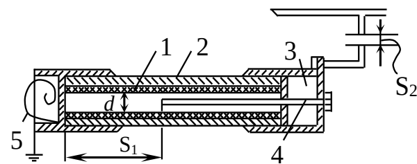
Рисунок 5.2 – Трубчатый разрядник
