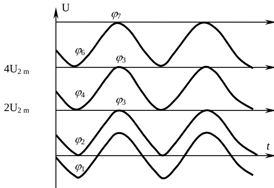
Рисунок 6.5 – Изменение потенциалов в различных точках схемы трехступенчатого выпрямителя в установившемся режиме
