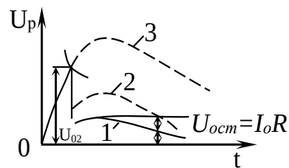
Рисунок 5.3 – Определение остающегося напряжения разрядника
