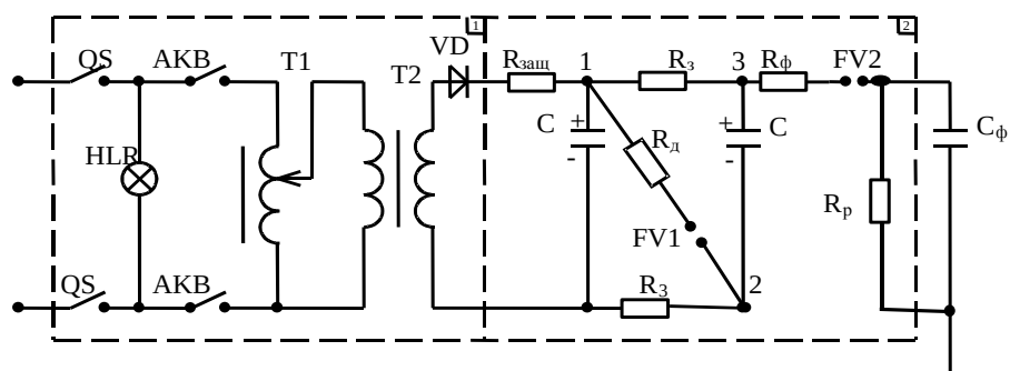
Рисунок 7.2 – Схема ГИН
