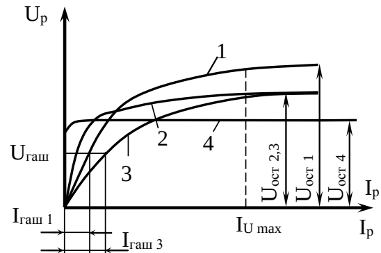
Рисунок 5.5 – Вольтамперная характеристика разрядника.
