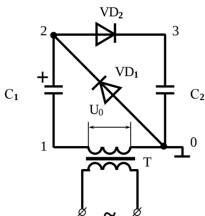
Рисунок 6.1 – Схема одной ступени каскадного выпрямителя
