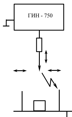
Рисунок 8.4 – принципиальная схема испытательной установки
