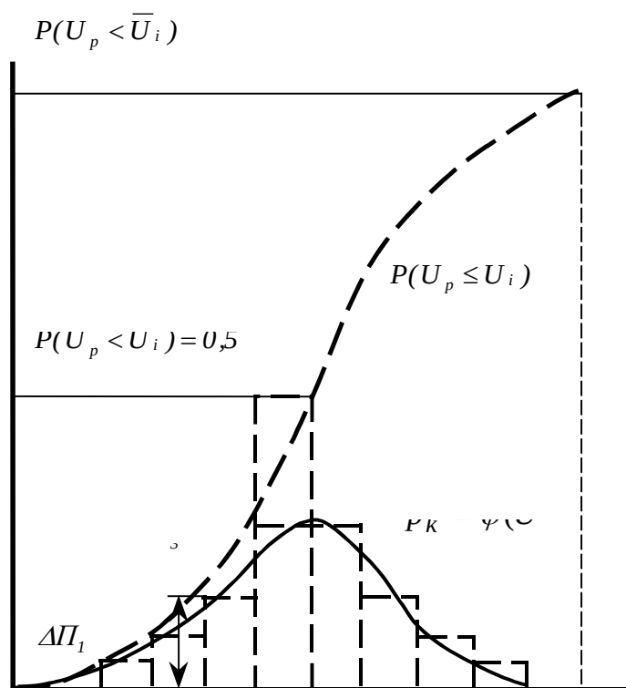
Рисунок 3.1 – Построение экспериментальных гистограмм распределения вероятности пробоев и аппроксимирующих кривых дифференциального и интегрального распределений
