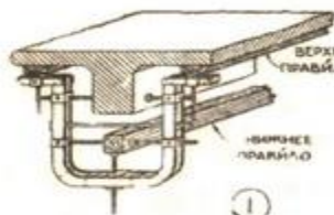
РЕЙКОДЕРЖАТЕЛЬ ДЛЯ ТЯГИ ПО БАЛКАМ
