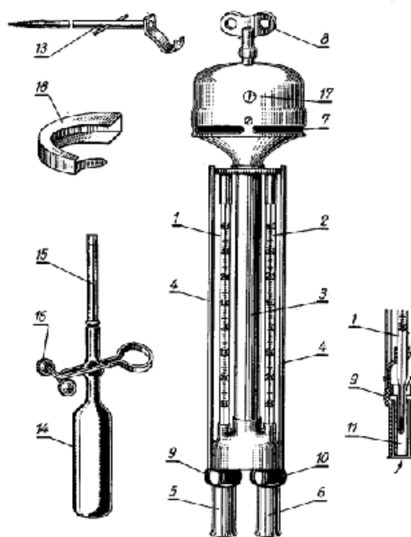
Рисунок 1.2 — Аспирационный психрометр Ассмана: а — общий вид; б — разрез; 1, 2 — ртутные метеорологические термометры («сухой» и «влажный»); 3 — корпус; 4 — планки корпуса; 5, 6 — защитные патрубки; 7 — аспиратор; 8 — механический ключ; 9, 10 — пластмассовые кольца, защищающие от передачи тепла от корпуса к термометрам; 11, 12 — внутренние трубки, в которых помещаются резервуары термометров; 13 — железный крюк — подвес; 14 — резиновая груша для смачивания батиста; 15 — стеклянная пипетка; 16 — зажим; 17 — винт; 18 — кольцо.
