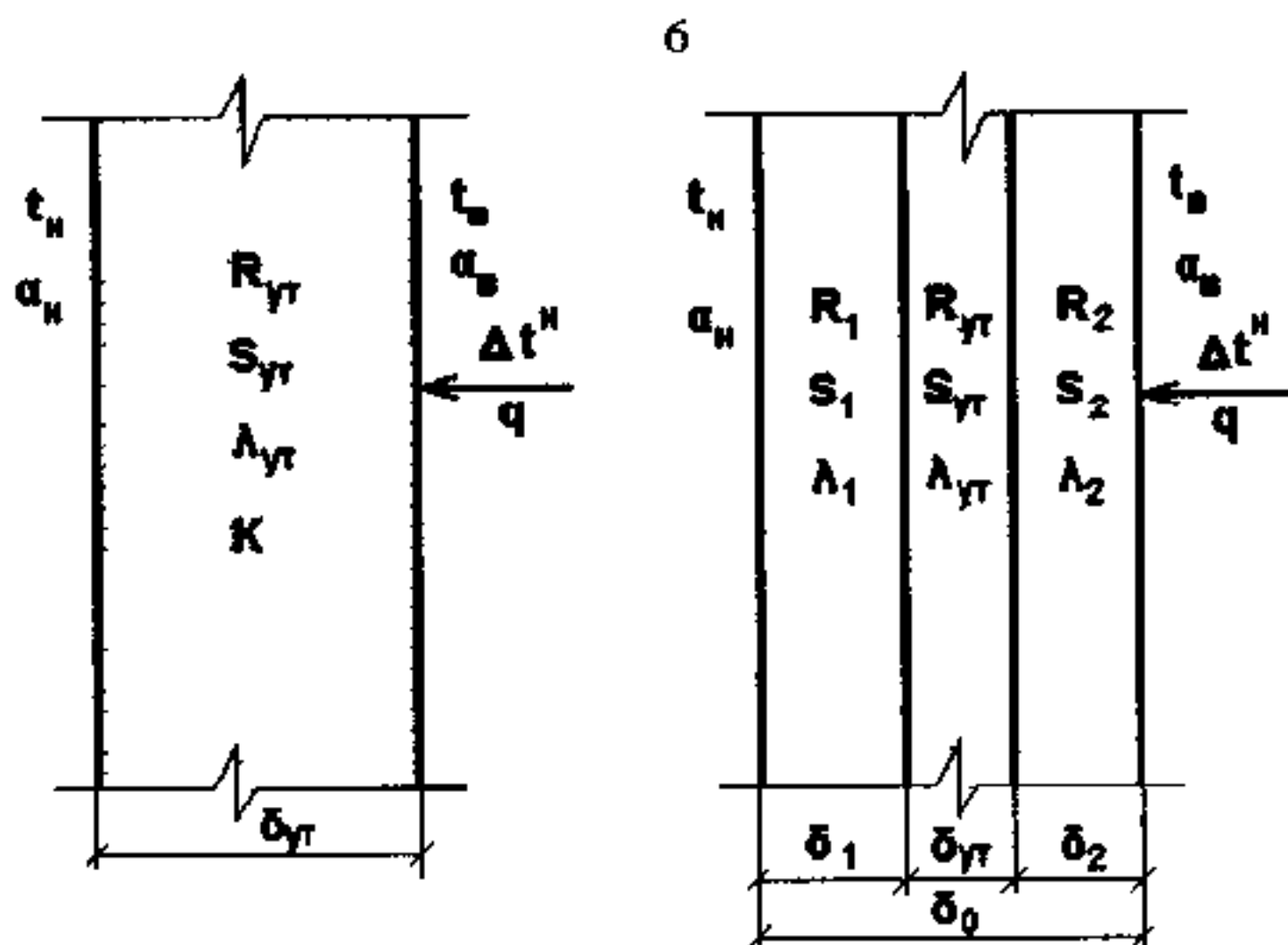
Рис.1 Ограждающая конструкция а)- однослойная; б) - многослойная
