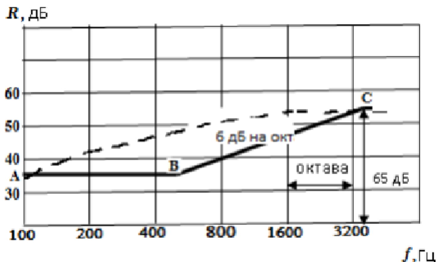
Рисунок 2 - Нормативная и расчетная характеристики звукоизоляции
