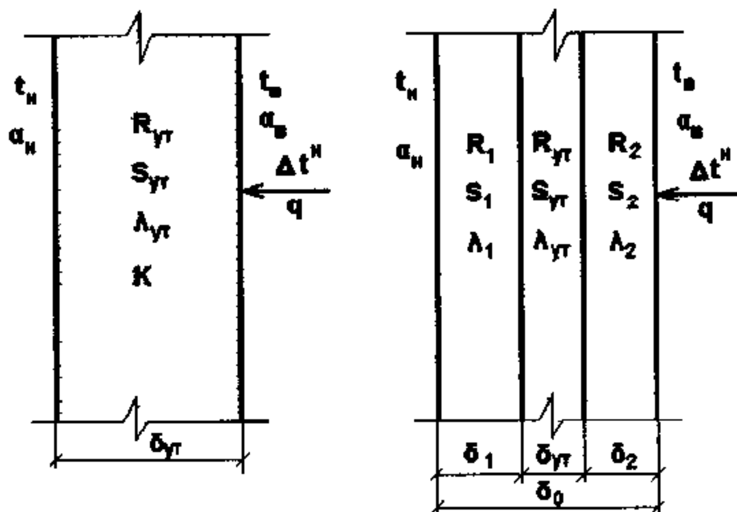
Рис.1 Ограждающая конструкция а)- однослойная; б) - многослойная
