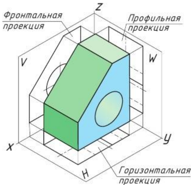
Рис. 49. Комплексный чертеж
