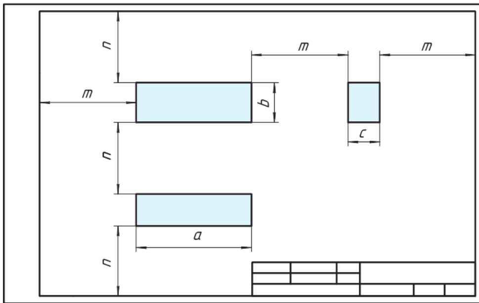
Рис. 22. Компоновка чертежа
