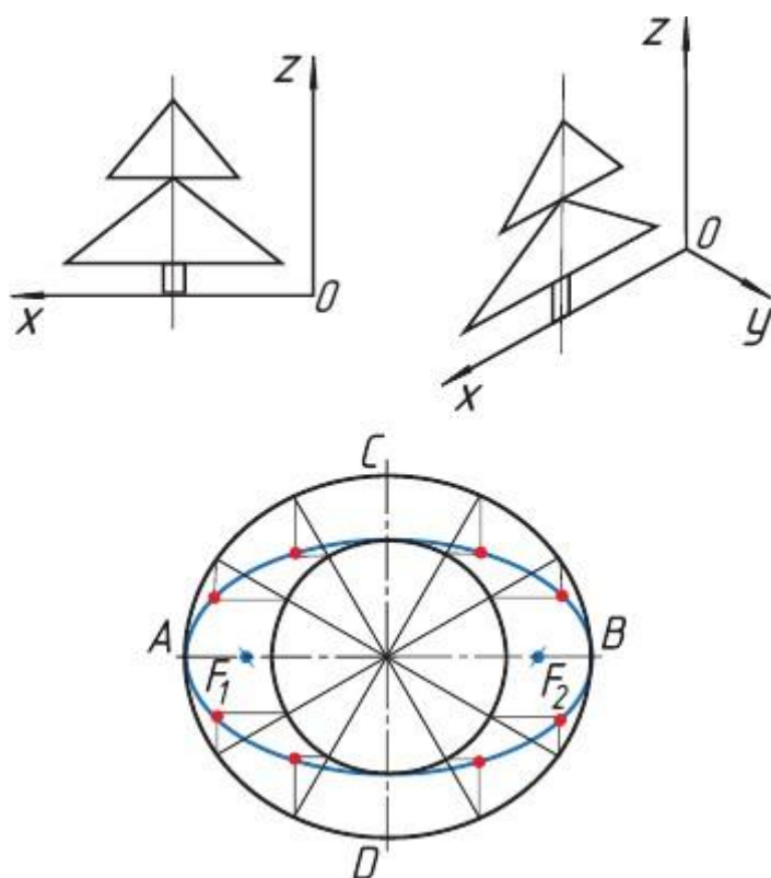
Рис. 55. Эллипс
