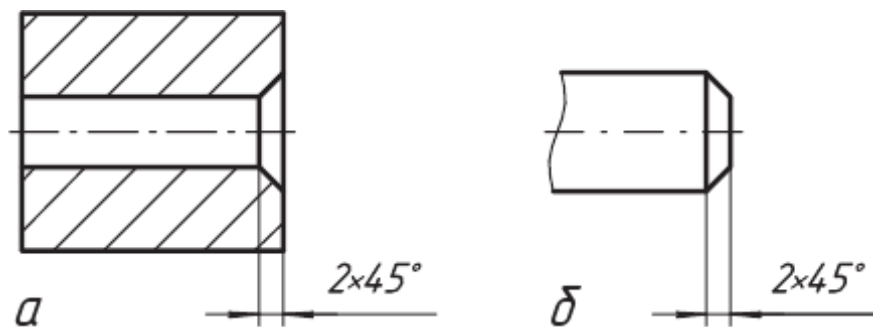
Рис. 31. Обозначение фаски
