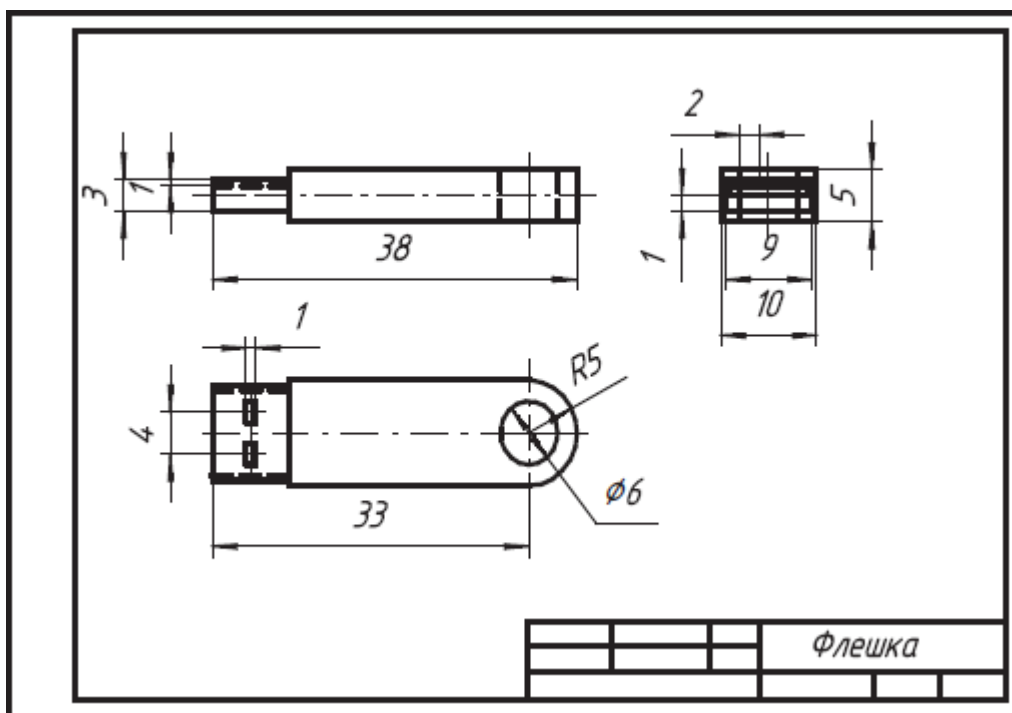
Рис. 5. Чертеж детали (пример)
