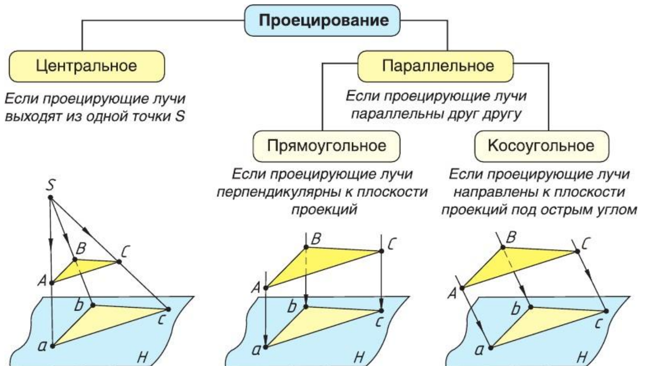
Рис. 40. Виды проецирования
