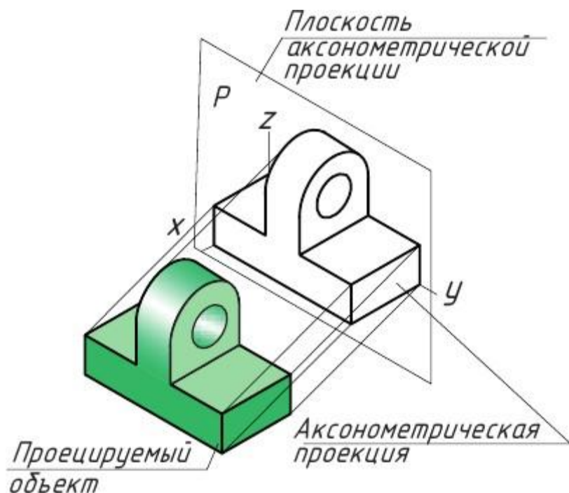
Рис. 54. Аксонометрическая проекция
