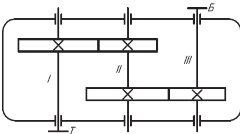
Рис. 8. Схема (пример)
