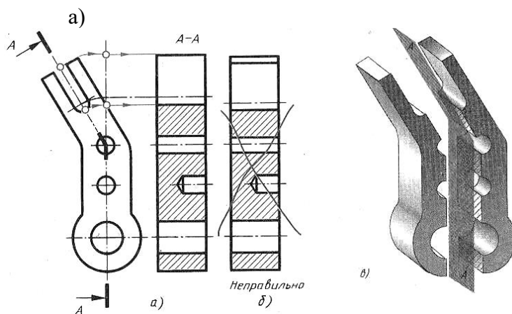
Рисунок 12.2. Сложный разрез (ломаный)
