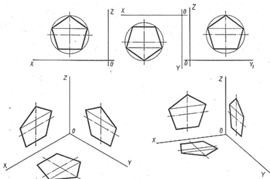
Рис.5.4. Пример выполнения задания
