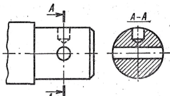
Рис.10.3 Сечение по типу разреза
