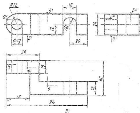
б) Эскиз детали.
