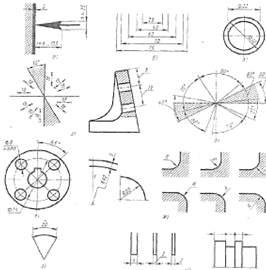
Рисунок 2.3. Правила нанесения размеров
