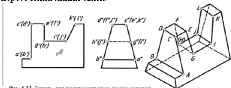
Рис. 4.32. Деталь, для построения вида сверху которой необходимо найти проекции точек
