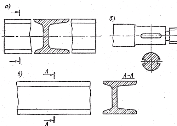
Рис.10.1. Расположение вынесенных сечений
