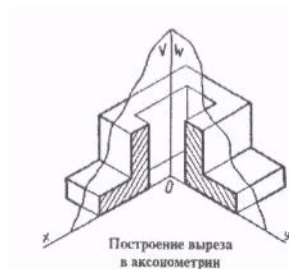
Рисунок 11.5. Построение выреза в аксонометрии.
