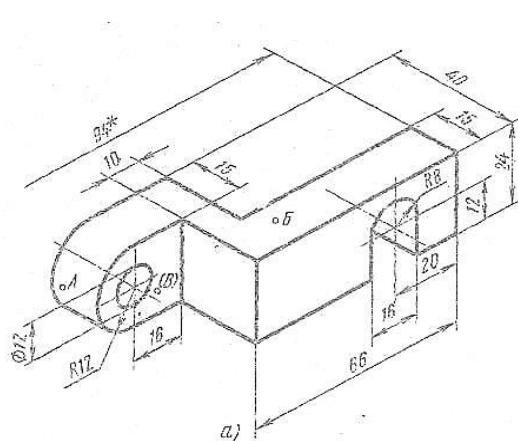
а) Аксонометрия детали
