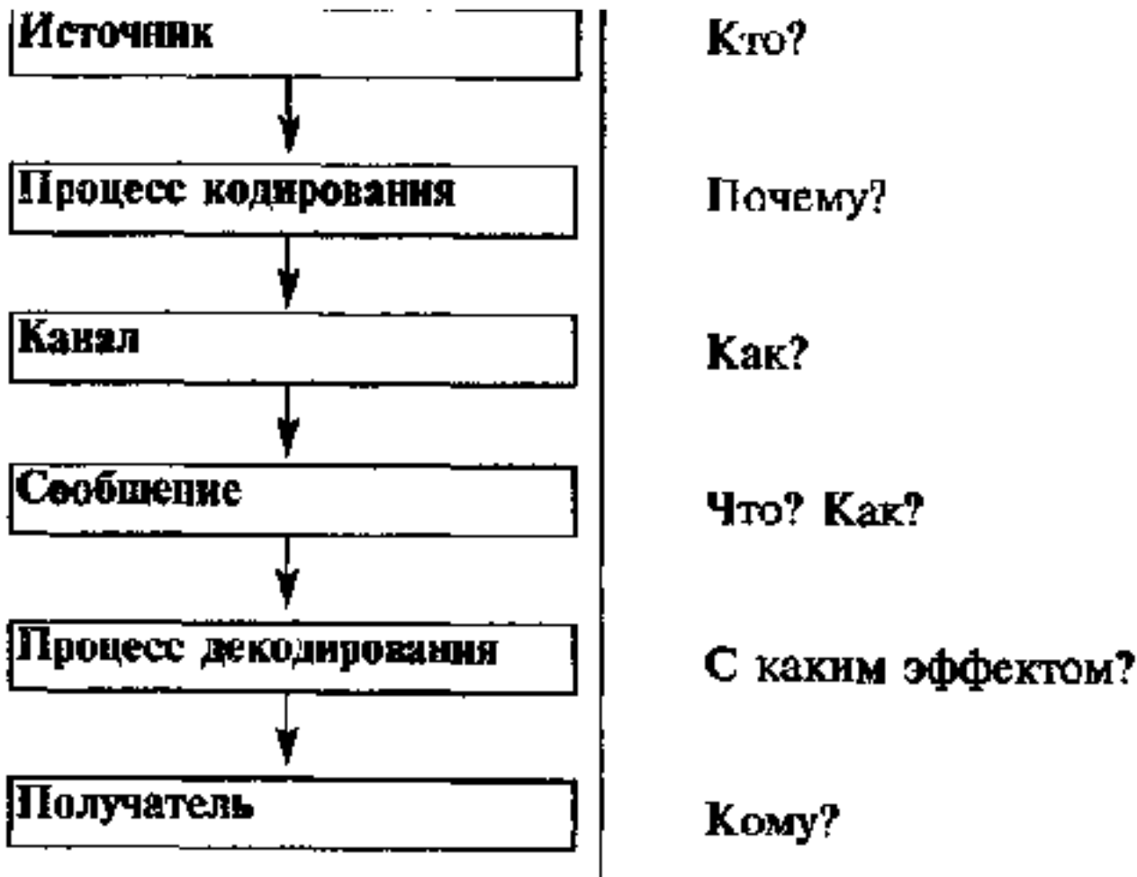
Рис.2.3 Модель контент-анализа
