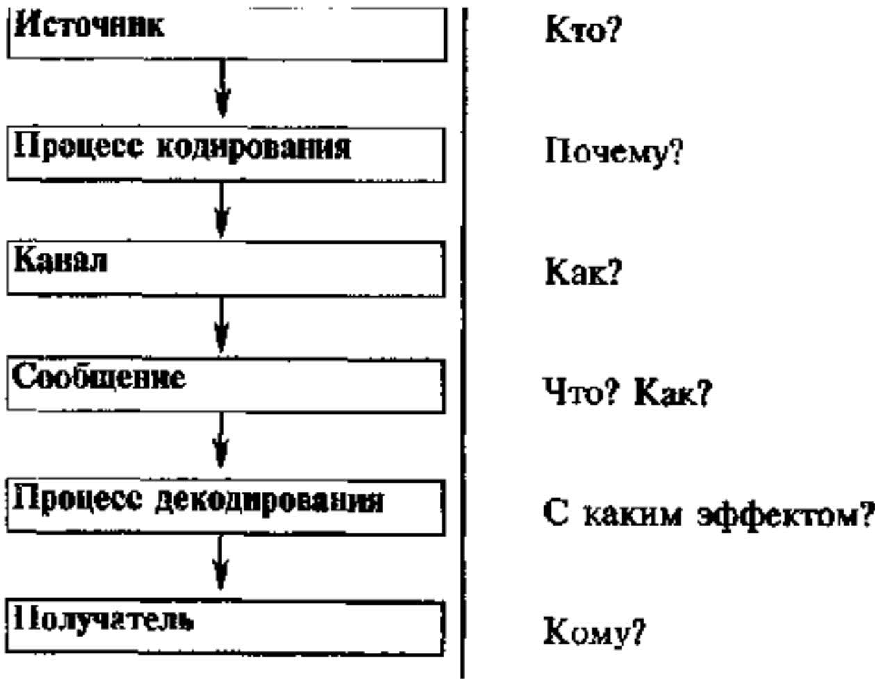
Рис.2.3 Модель контент-анализа
