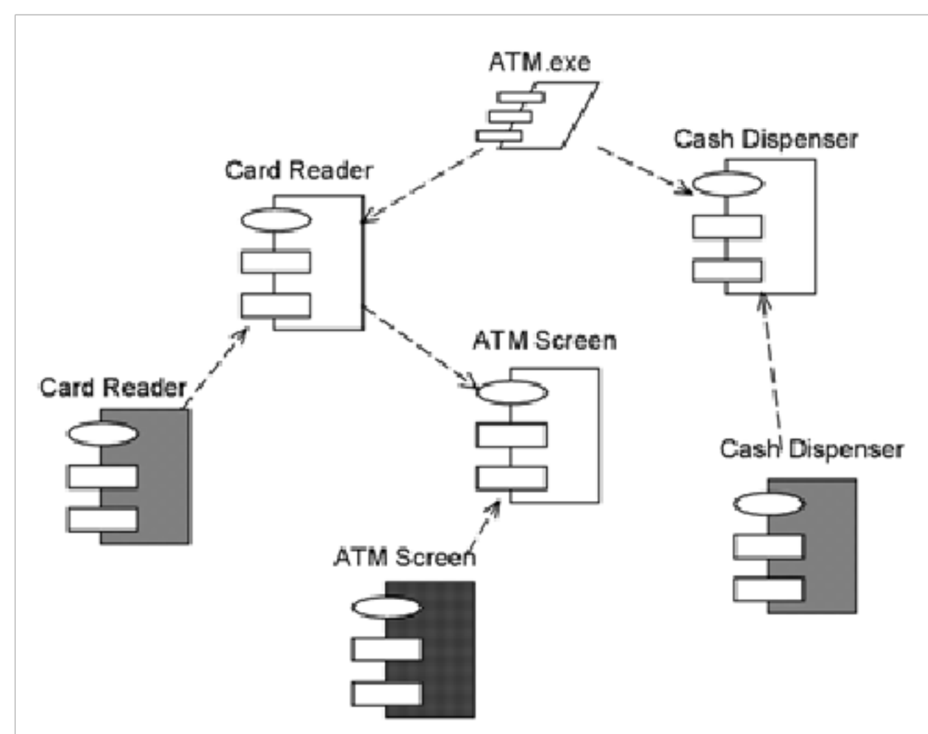
Рисунок 3.20 -. Пример диаграммы компонентов
