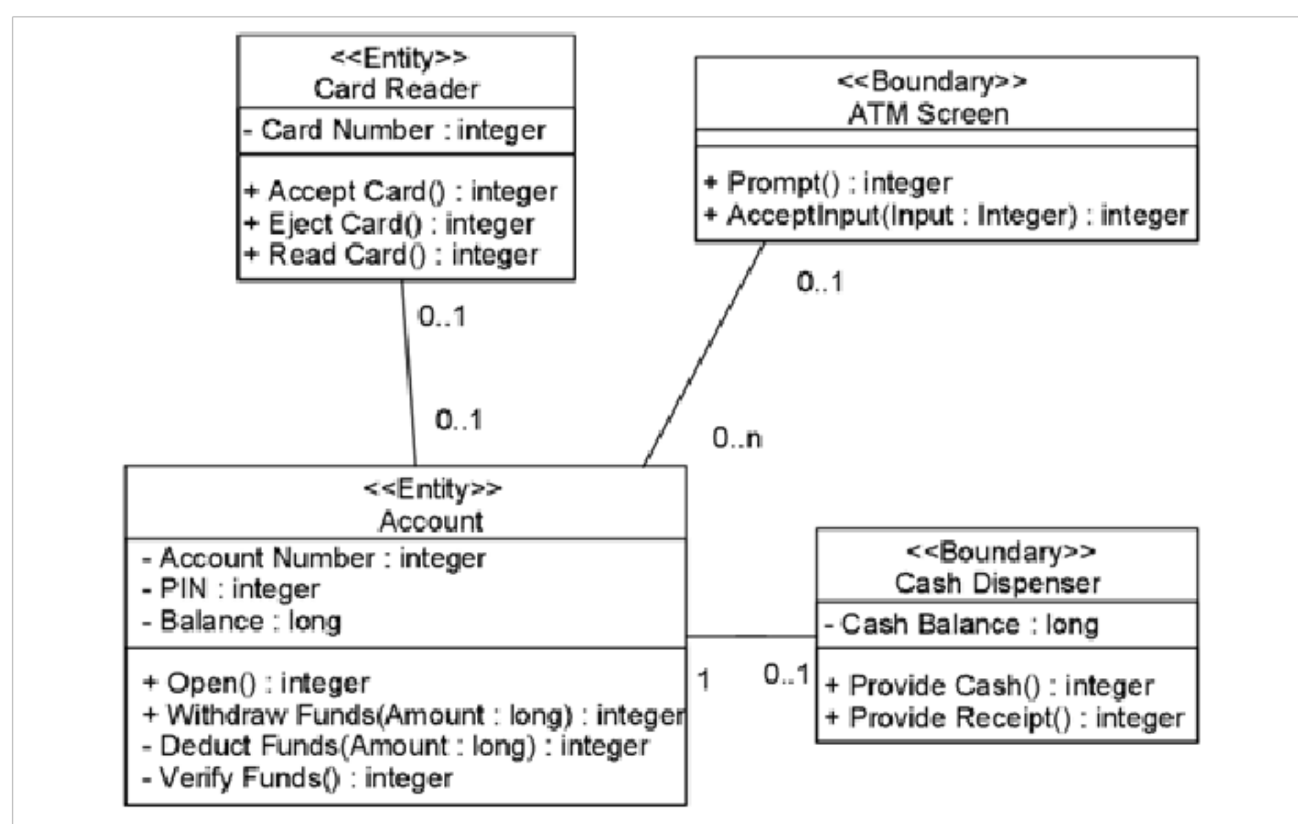
Рисунок 3.9 - Пример диаграммы классов
