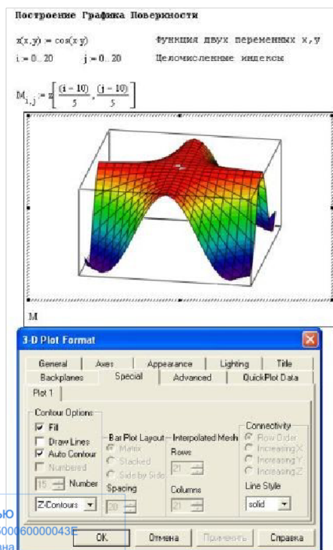
Рисунок 5.2 - Построение графика поверхности в системе Mathcad
