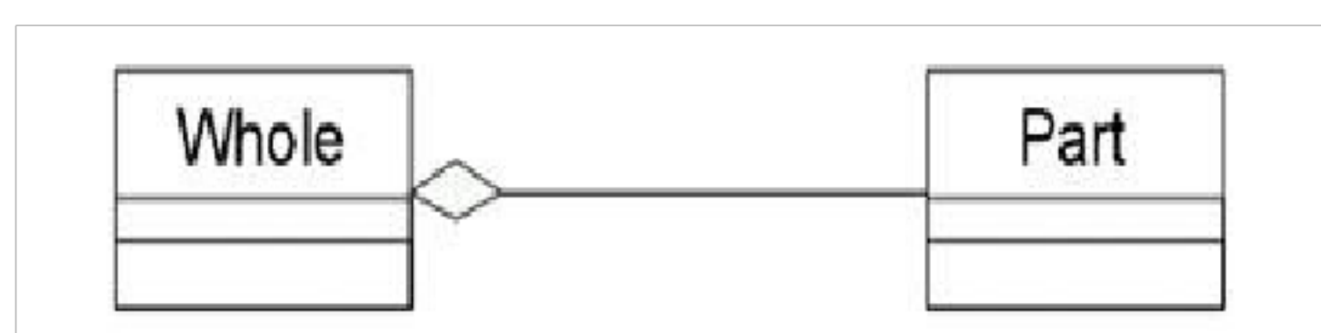
Рисунок 3.12 - Связь агрегация
