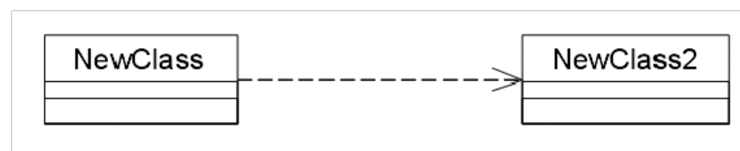
Рисунок 3.11 - Связь зависимость
