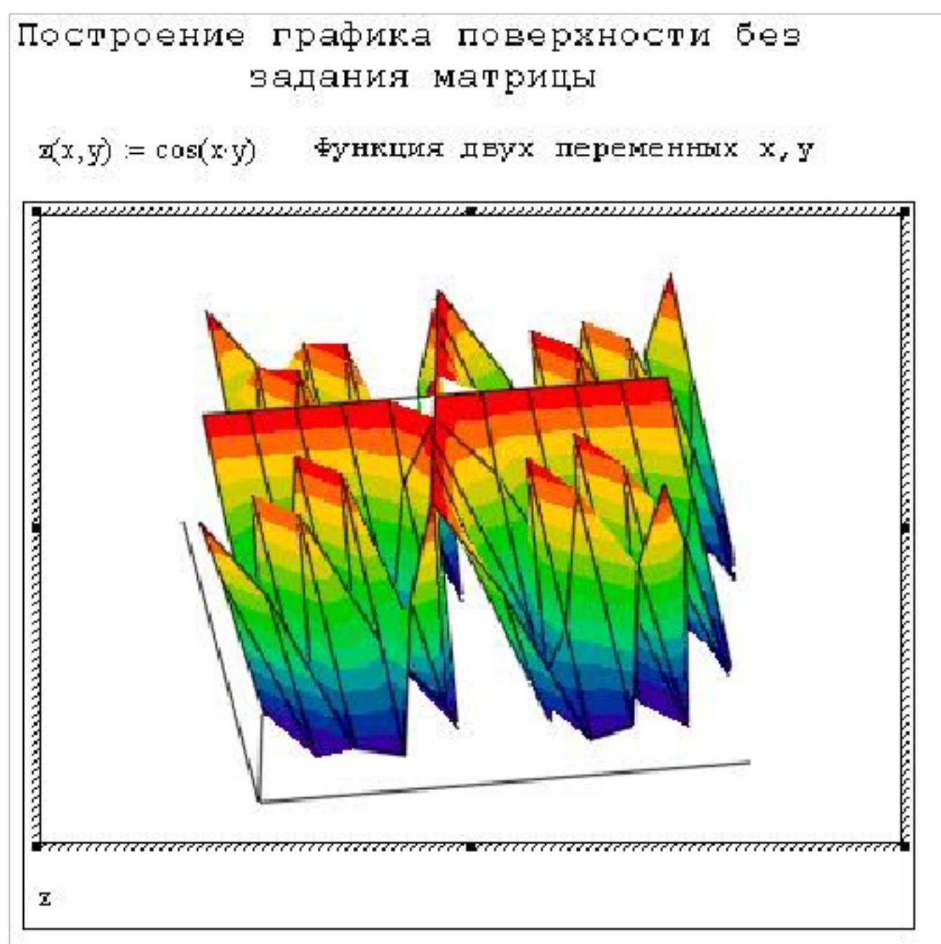
Рисунок 6.1 - Построение графика поверхности без задания матрицы
