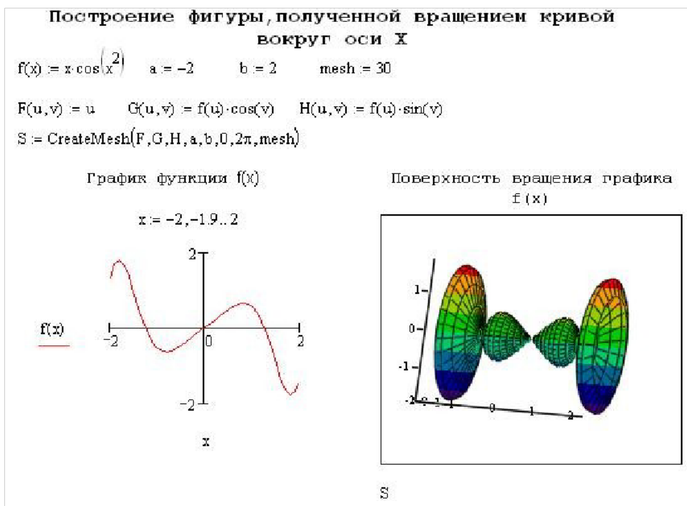
Рисунок 6.3 – Фигура, полученная вращением кривой.
