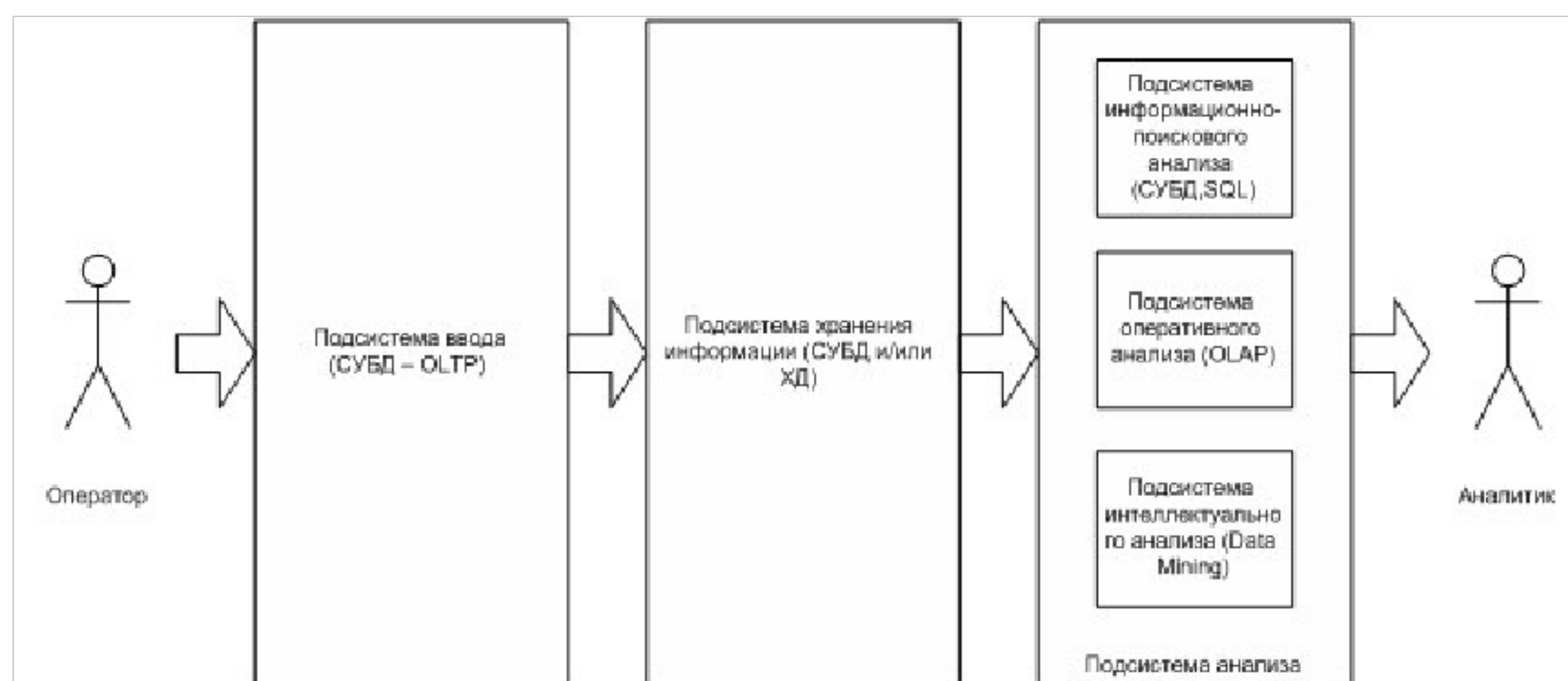
Рисунок 1.11 - Архитектура СППР
