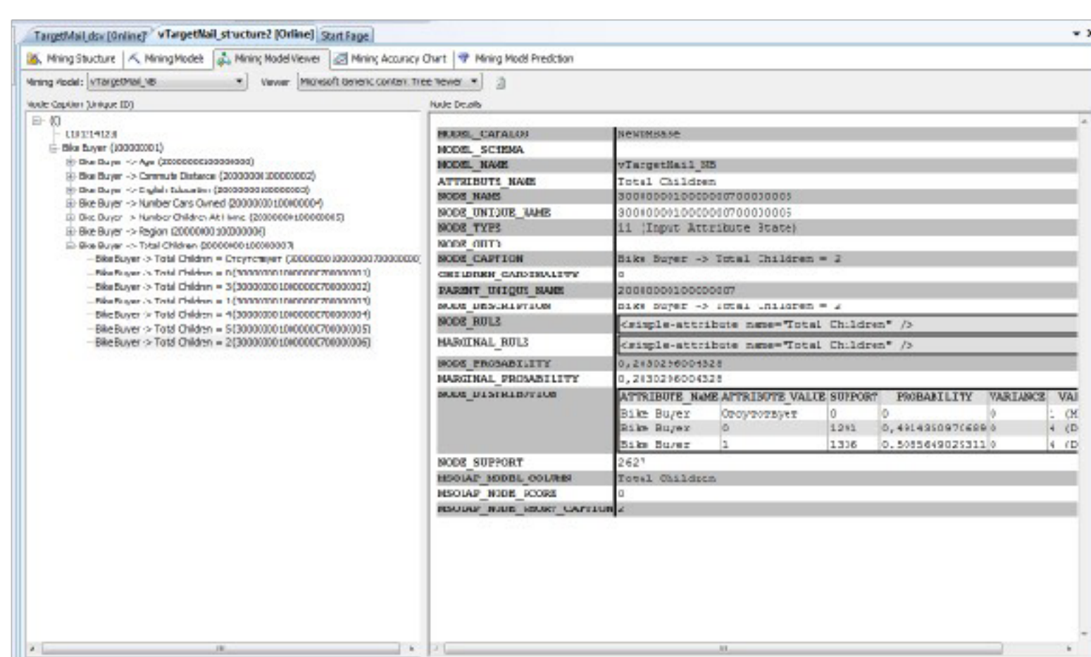
Рисунок 1.1. - Просмотр модели на базе упрощенного алгоритма Байеса средствами BIDEVStudio
