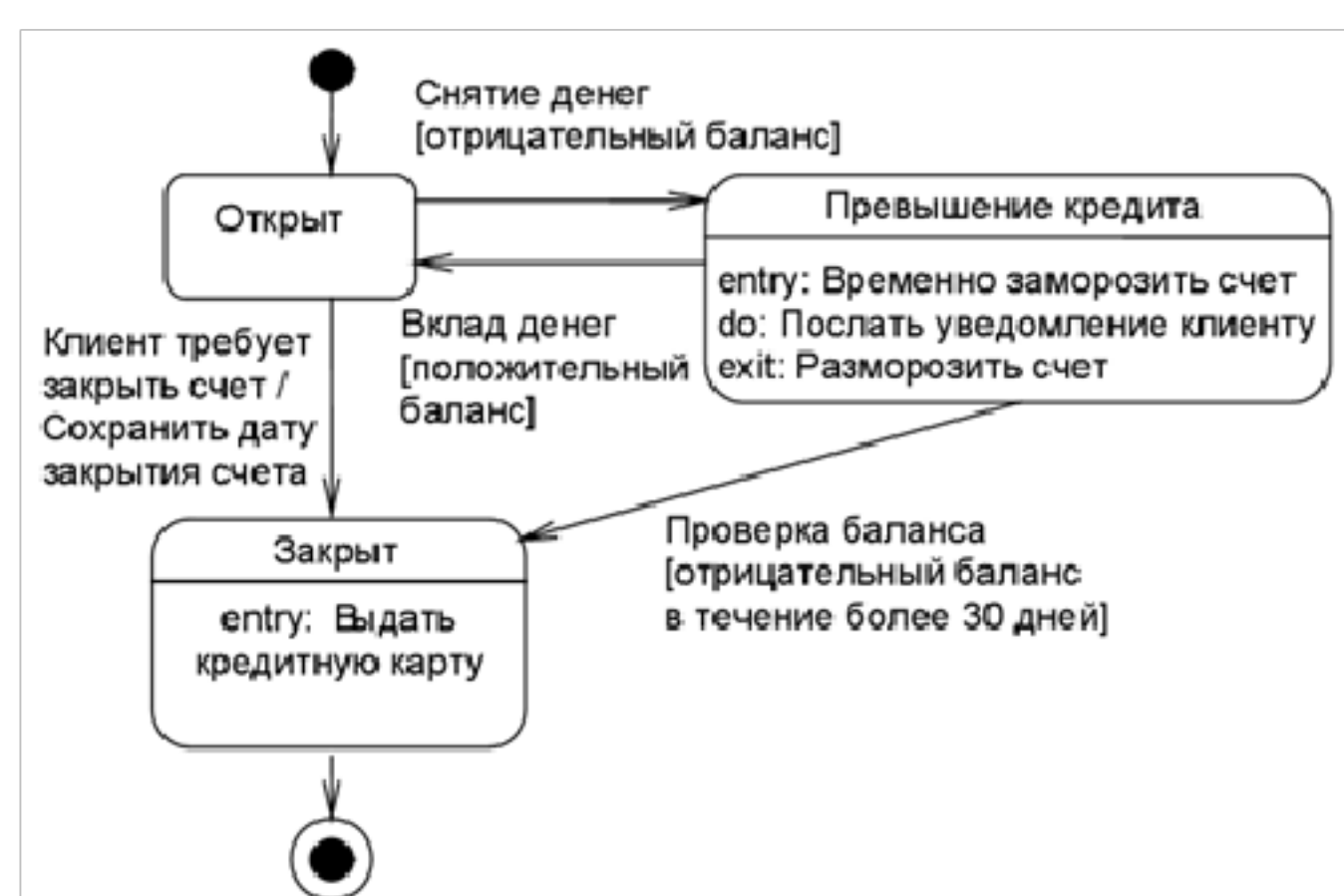
Рисунок 3.18 - Пример диаграммы состояний
