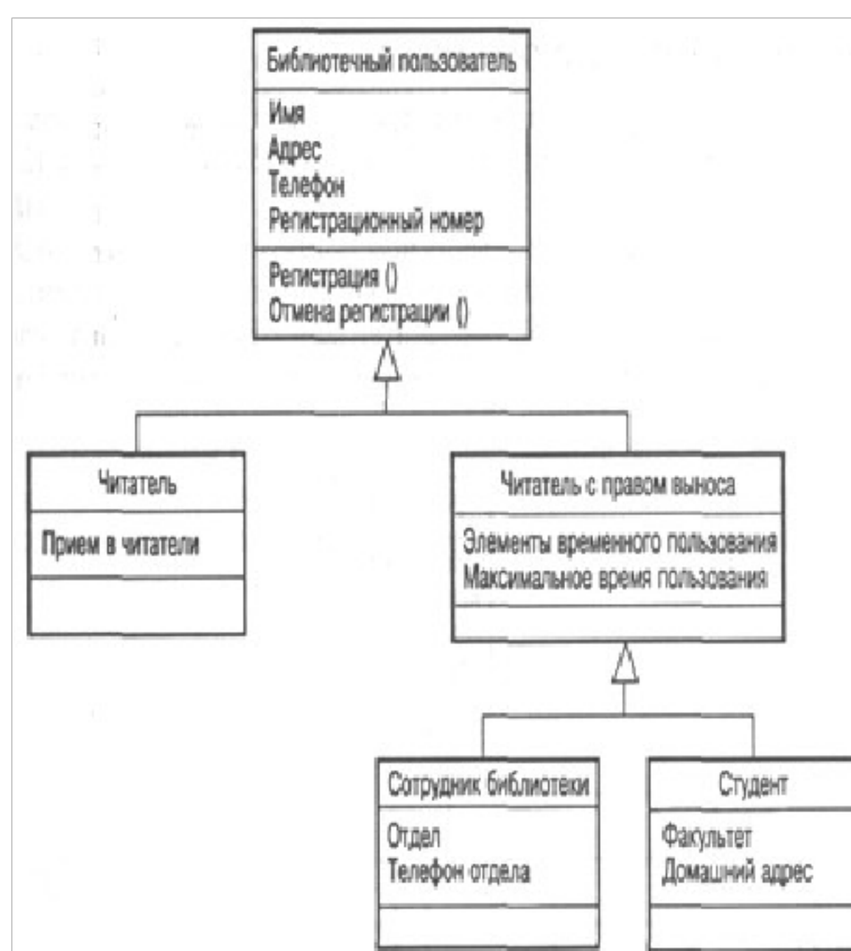
Рисунок 3.13 - Пример связи наследование
