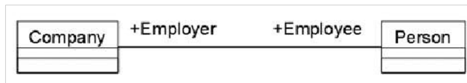
Рисунок 3.15 - Пример ролей связей
