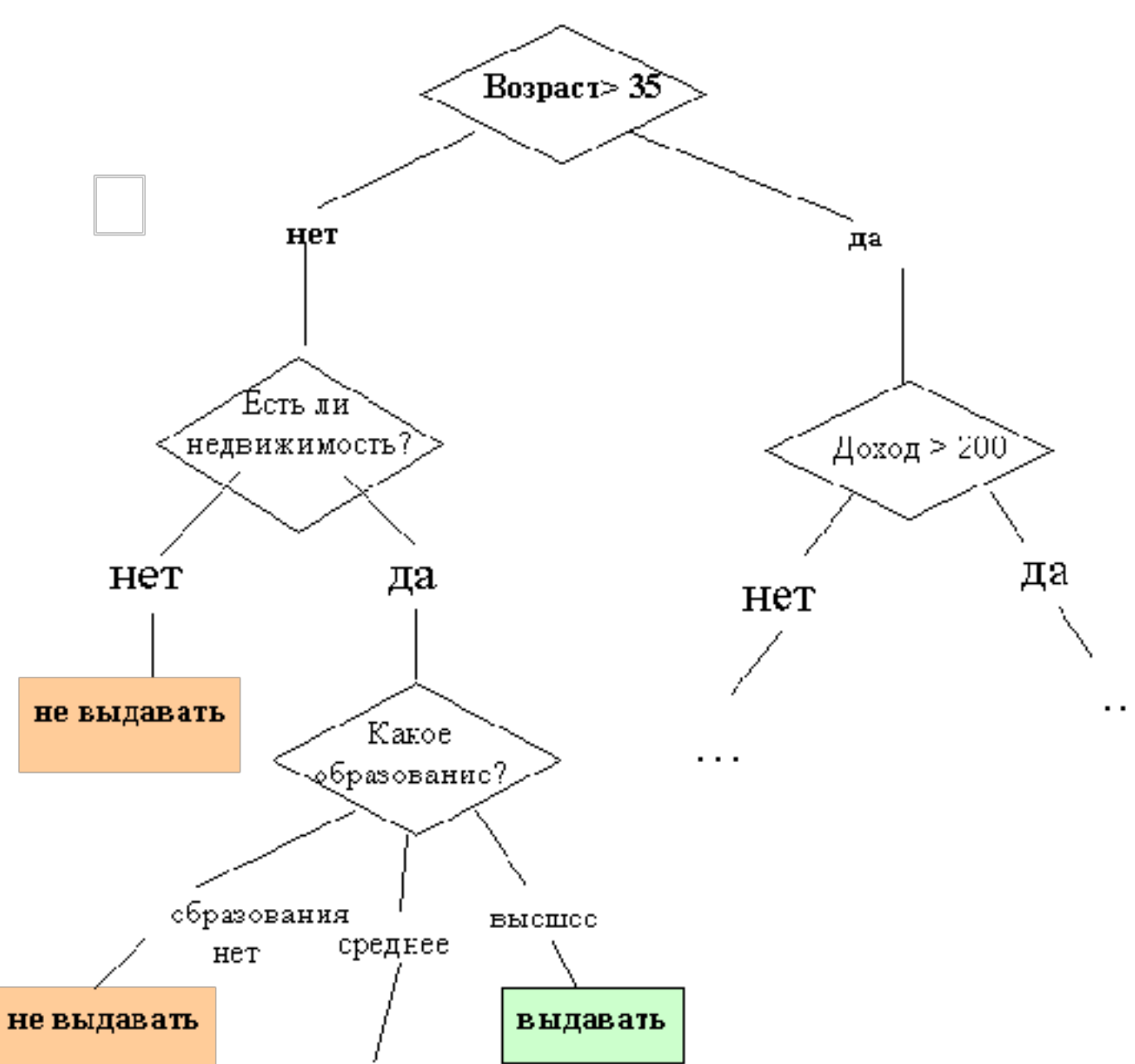
Рис. 9.2. Дерево решений "Выдавать ли кредит?"
