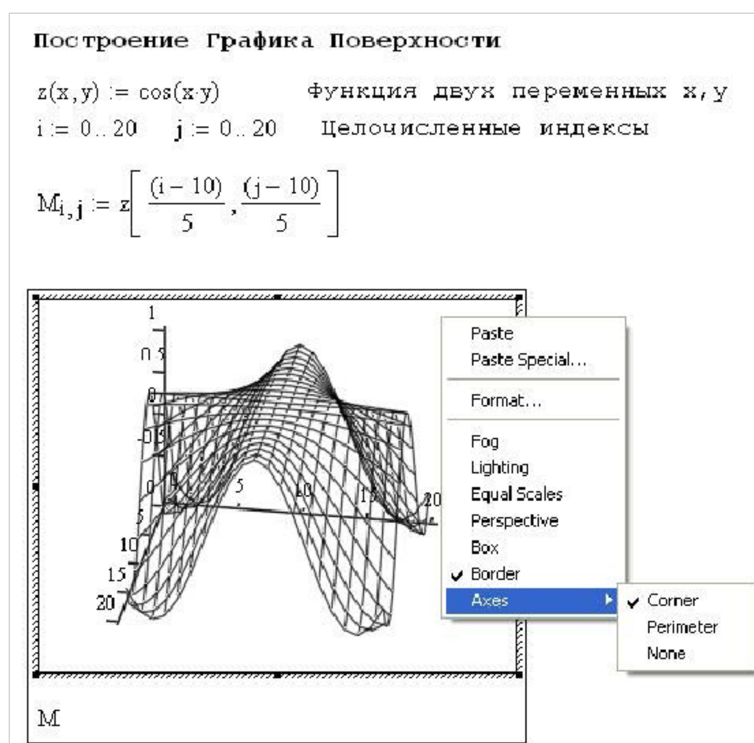
Рисунок 5.1 - Построение поверхности без удаления невидимых линий
