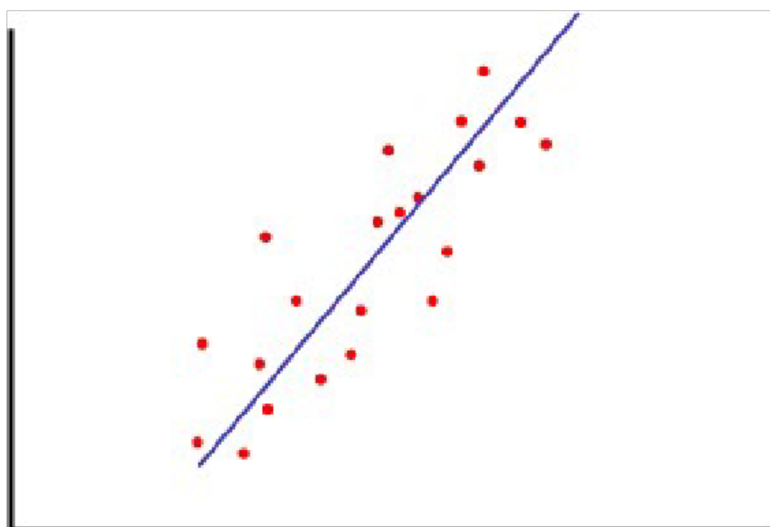
Рисунок 1.5. Пример использования линейной регрессии
