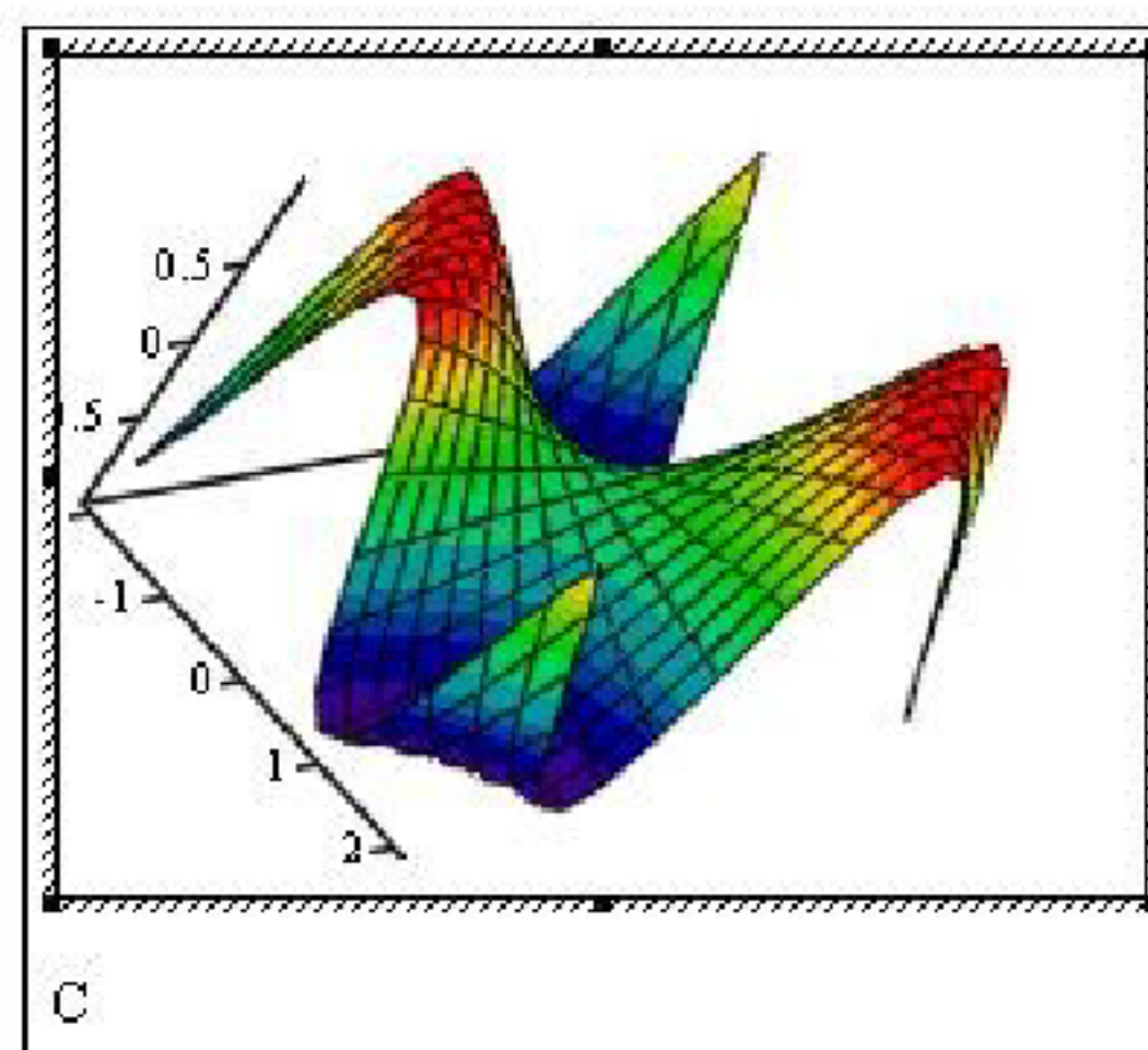
Рисунок 6.2 - Построение графика поверхности с применением функции CreateMesh
