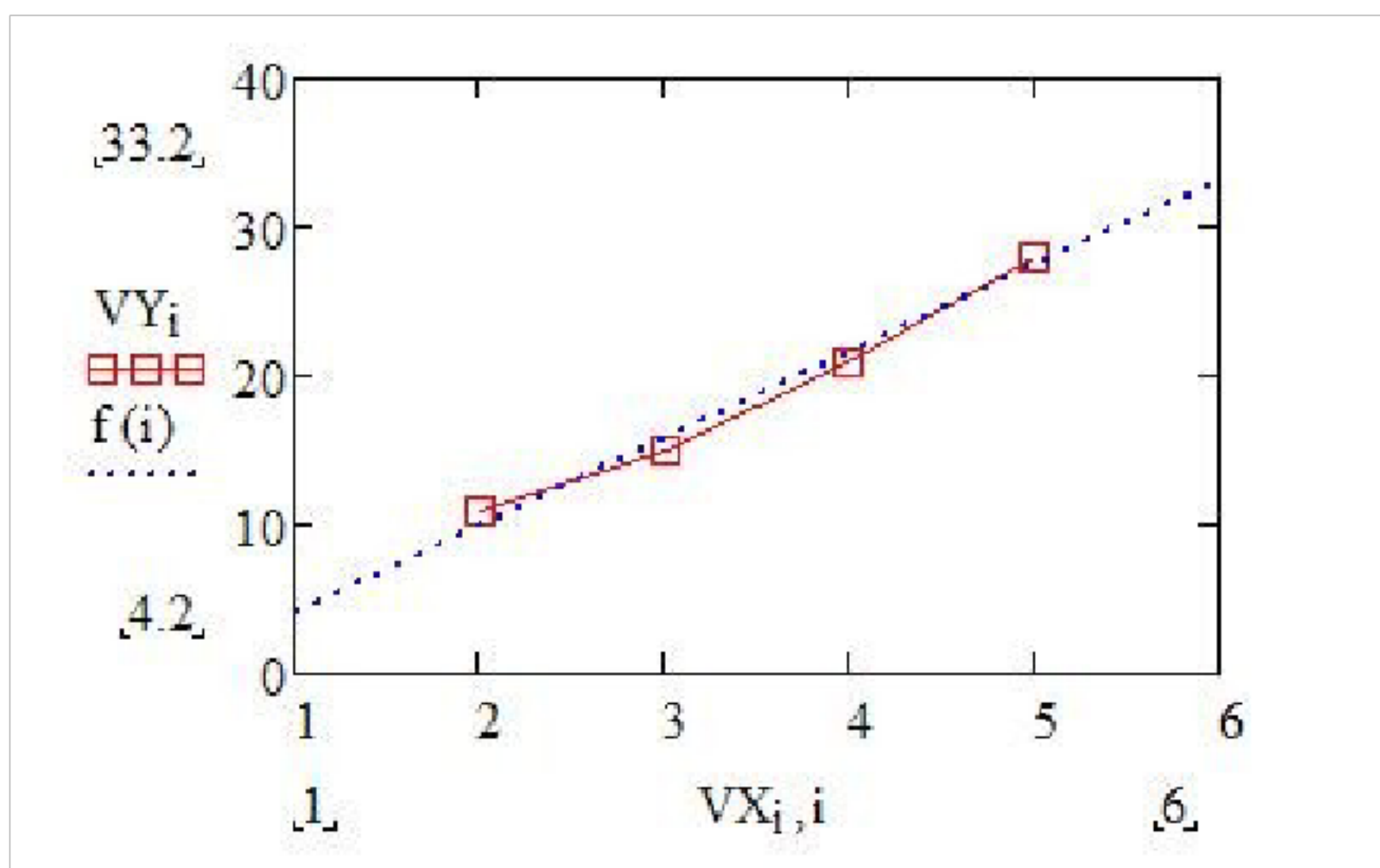
Рисунок 4.2 - Линейная регрессия
