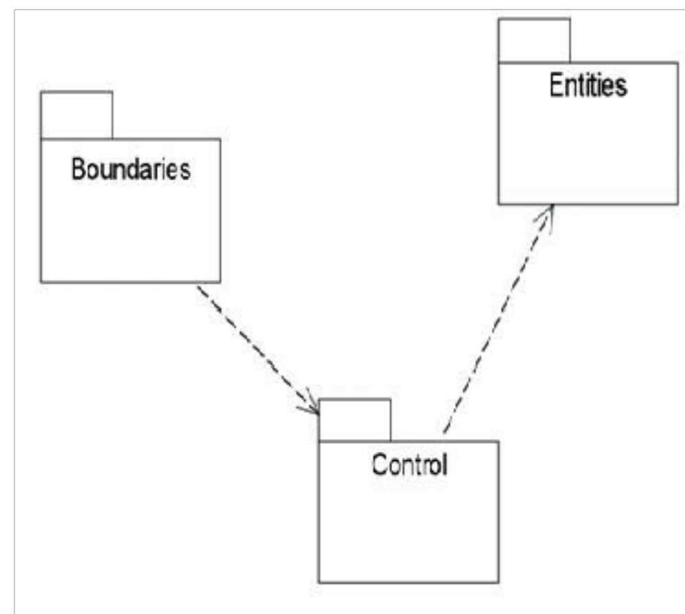
Рисунок 3.17 - Пример диаграммы пакетов
