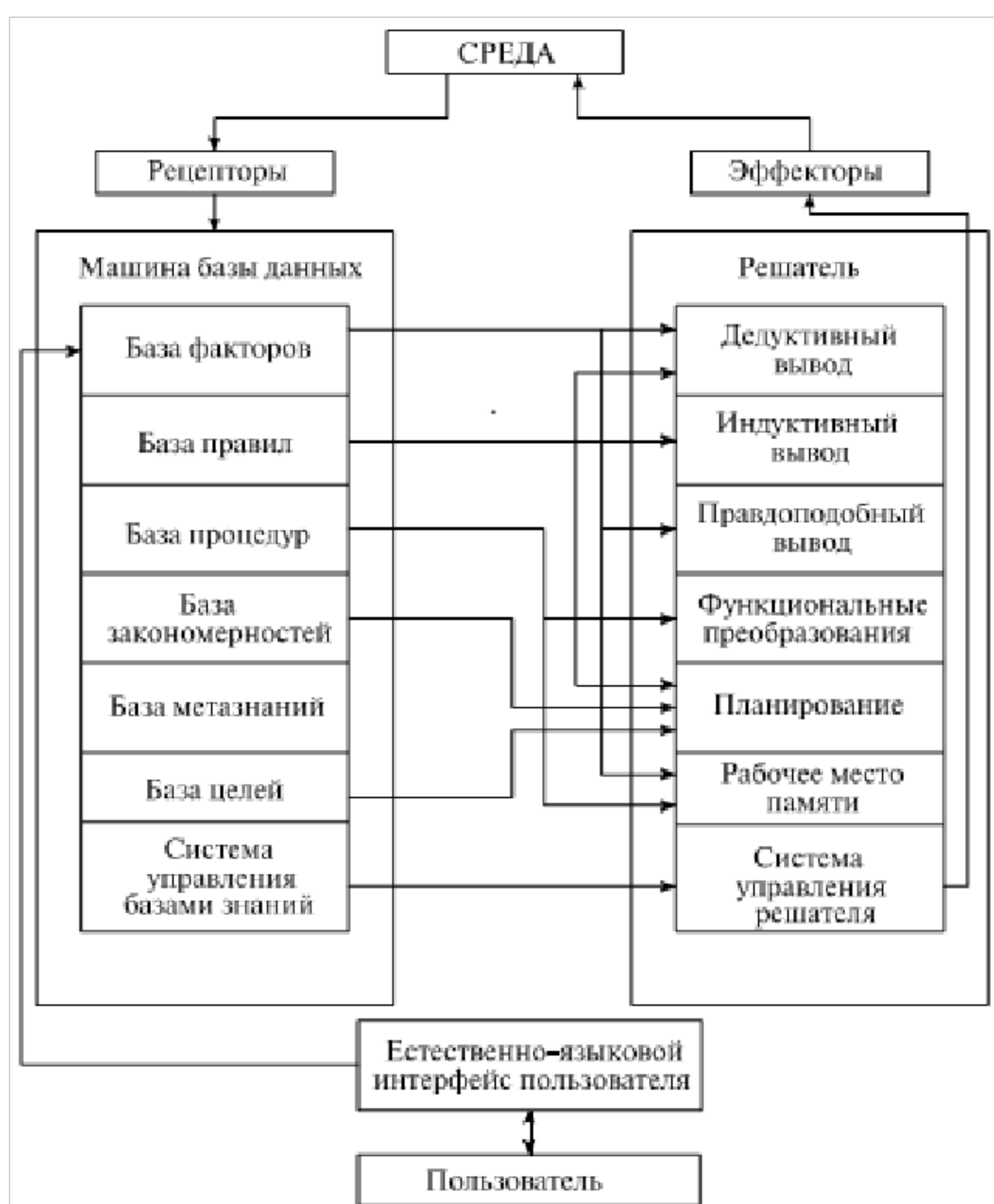
Рисунок 1.15. Общая структура интеллектуальной системы
