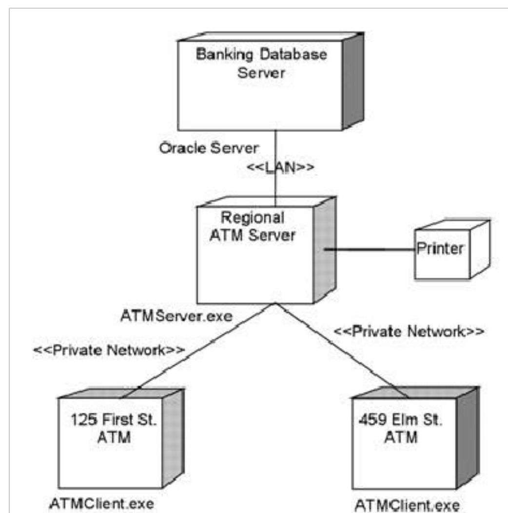
Рисунок 3.19 - Пример диаграммы размещения
