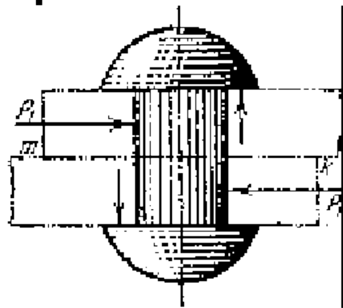
Рис.3. Расчетная модель действия нормальных напряжений
