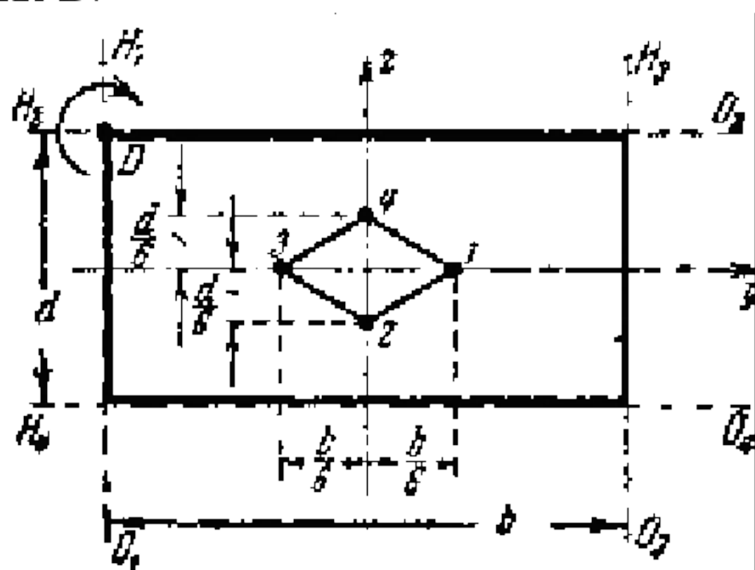
Рис.4. построение ядра для прямоугольного сечения.
