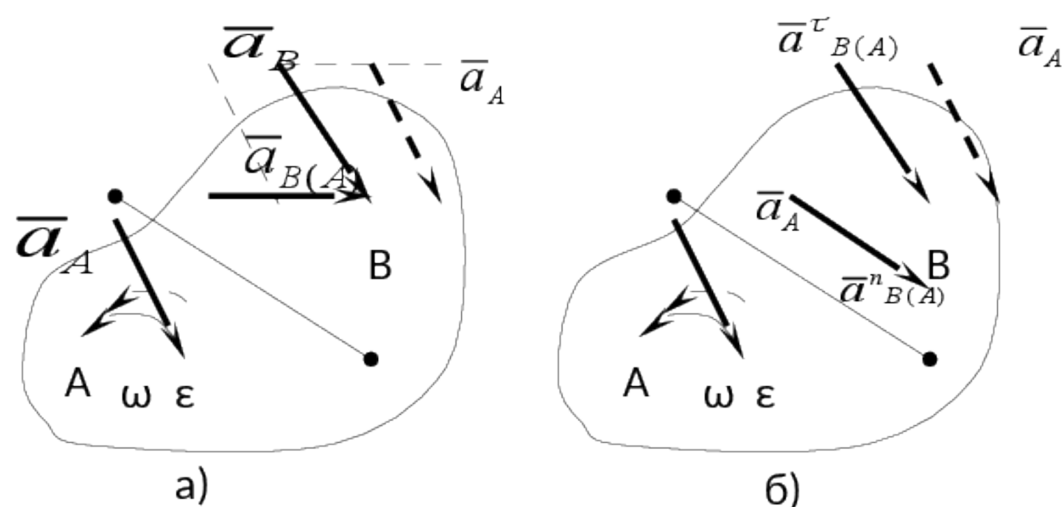
Рисунок 10. Определение ускорений точек плоской фигуры.
