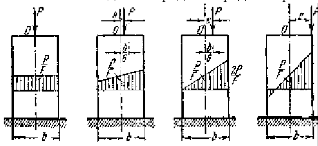
Рис.5. Динамика изменения напряжений при изменении эксцентриситета.
