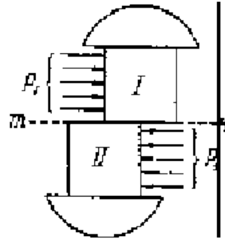
Рис.2. Силы, действующие на заклепочное соединение.
