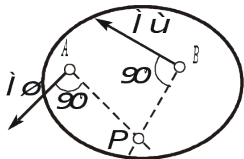
Рис. 2.28. Основной случай определения положения М.Ц.С.
