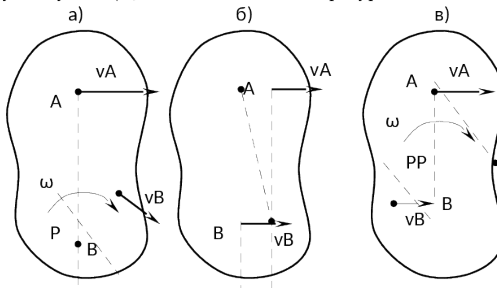
Рисунок 9. Нахождение мгновенного центра скоростей.
