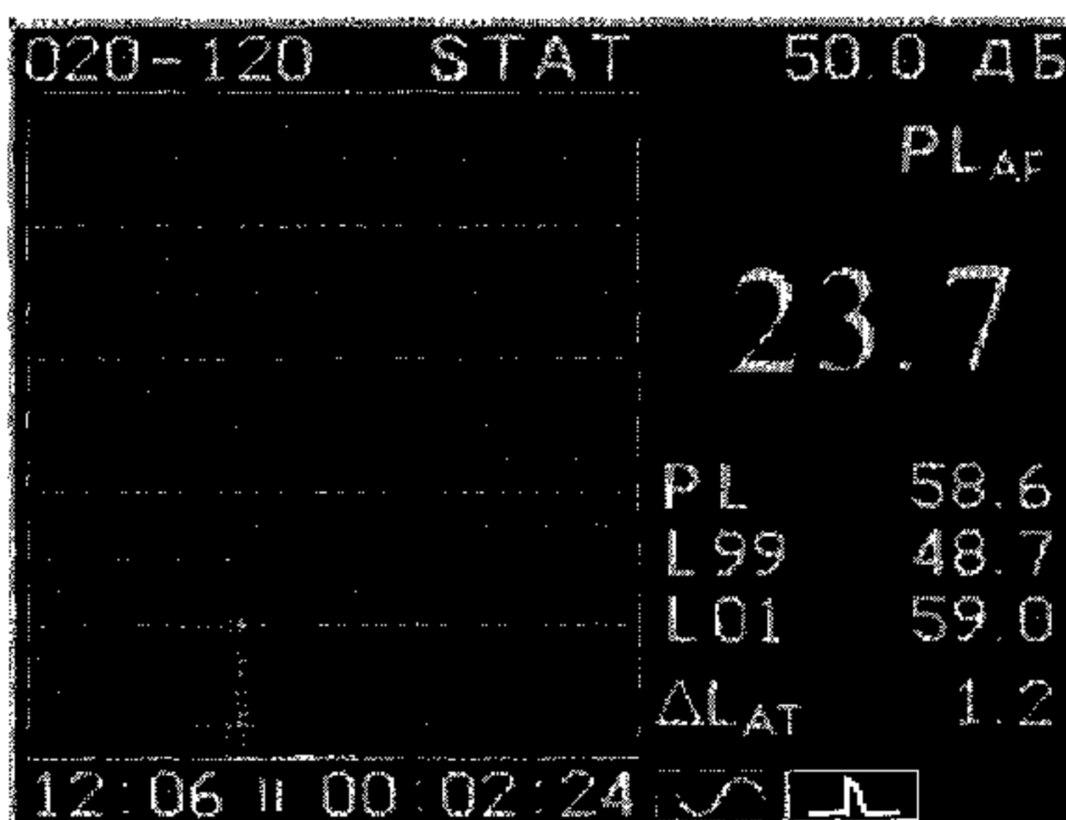
Рисунок 18 - Индикация в режиме STAT
