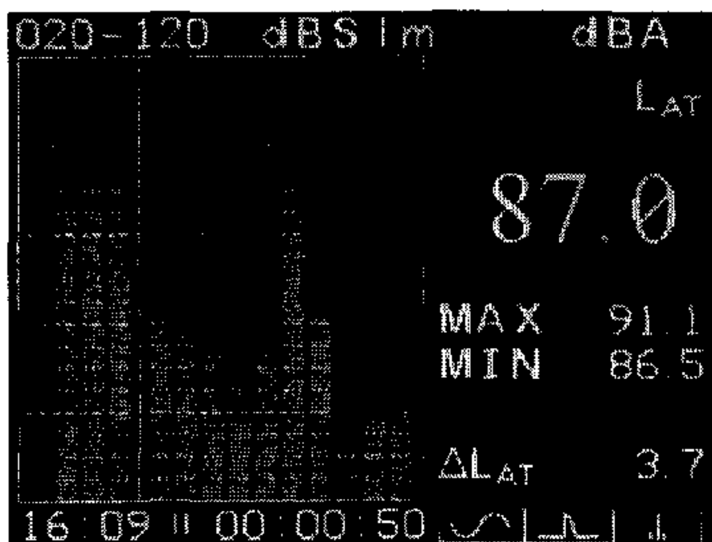
Рисунок 7 - Индикация в режиме dB SIm
