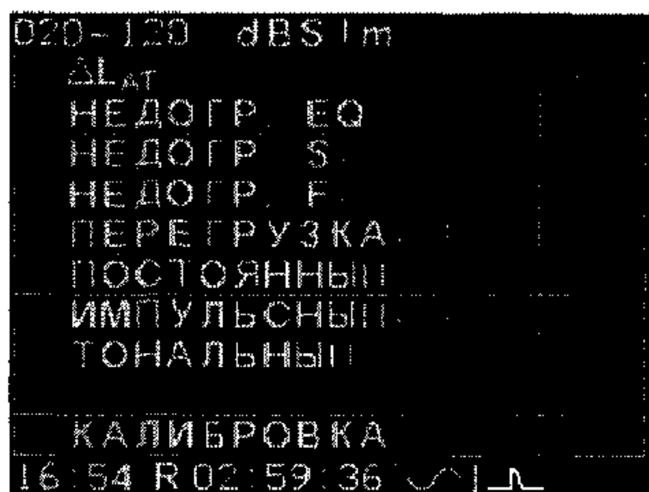
Рисунок 9 - варианты табличного представления результатов
