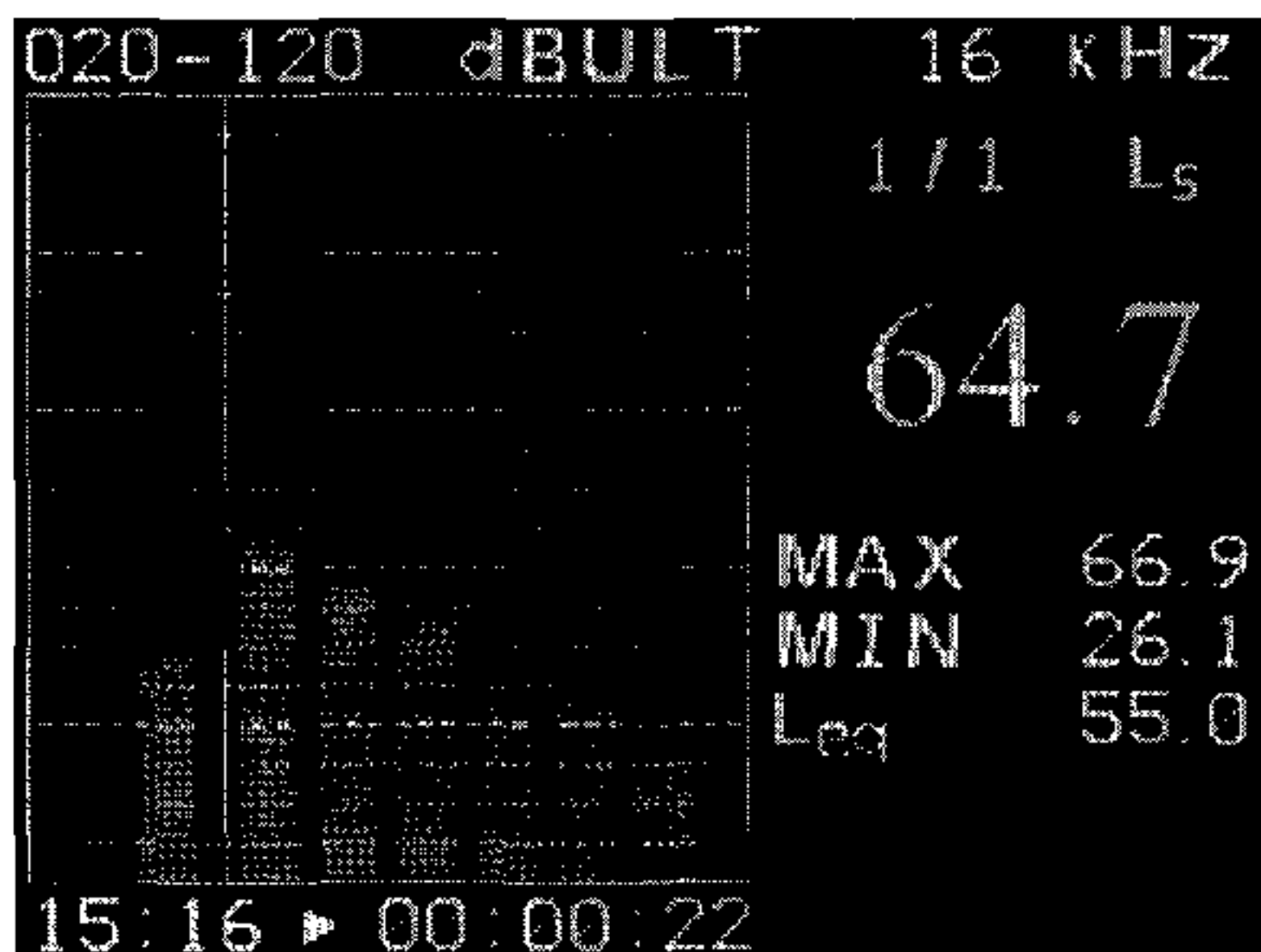
Рисунок 16 - индикация в режиме dBULT
