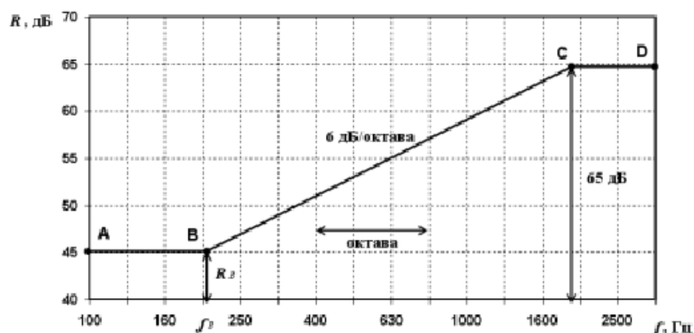
Рисунок 1 - Частотная характеристика звукоизоляции (шкала абсцисс – логарифмическая)
