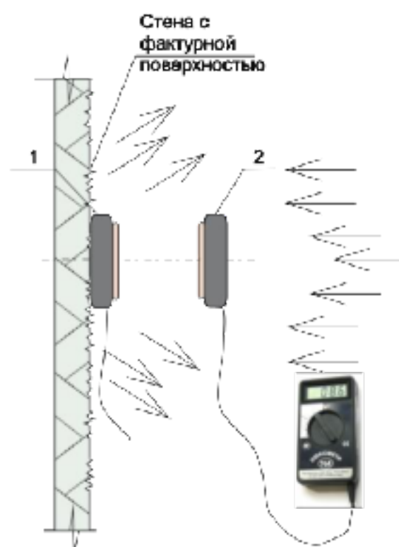
Рисунок 3.1 — Пример проведения замеров отраженного света люксометром (положения фотозлемента при измерении светотражения различных по фактуре поверхностей стен): 1 — измерение падающего на поверхность стены света; 2 — измерение света, отраженного от поверхности стены
