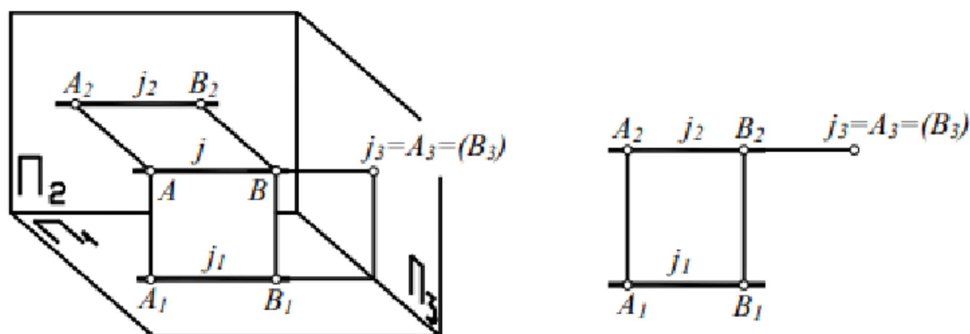
Рис.13. Профильно-проецирующая прямая
