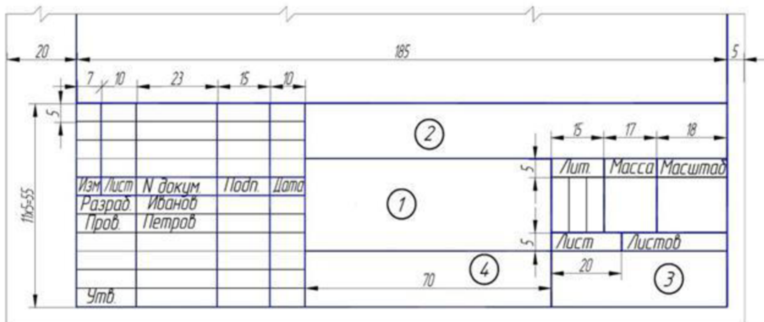
Рисунок 1 Основная надпись
