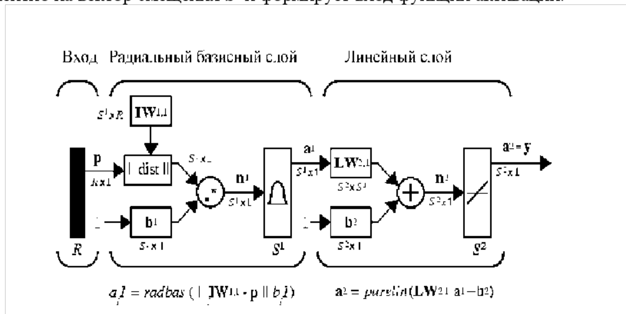
Рис. 3. Радиальная базисная сеть
