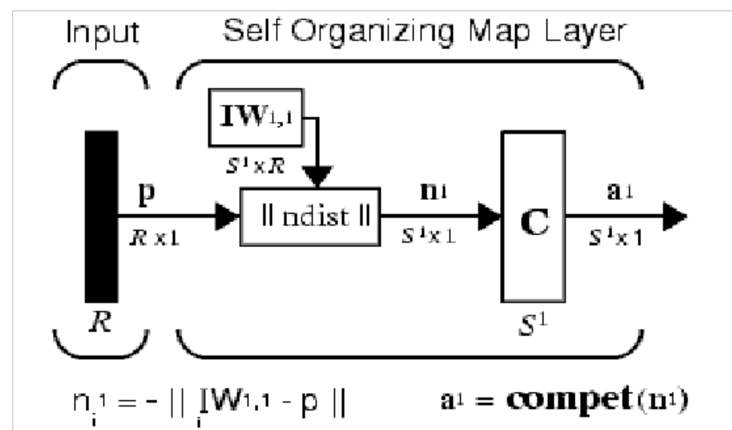
Рис. 12.2. Архитектура карты Кохонена
