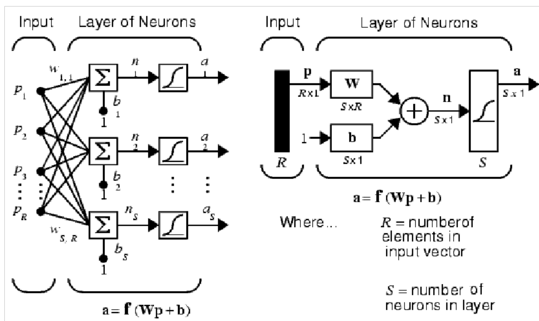
Рис. 7.5. Однослойная сеть с прямой передачей сигнала
