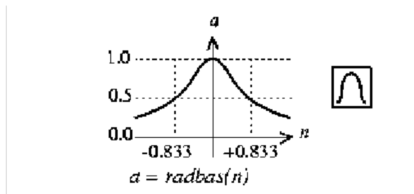
Рис. 2. График функции активации
