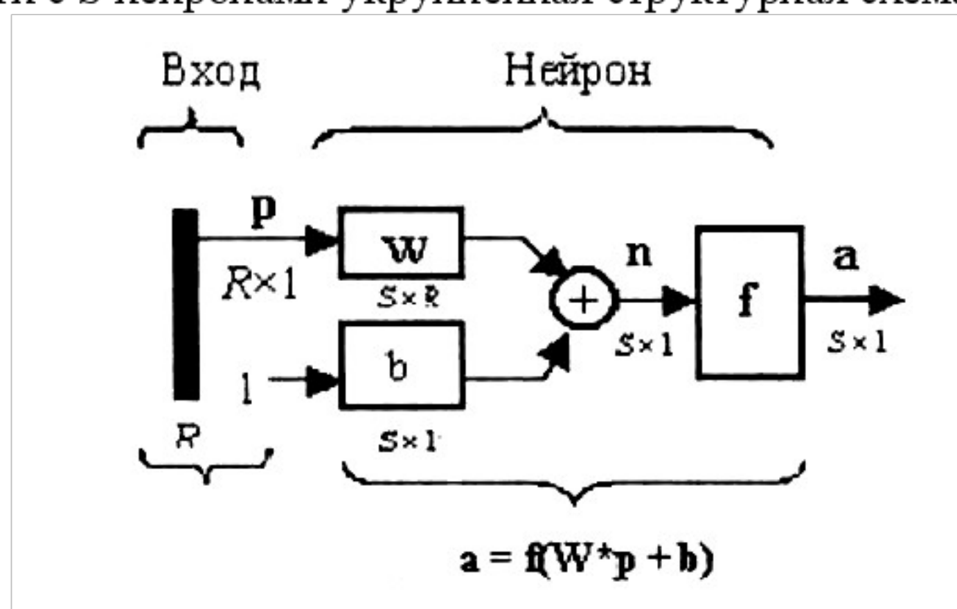
Рис. 7.2. Структурная схема однослойной сети
