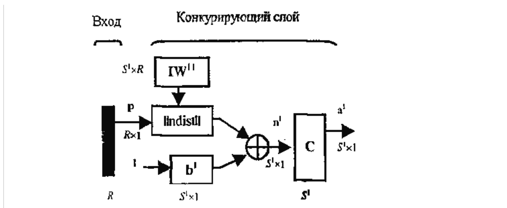
Рис. 12.1. Архитектура слоя Кохонена
