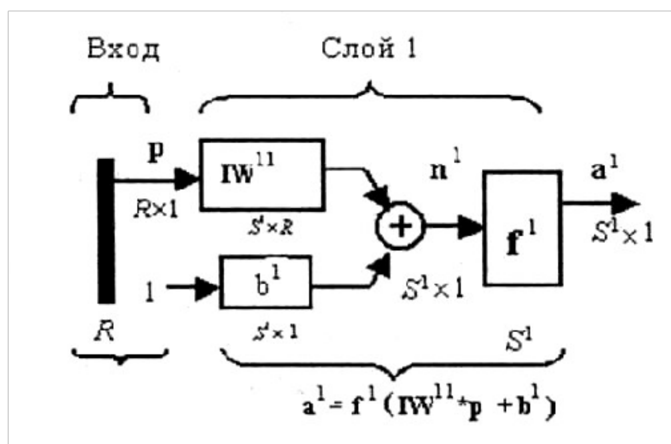
Рис. 7.3. Слой многослойной сети
