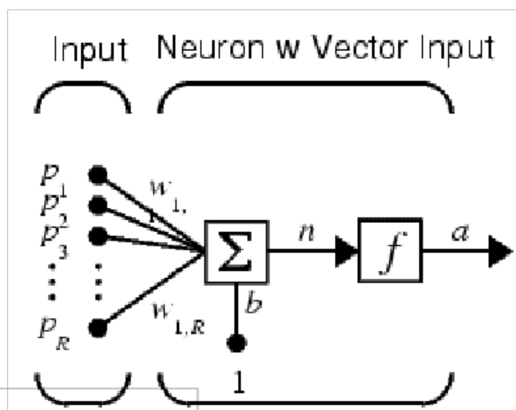
Рис. 6.2. Нейрон с векторным входом
