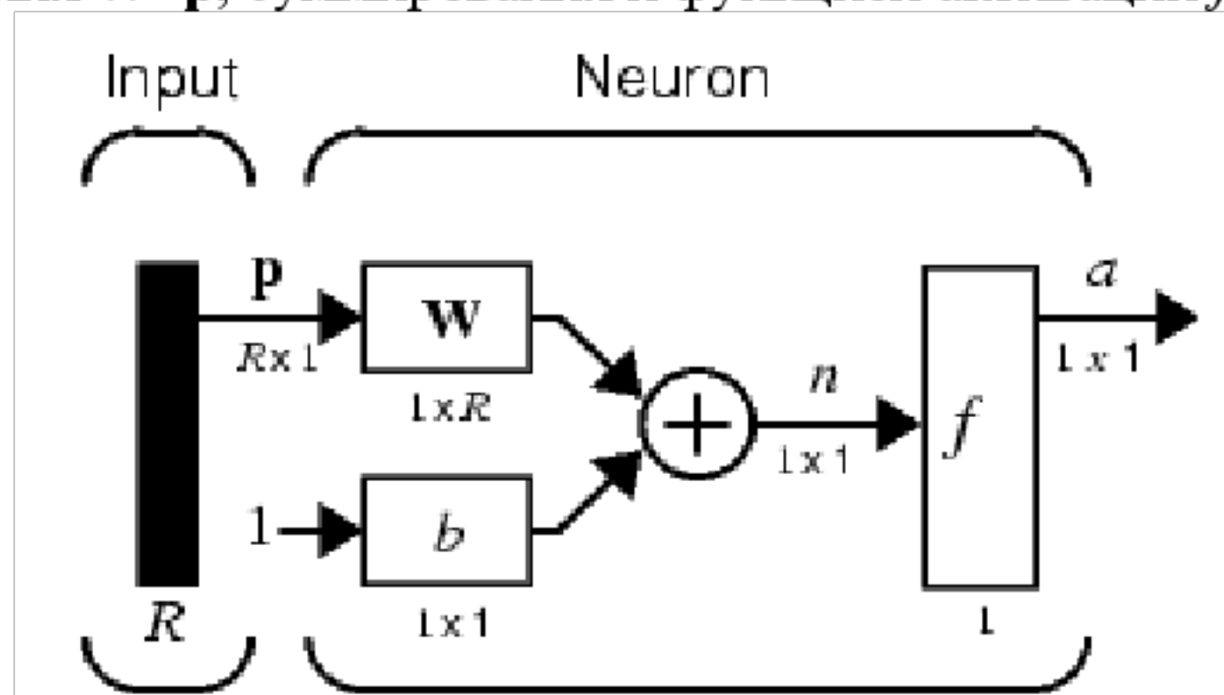
Рис. 6.3. Укрупненная схема нейрона с векторным входом
