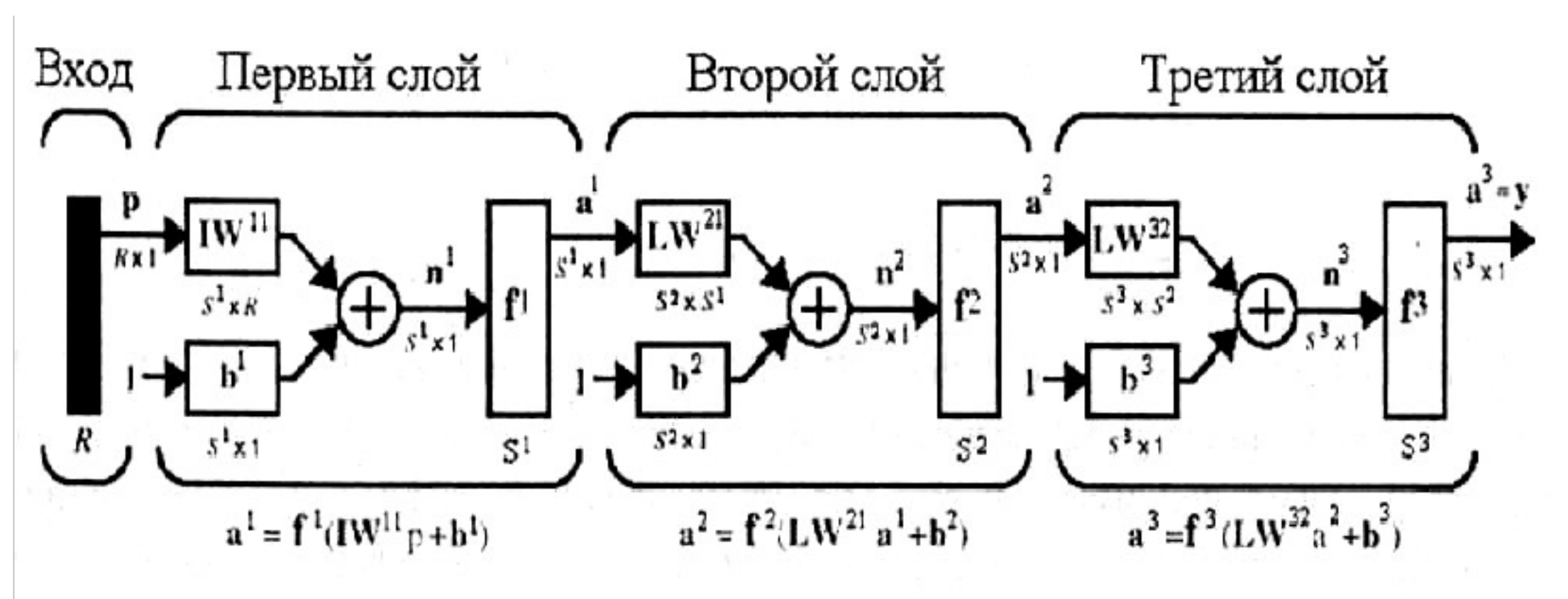
Рис. 7.4. Структурная схема трехслойной сети
