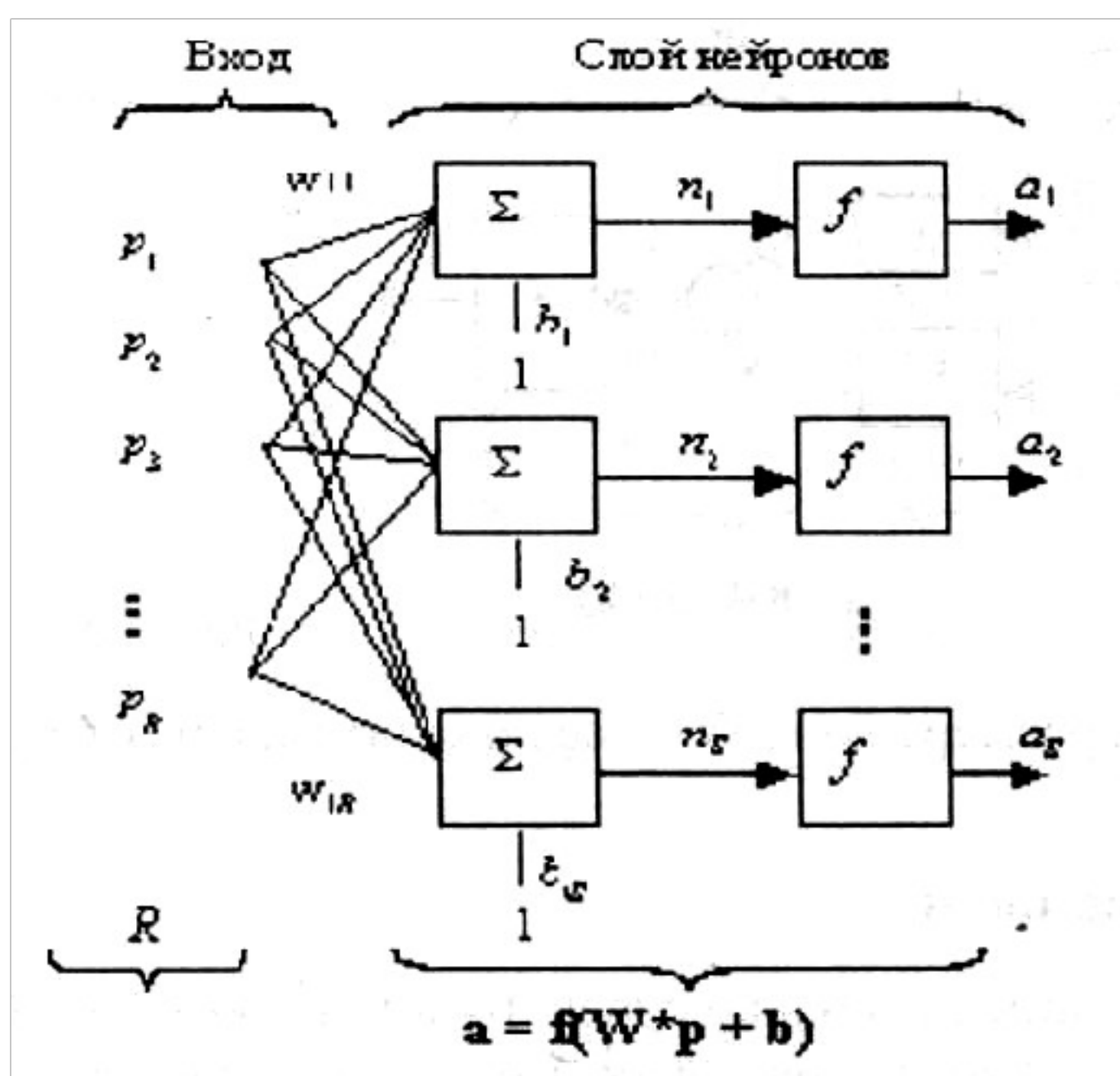
Рис. 7.1. Развернутая схема однослойной сети
