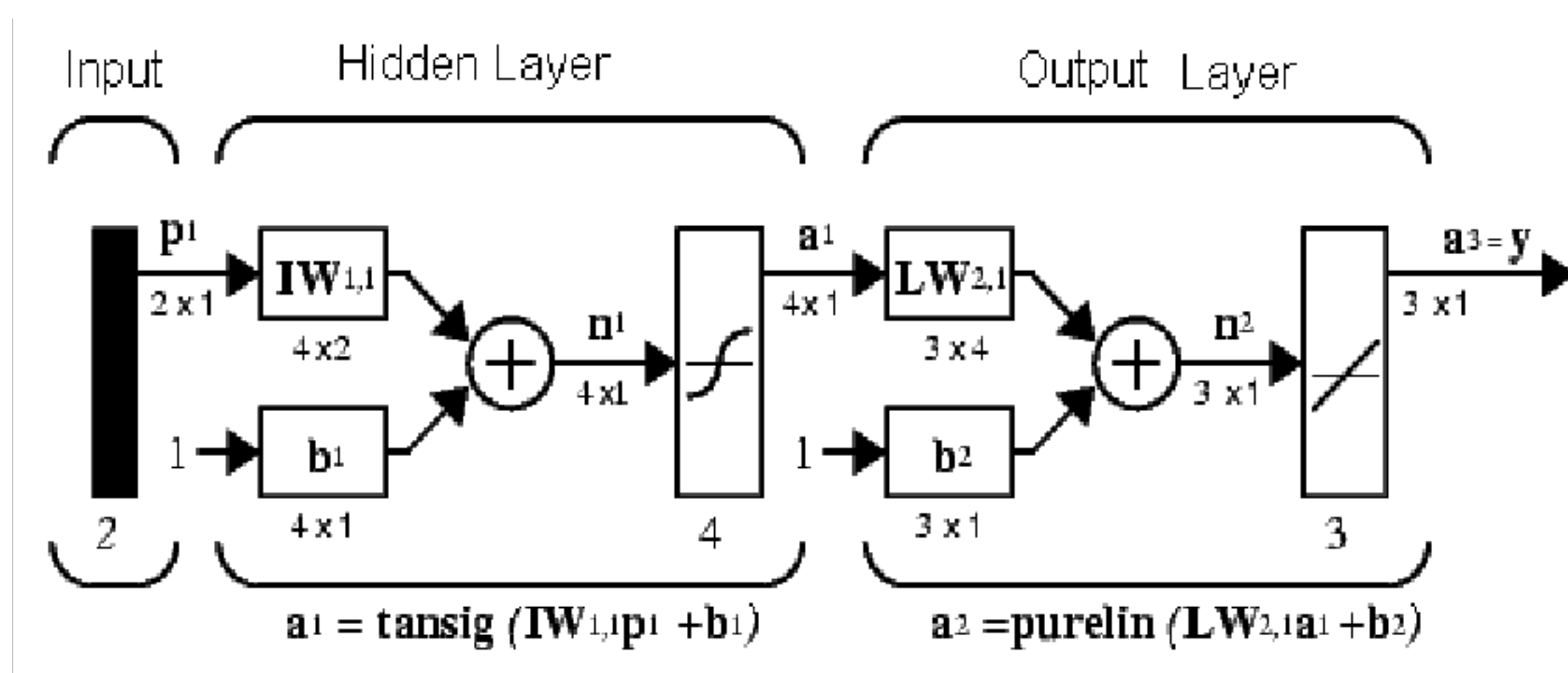
Рис. 7.6. Двухслойная сеть с прямой передачей сигнала
