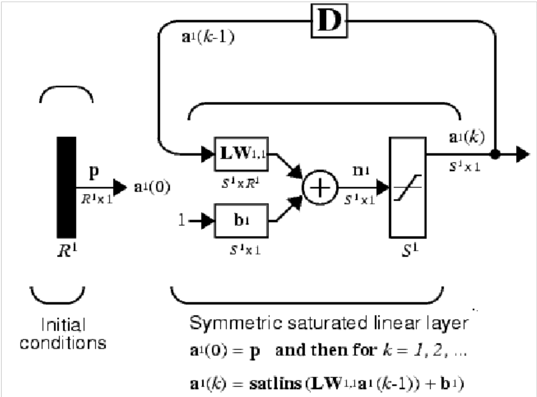
Рис. 13.2. Архитектура сети Хопфилда
