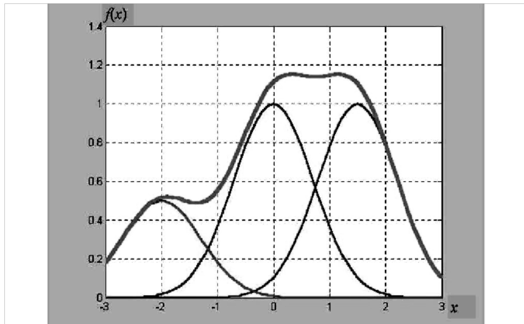
Рис. 4. Функция f(x)
