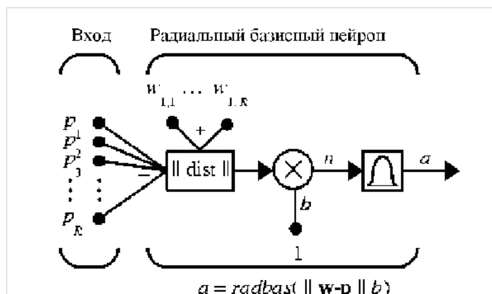
Рис. 1. Радиальный базисный нейрон
