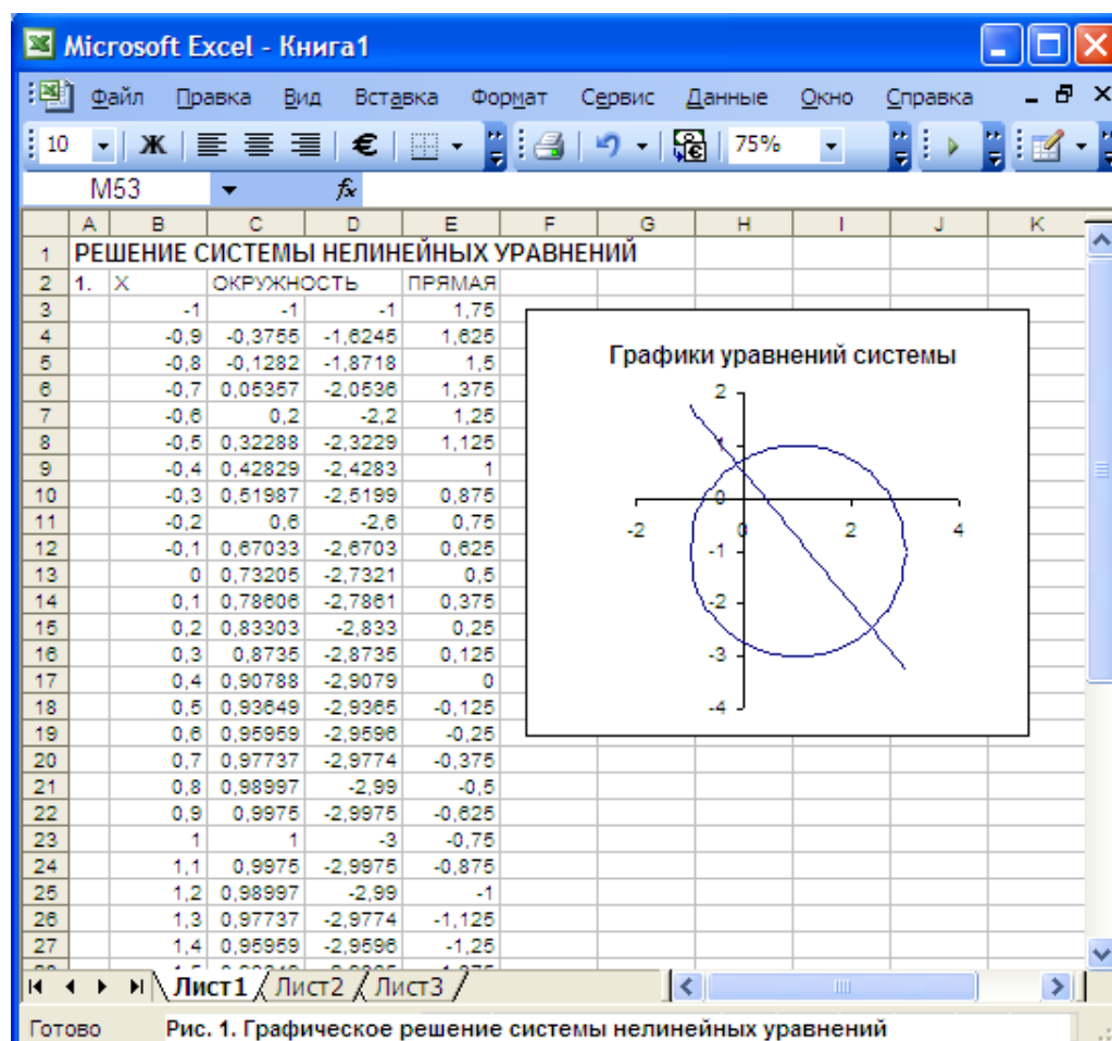
Рис. 1. Графическое решение системы нелинейных уравнений
