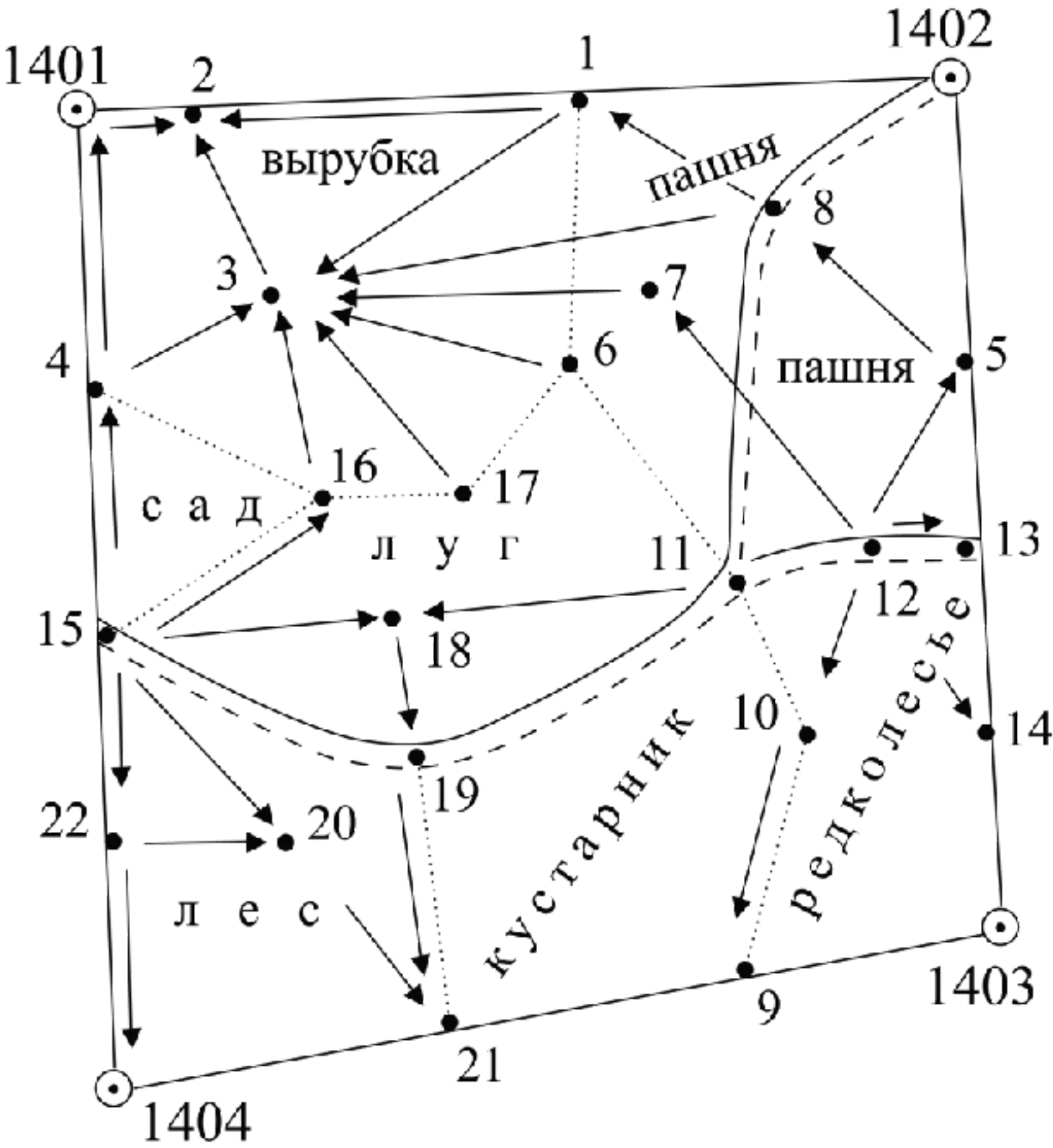
Абрис тахеометрической съемки.
