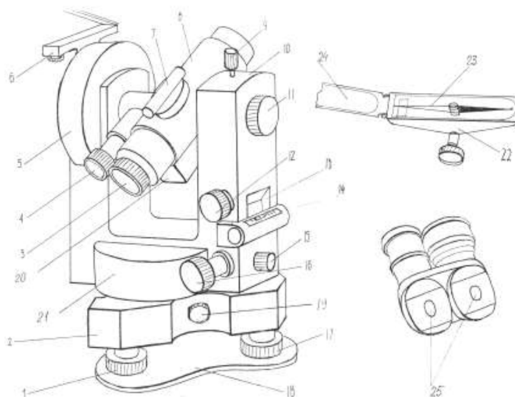
Рис.1 Теодолит 4Т-30П
