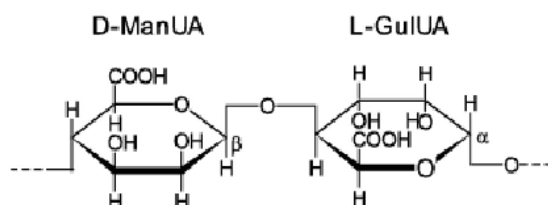
Рисунок 5.3 - Молекула альгиновой кислоты
