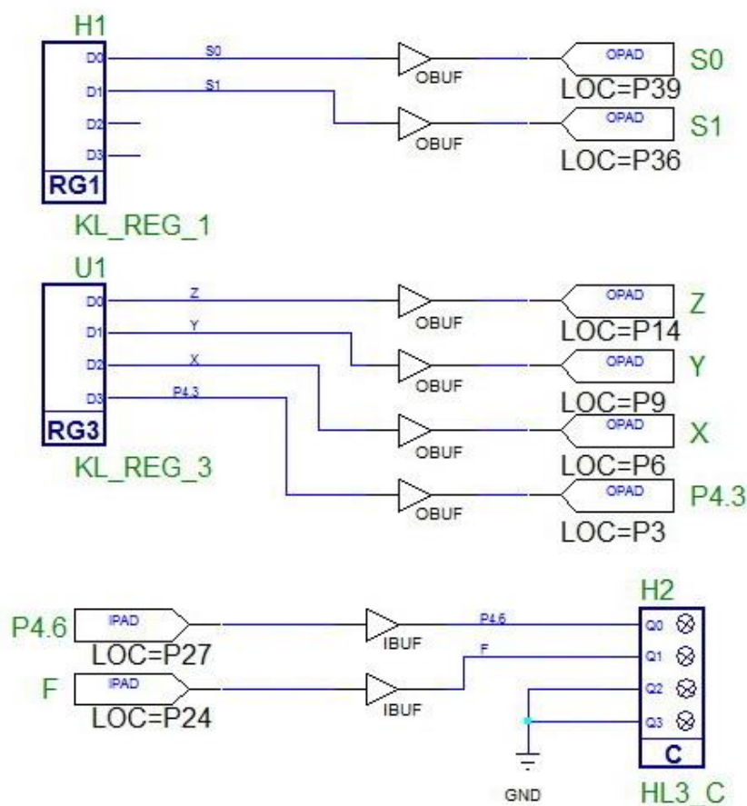
Рис. 27.2. Схема источника и приемника сигналов – проект, загружаемый в ПЛИС
