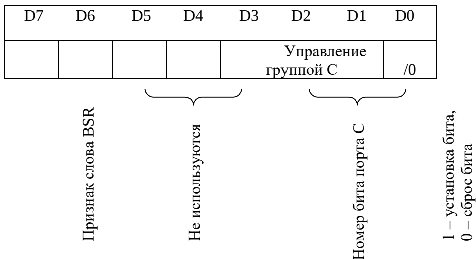
Рис. 3. Формат регистра BSR
