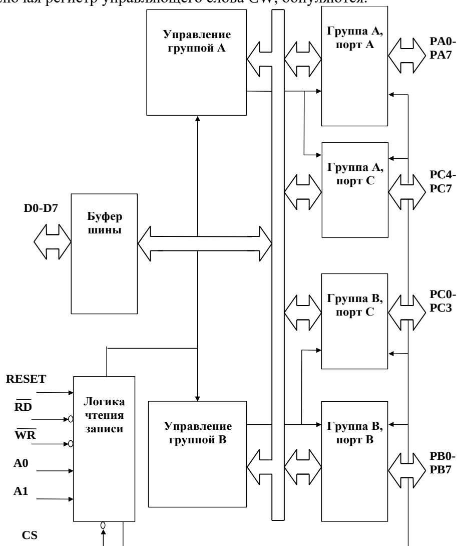
Рис. 1. Структурная схема БИС ППА К580ВВ55А
