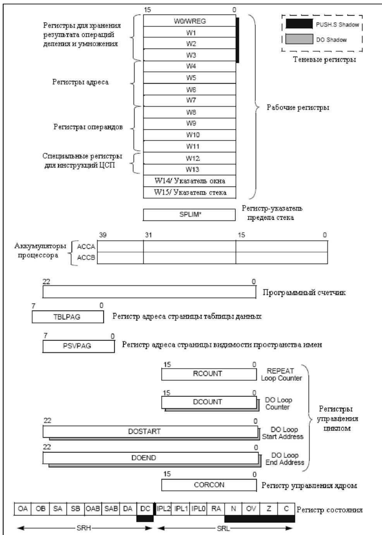
Рисунок 8 - Регистры микропроцессора
