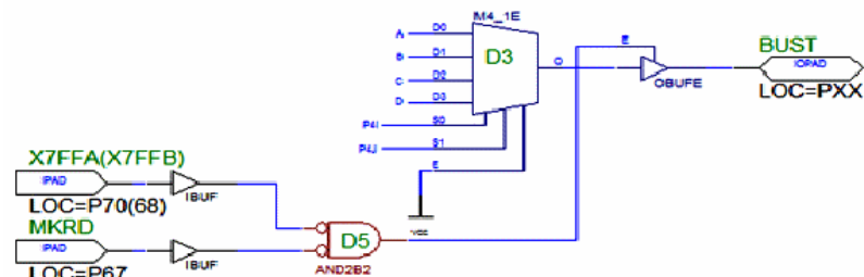
Рис. 29.9. Вариант подключения четырёх источников через мультиплексор (управление от порта P4)
