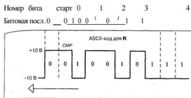
Рисунок 1.-Сигнал стандарта RS232C при передаче символа «R».
