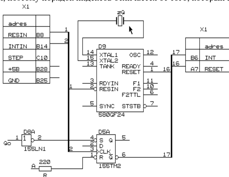
Рис. 2 Схема формирования сигнала “RESET”
