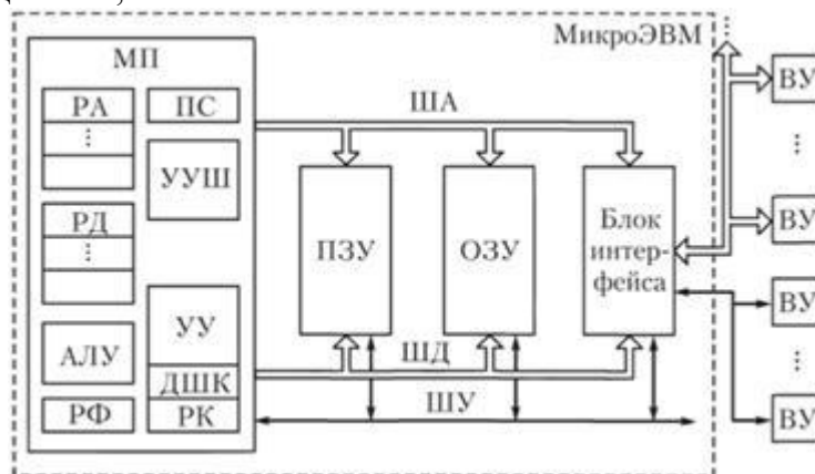
Рис. 1. Структура микропроцессорной системы
