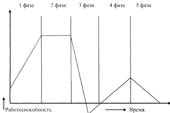
Рисунок 1.2.1 – Динамика работоспособности [5]
