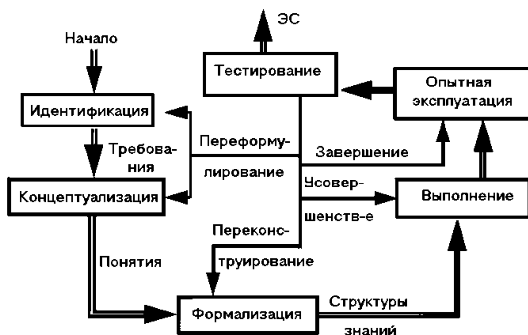
Рис. 4.3. технология разработка ЭС
