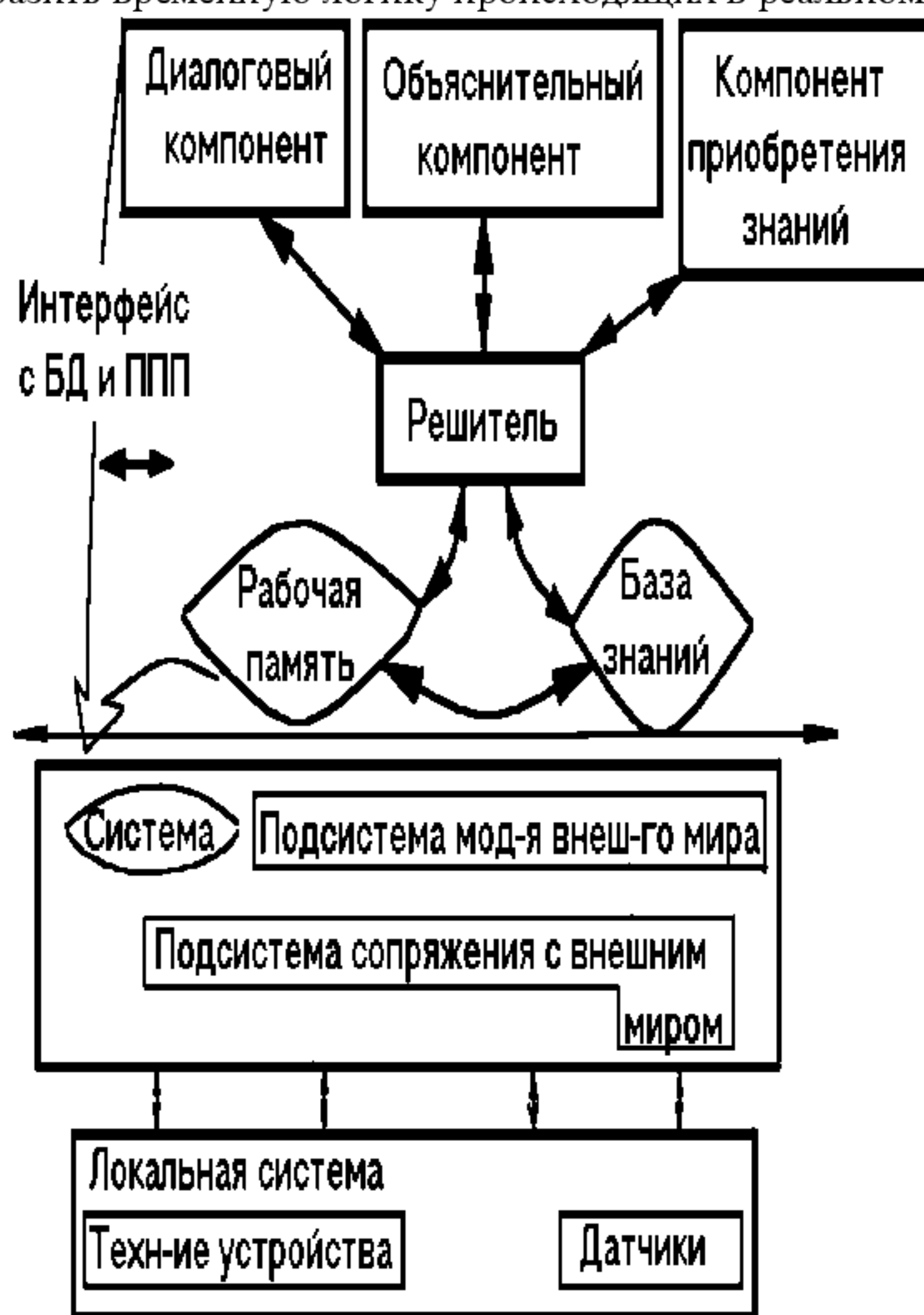
Рис. 4.2. Структура статической ЭС
