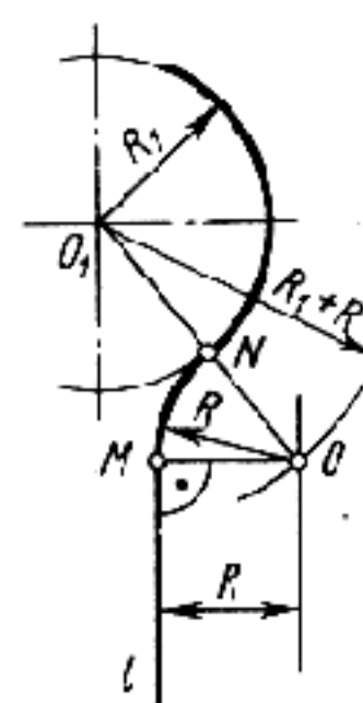
Рис. 6 Сопряжение прямой линии с дугой.
