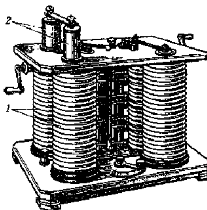
Рисунок 9 Трансформатор Голяра и Гиббса
