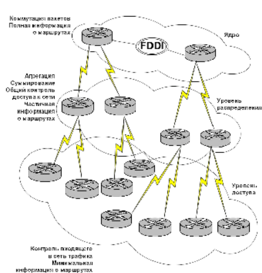
Рисунок 10 – Структура иерархической сети
