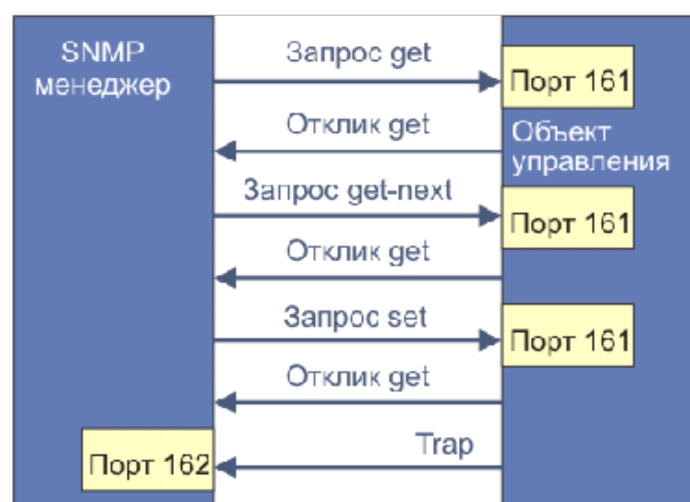
Рисунок 18 - Архитектурная модель SNMP
