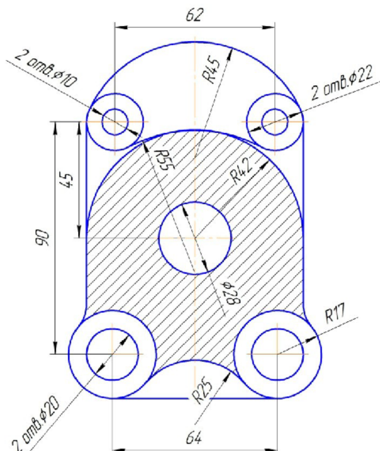
Остов
