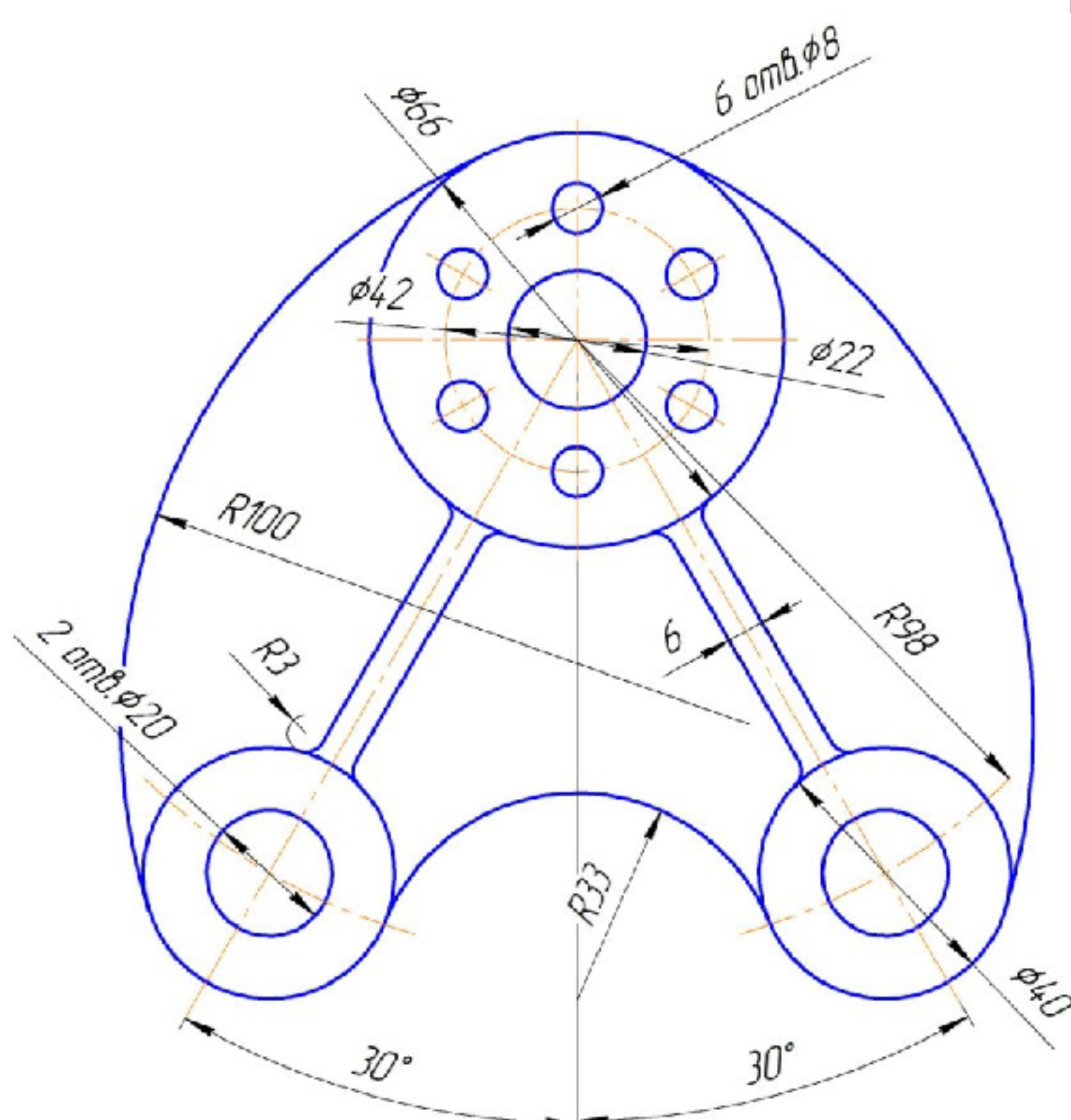
Вилка
