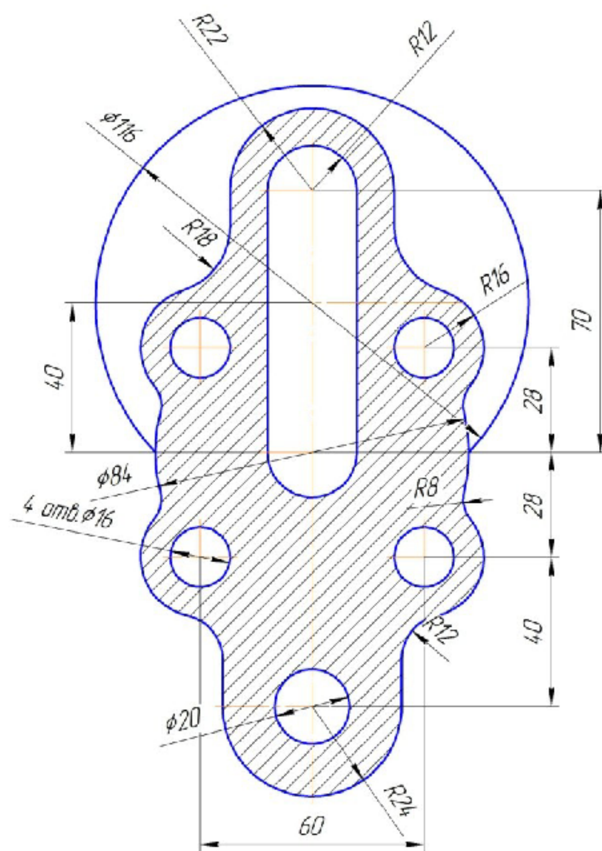
Крышка
