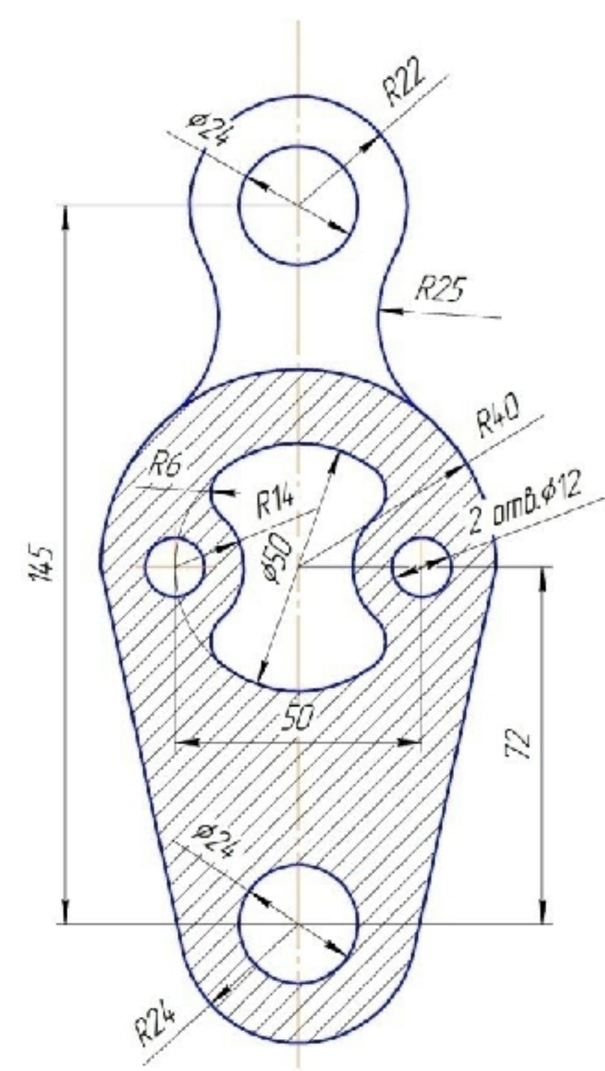
Подвеска
