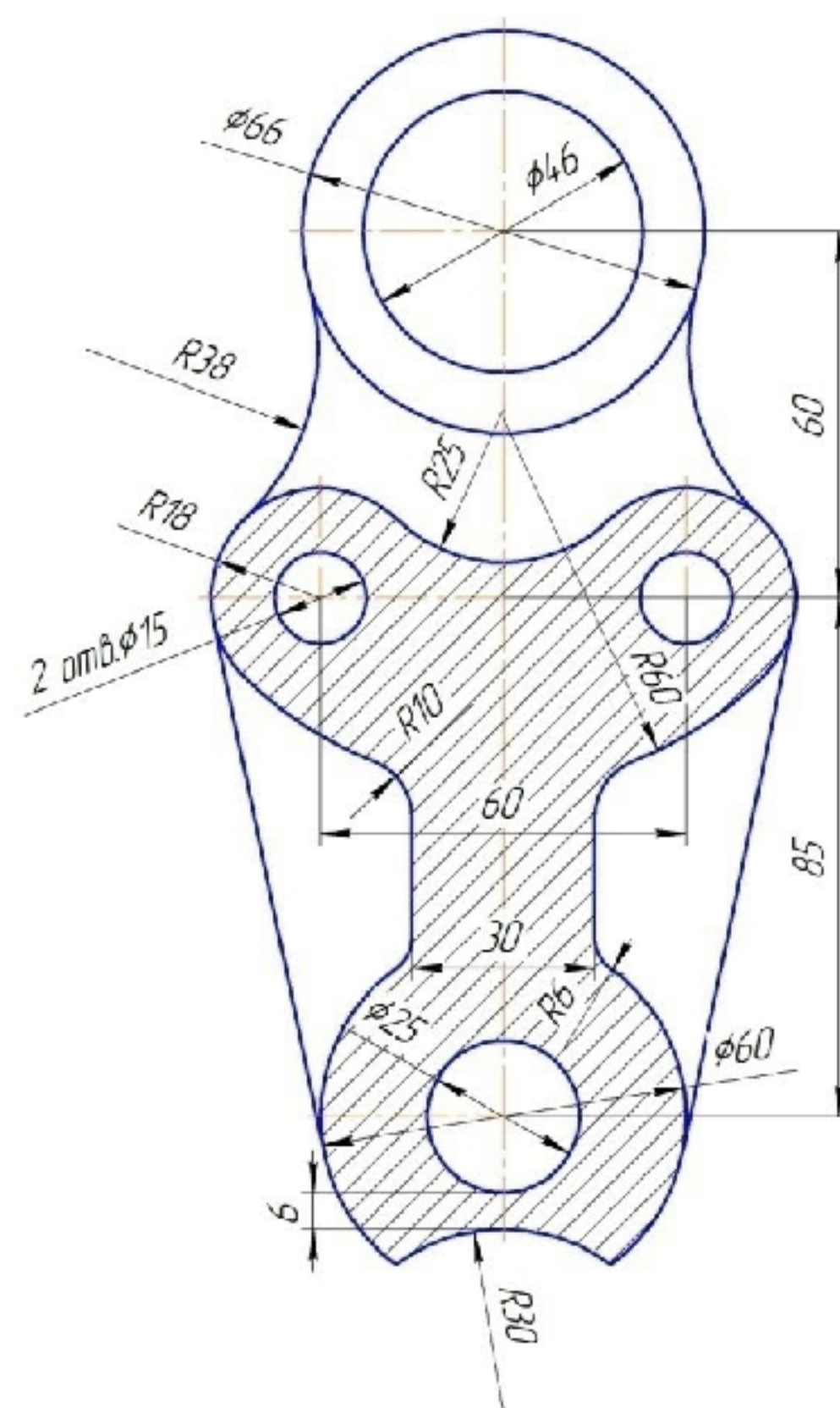
Кондуктор
