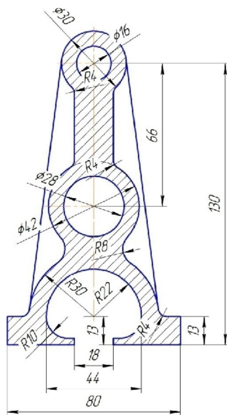
Стойка
