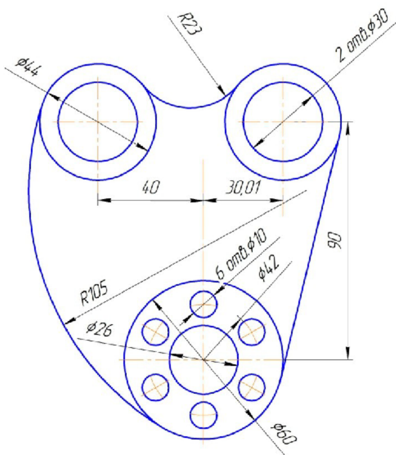
Ушко
