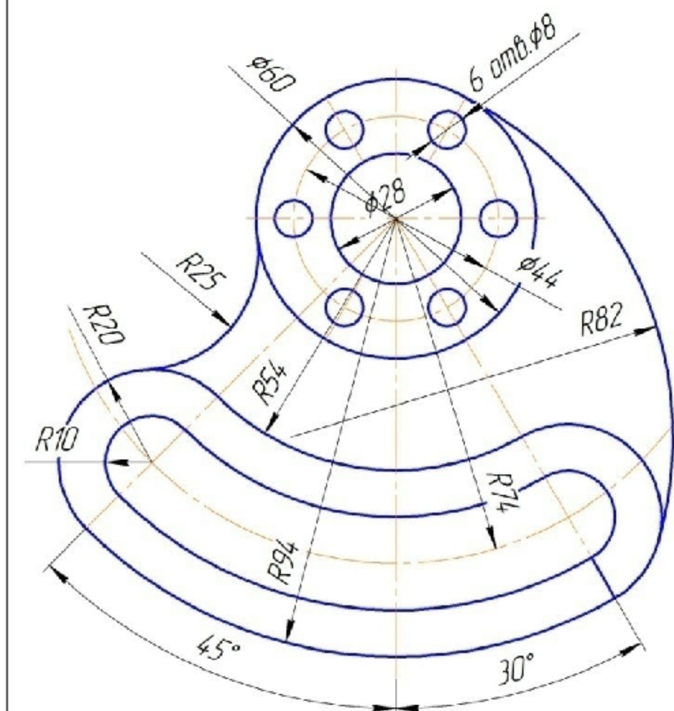
Гитара
