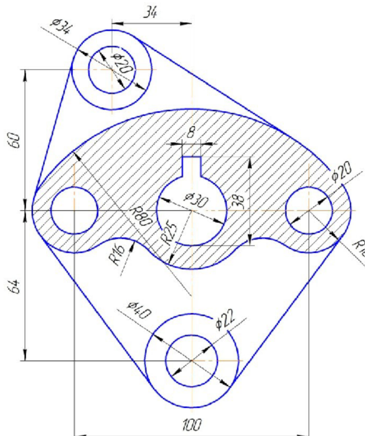
Рычаг
