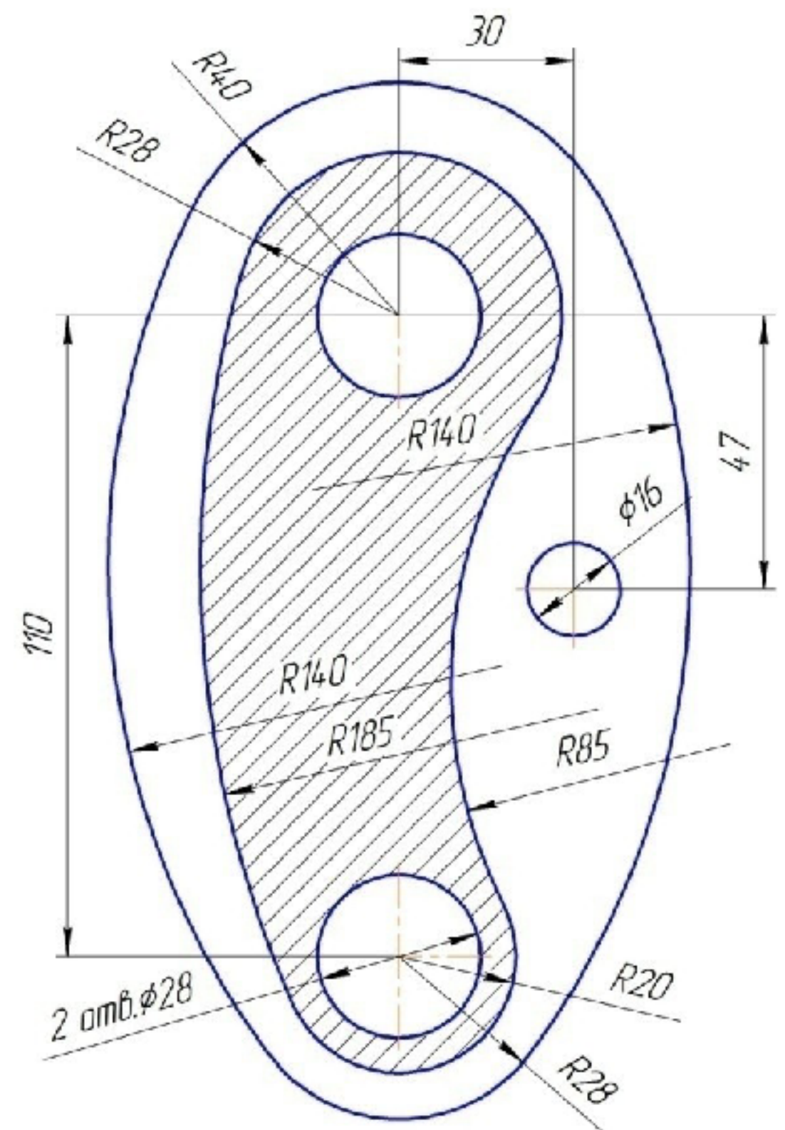
Коромысло
