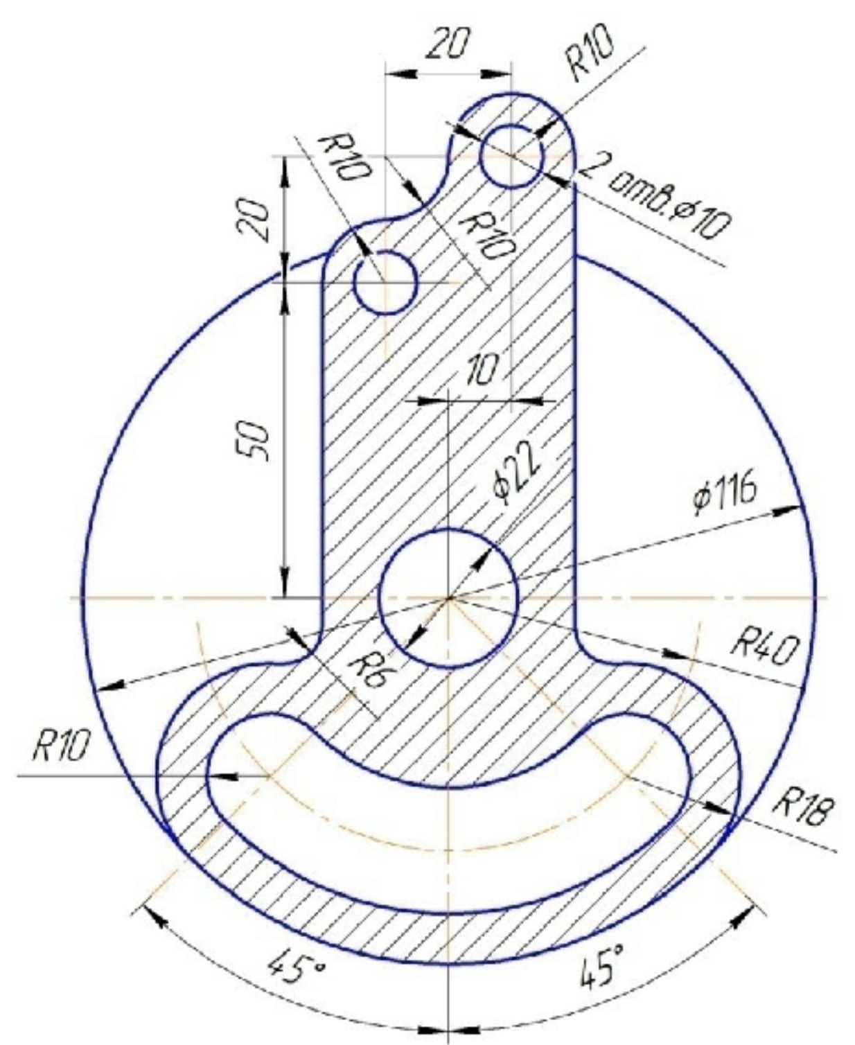
Патрон
