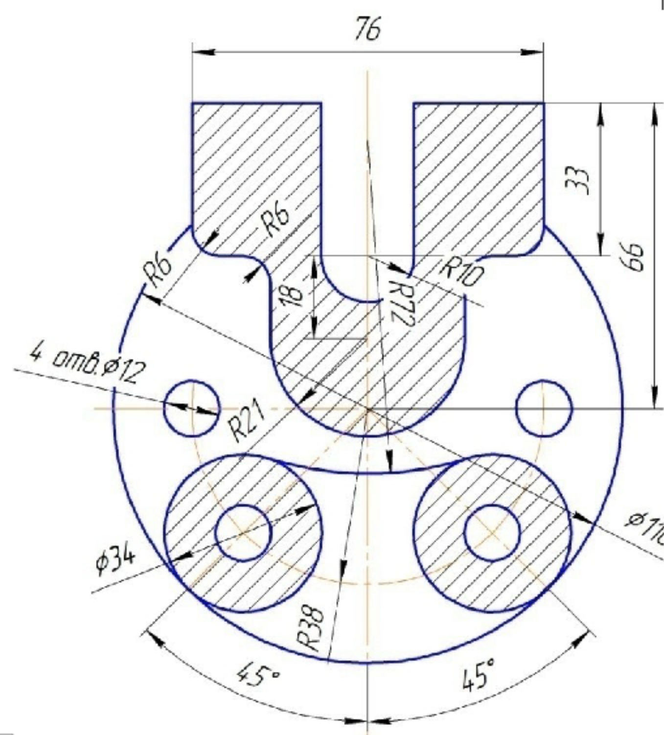
Корпус
