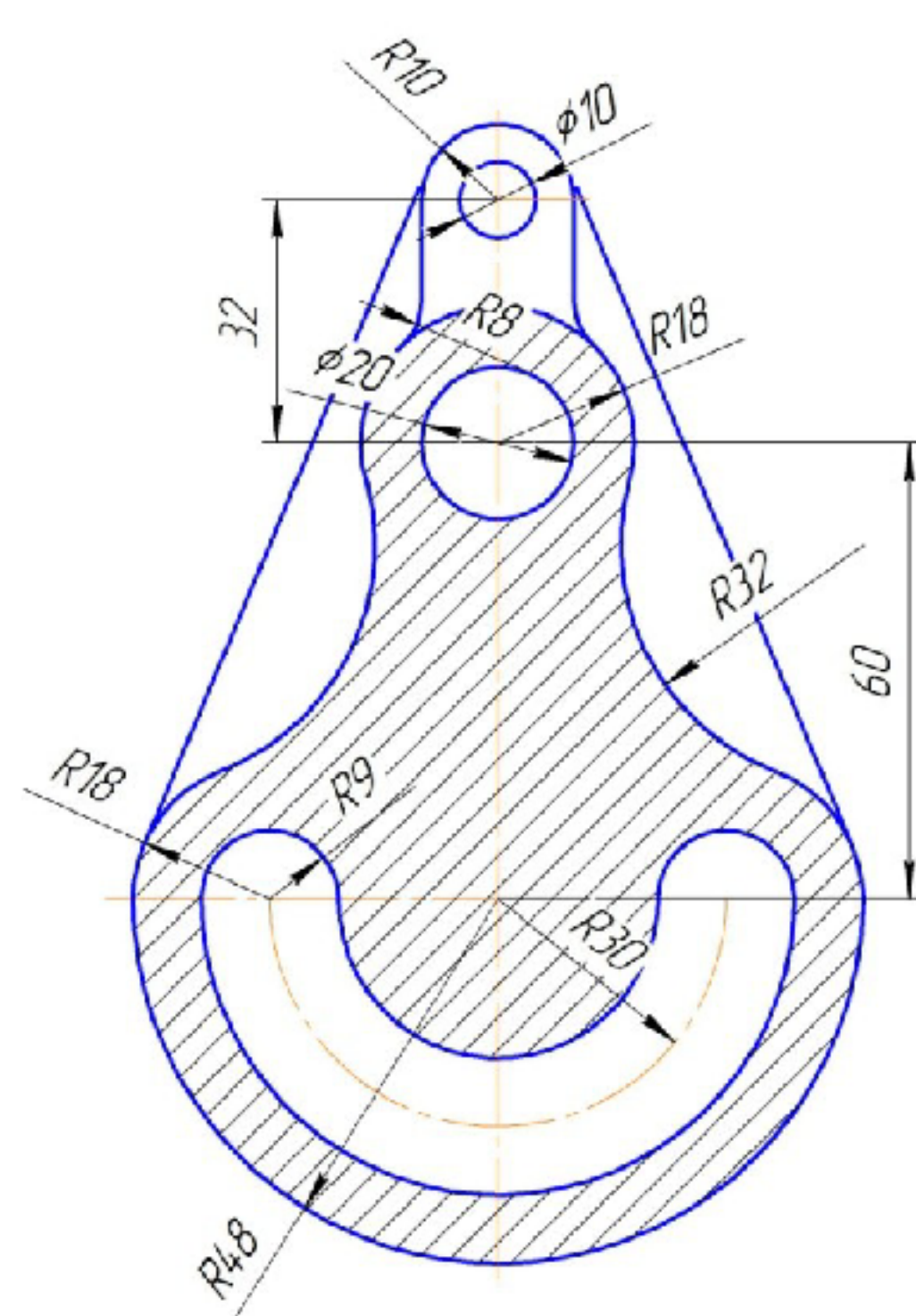
Корпус
