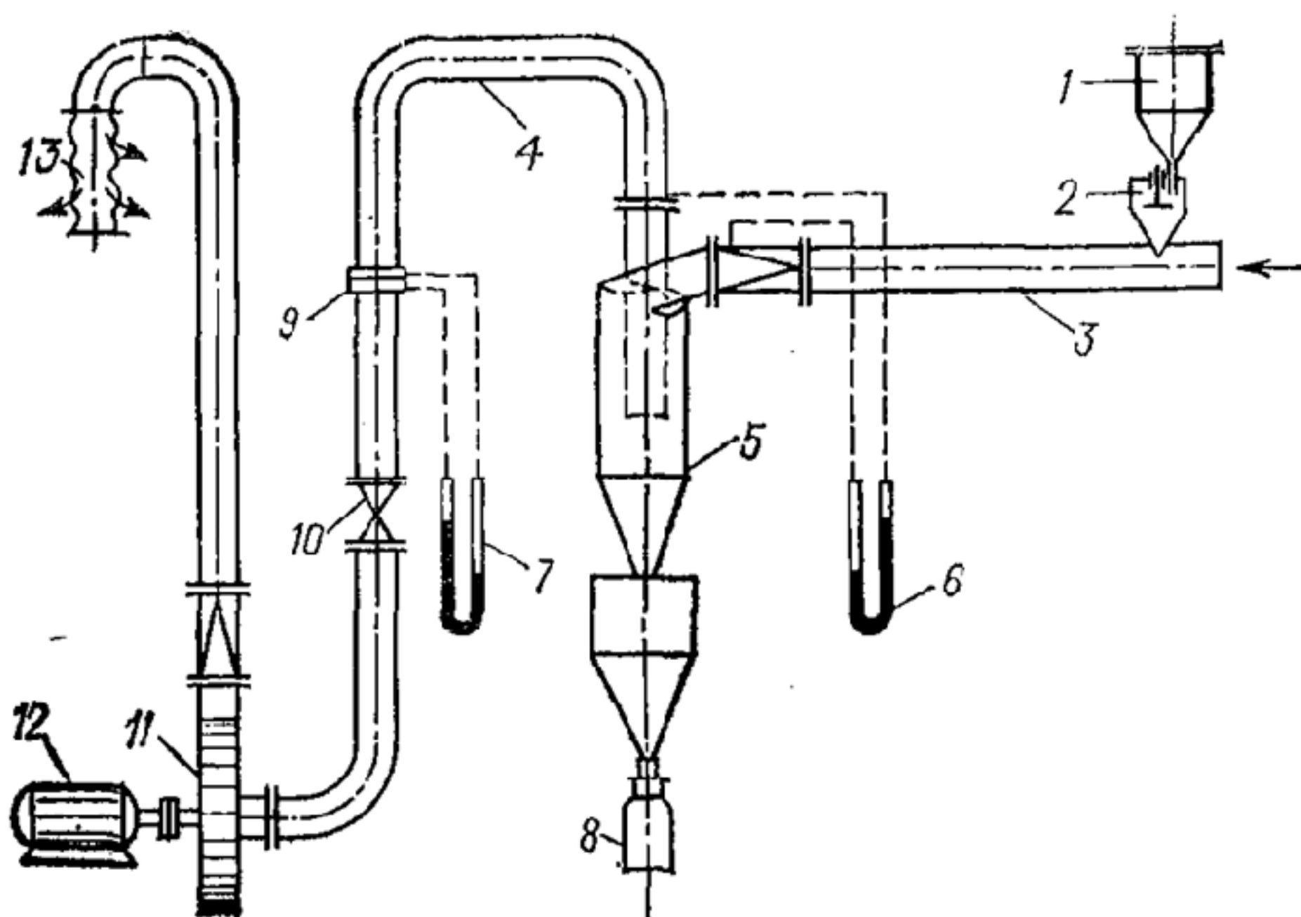
Рис. 2. Схема установки:
