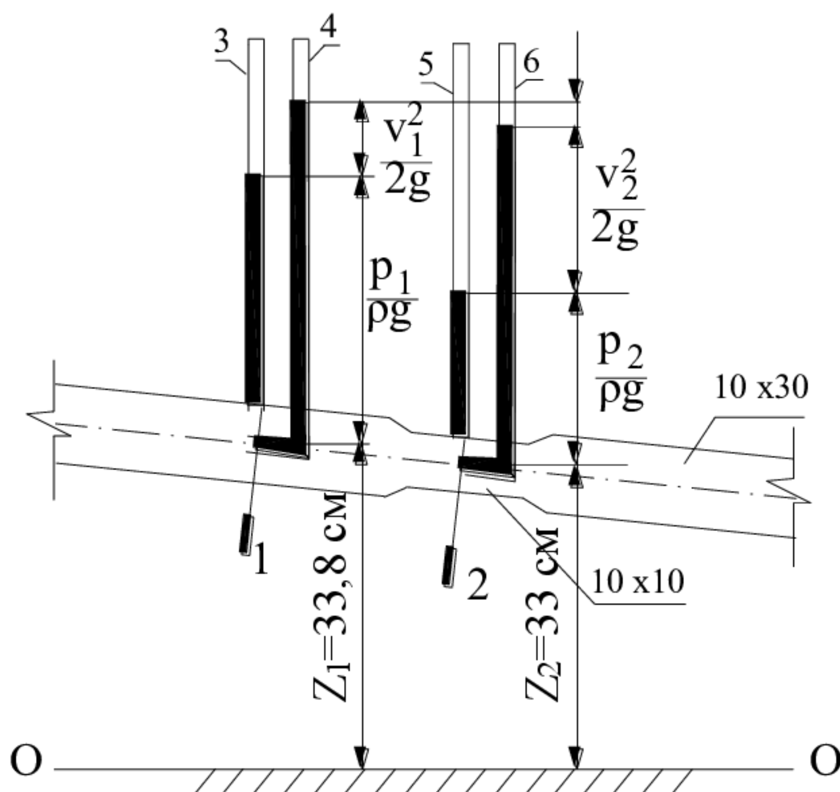
Рисунок 3.1 Расчетная схема трубчатого расходомер (расходомера Вентури)
