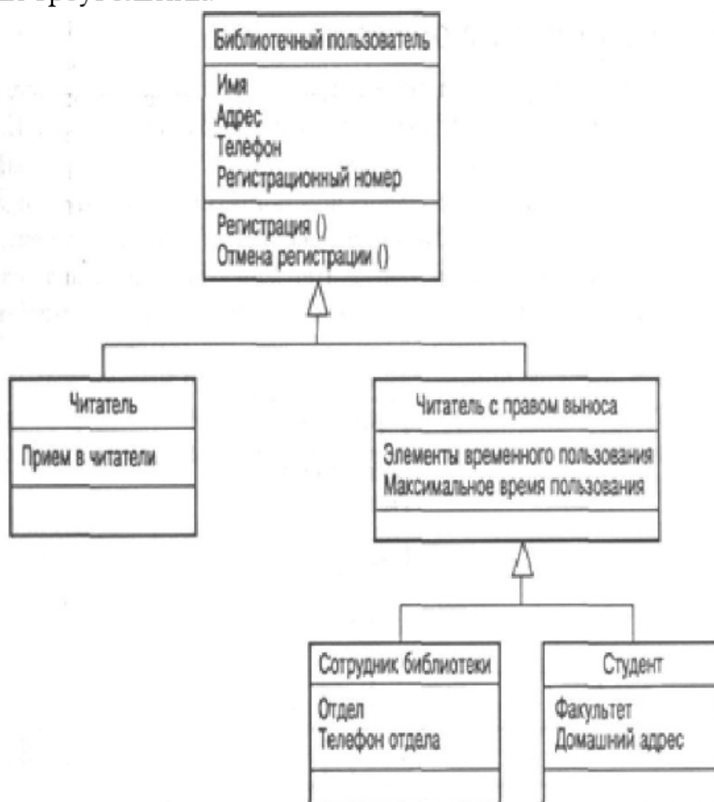
Рис. 12. Пример связи наследование
