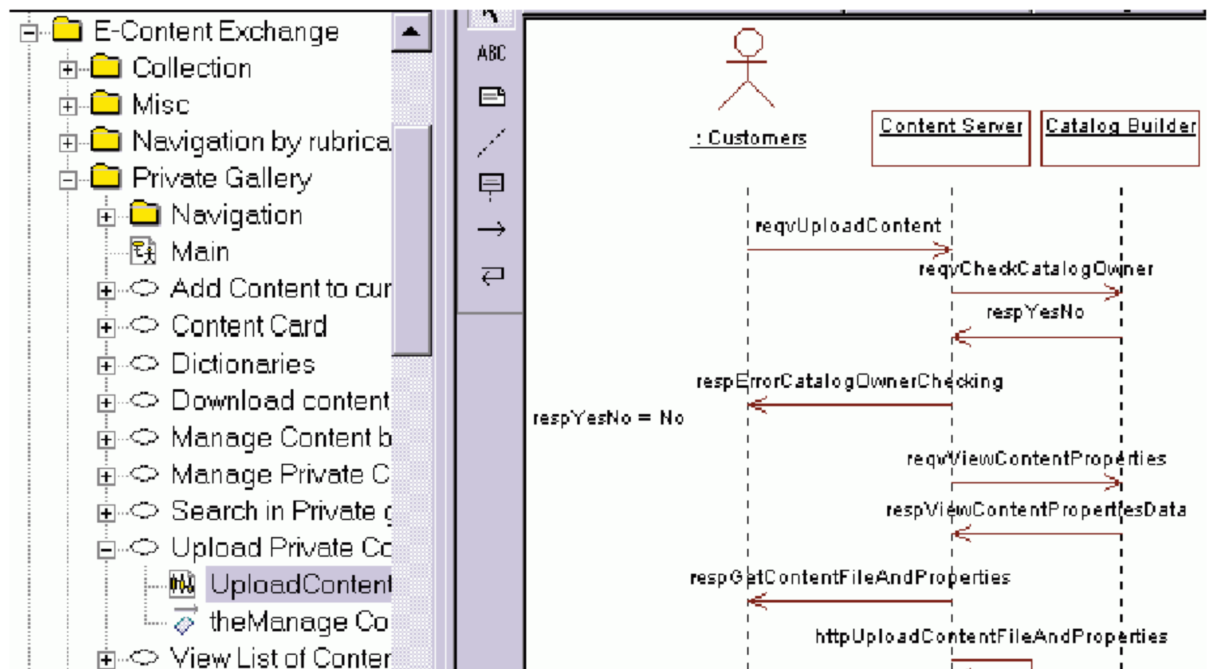
Рисунок 4 - Описание механизма вызова компонентов
