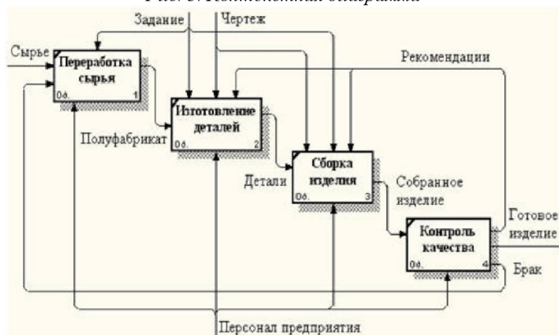
Рис.4. Диаграмма первого уровня декомпозиции
