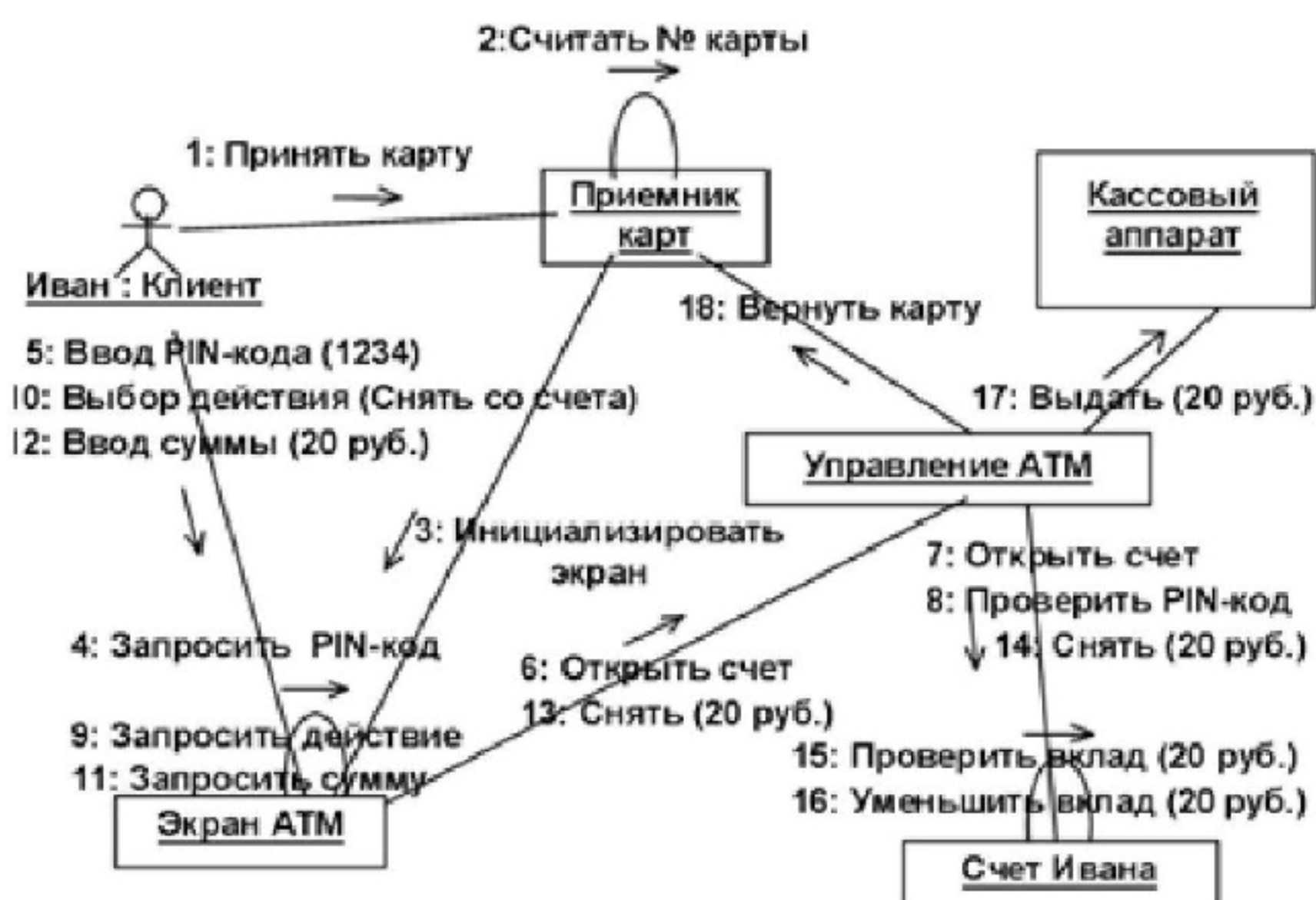
Рис. 8. Пример диаграммы кооперации
