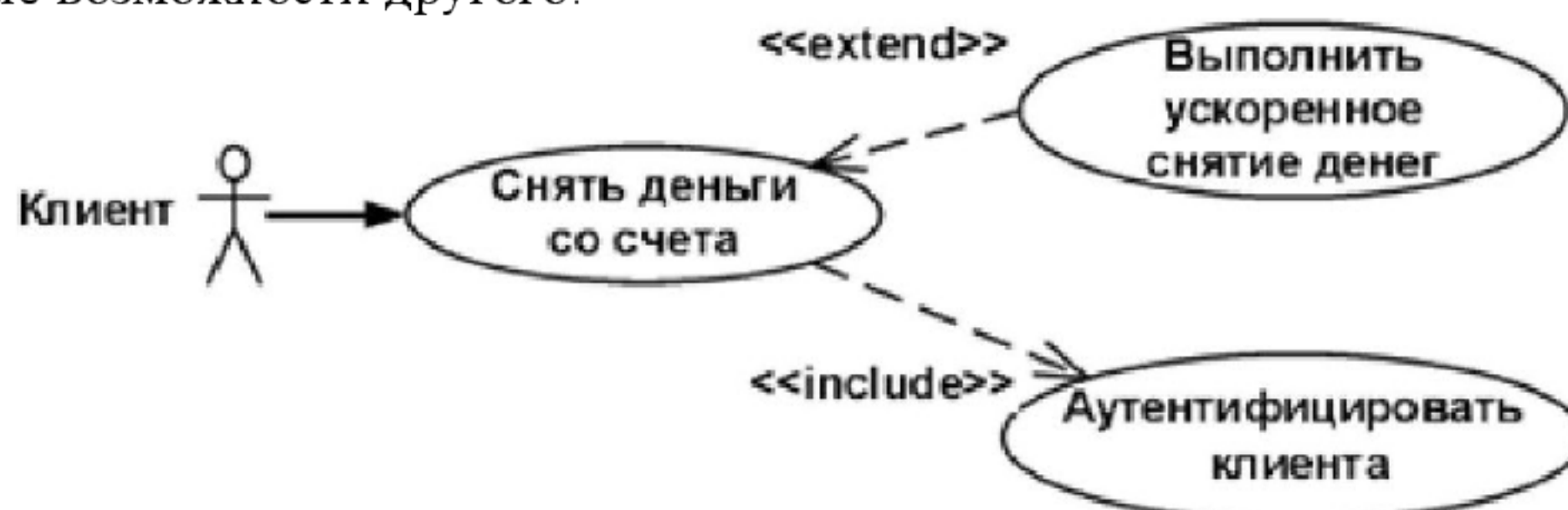
Рис.5. Пример связи включения и расширения
