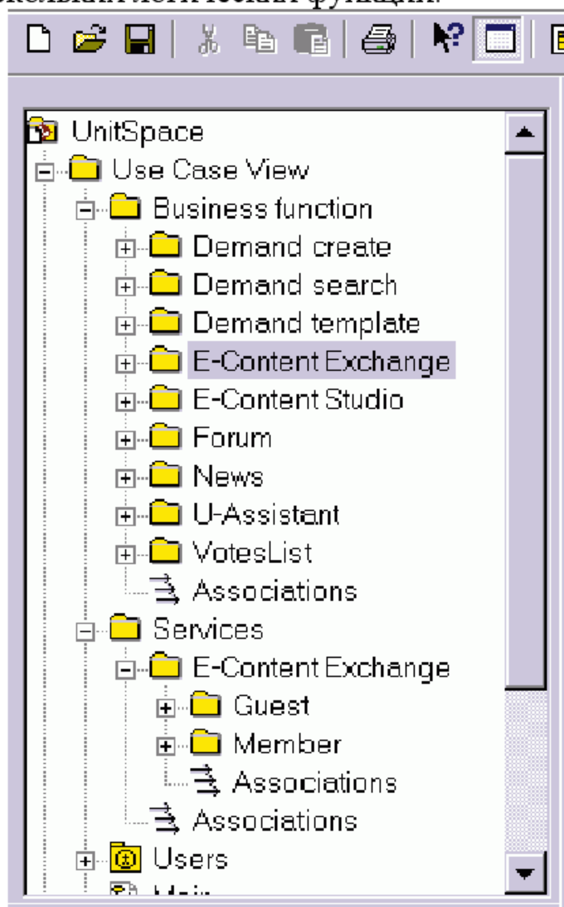
Рисунок 3 - Список бизнес-функций
