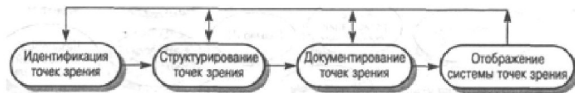
Рис. 3. Метод VORD
