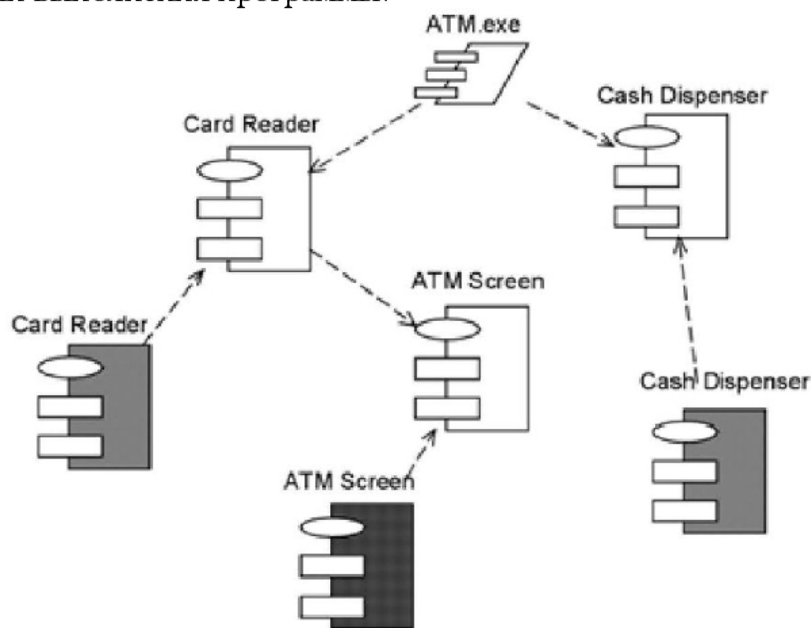
Рис. 18. Пример диаграммы компонентов
