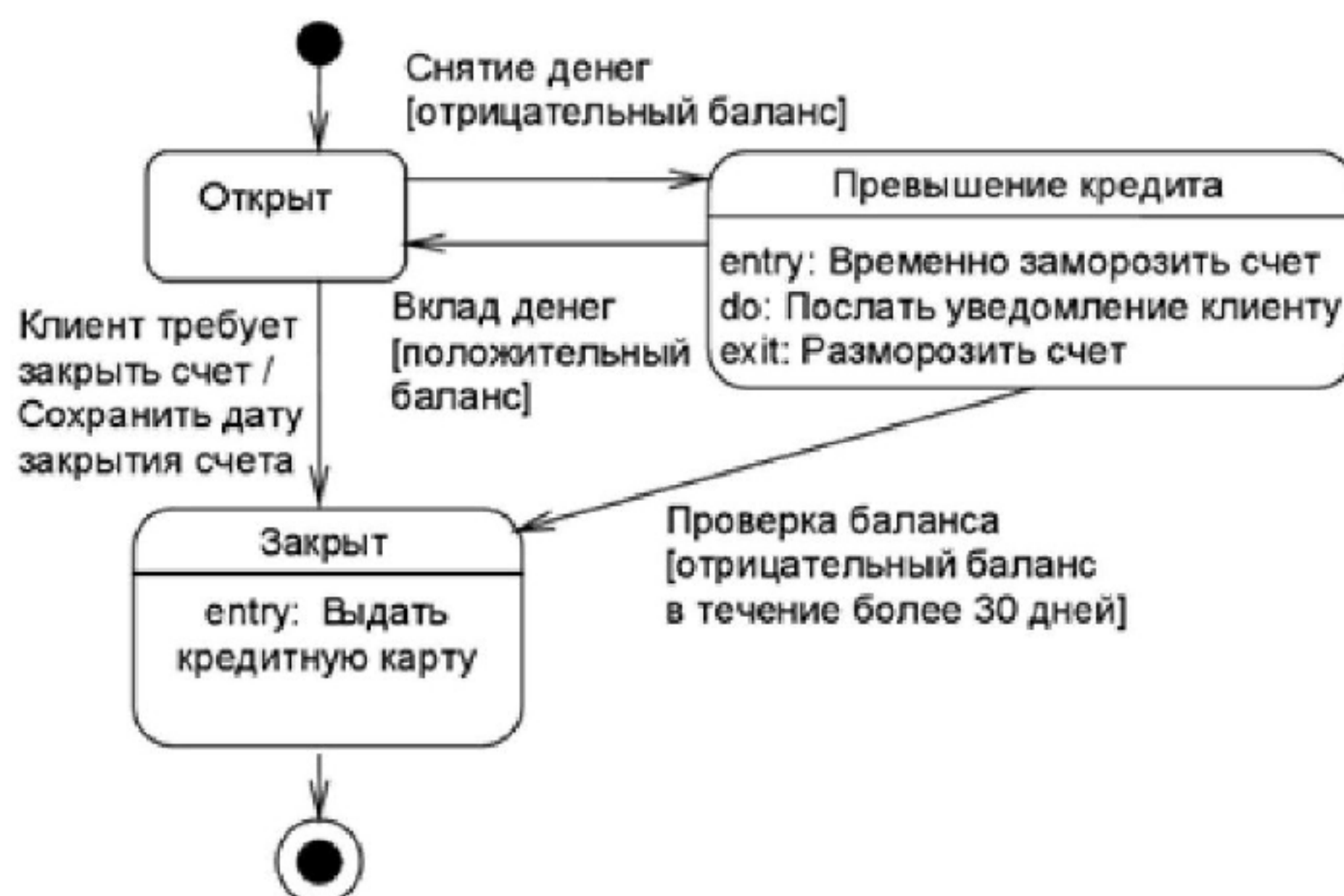
Рис. 17. Пример диаграммы состояний
