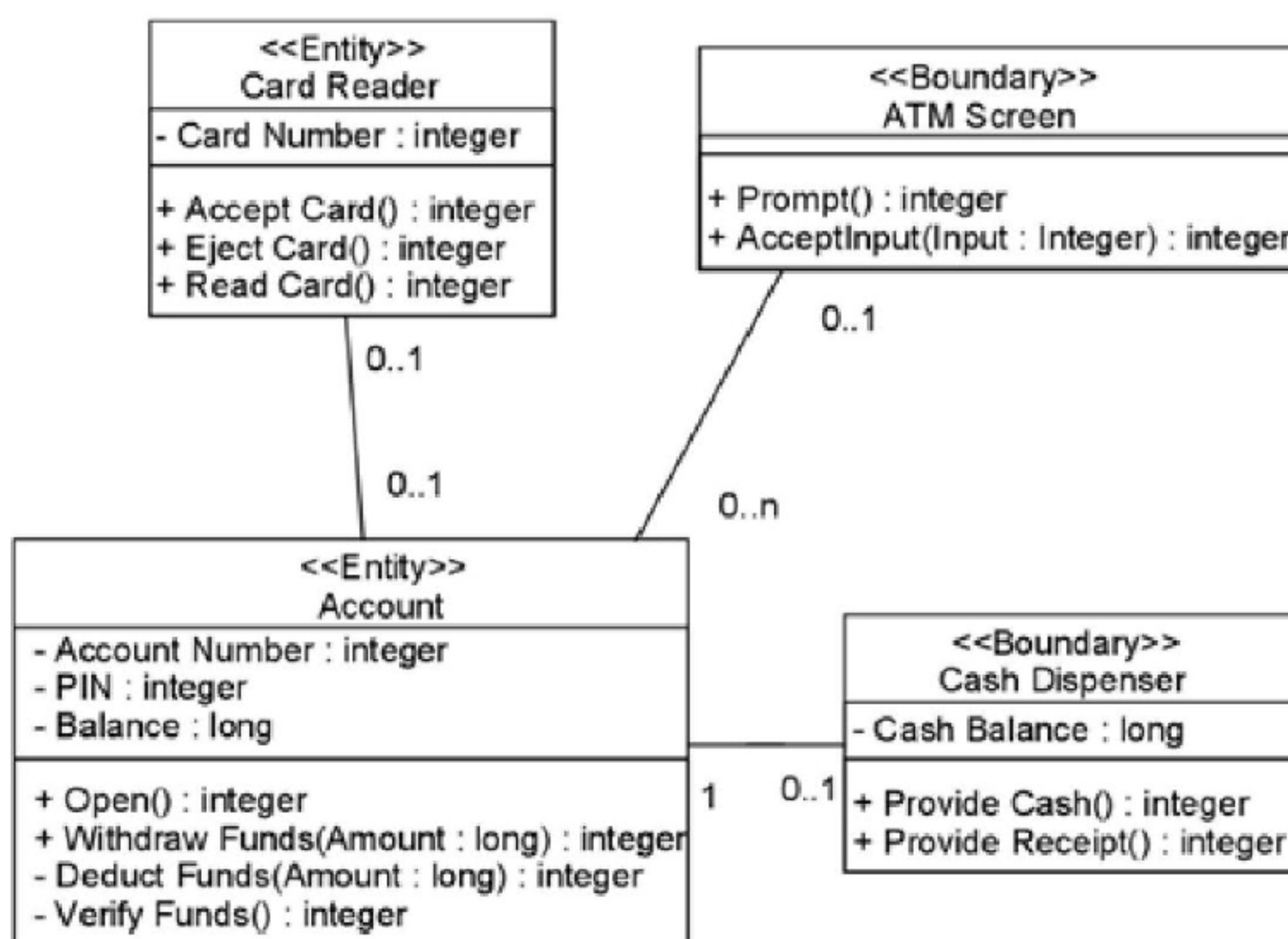
Рис. 9. Пример диаграммы классов
