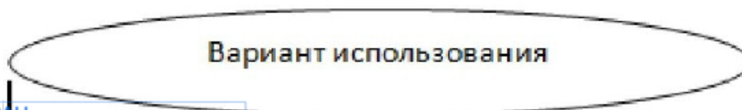
Рис.2. Вариант использования
