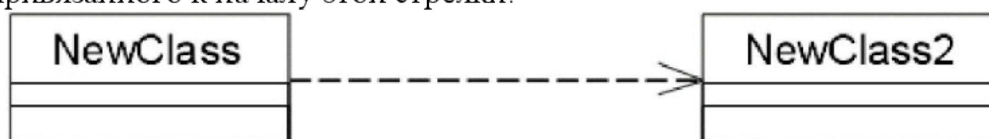
Рис. 11. Связь зависимость
