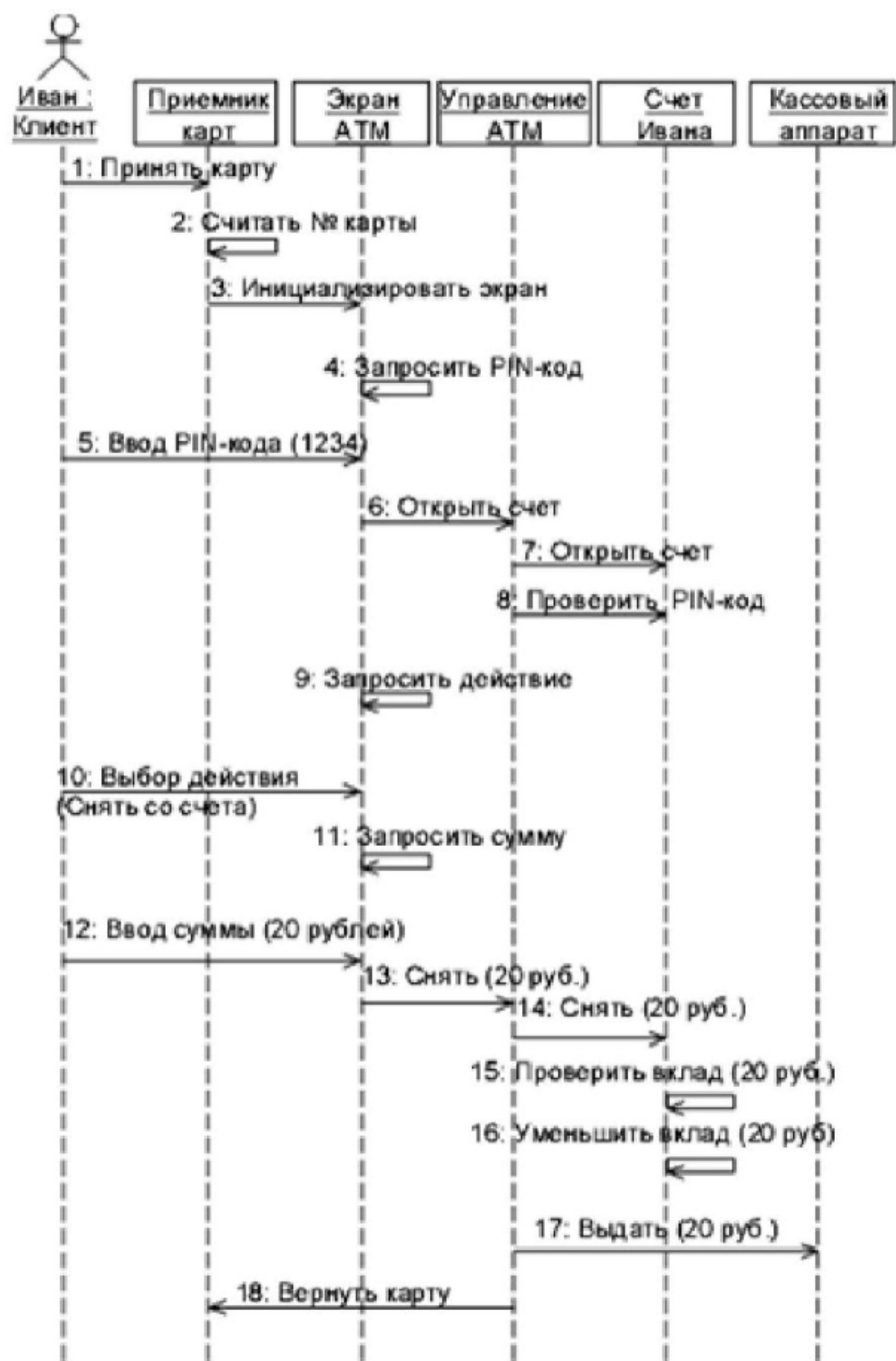
Рис. 7. Пример диаграммы последовательности
