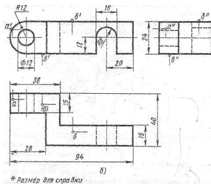
б) Эскиз детали.
