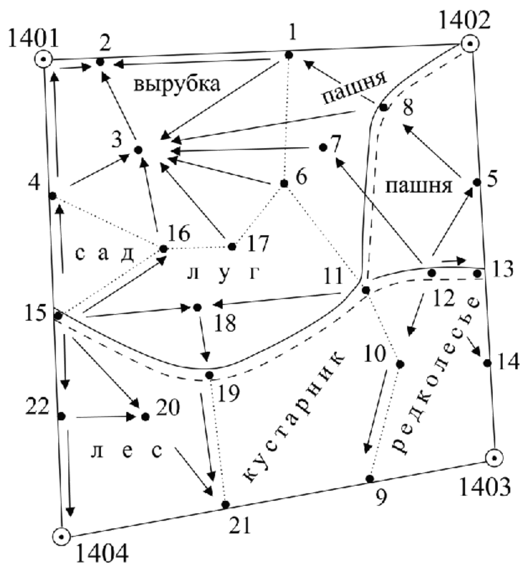
Абрис тахеометрической съемки.
