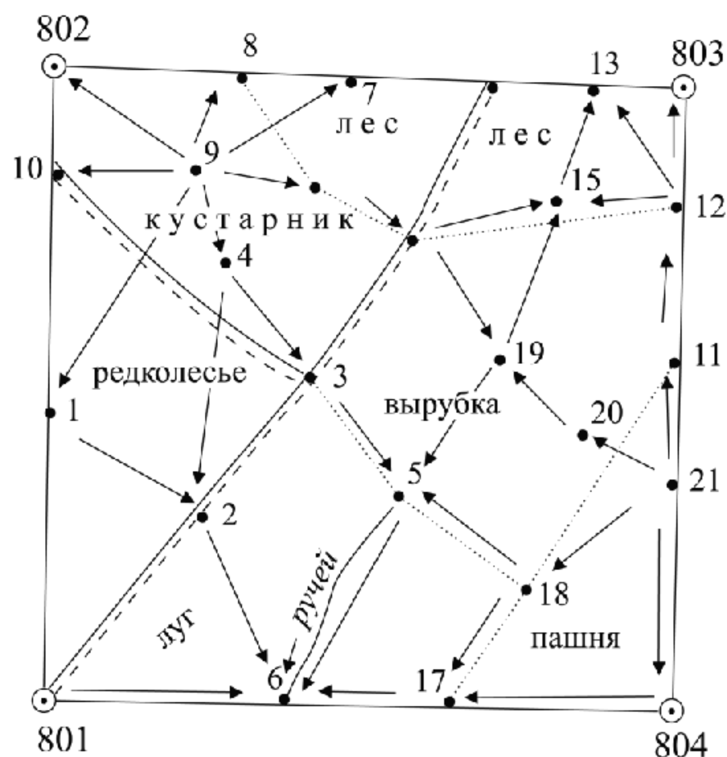
Абрис тахеометрической съемки.
