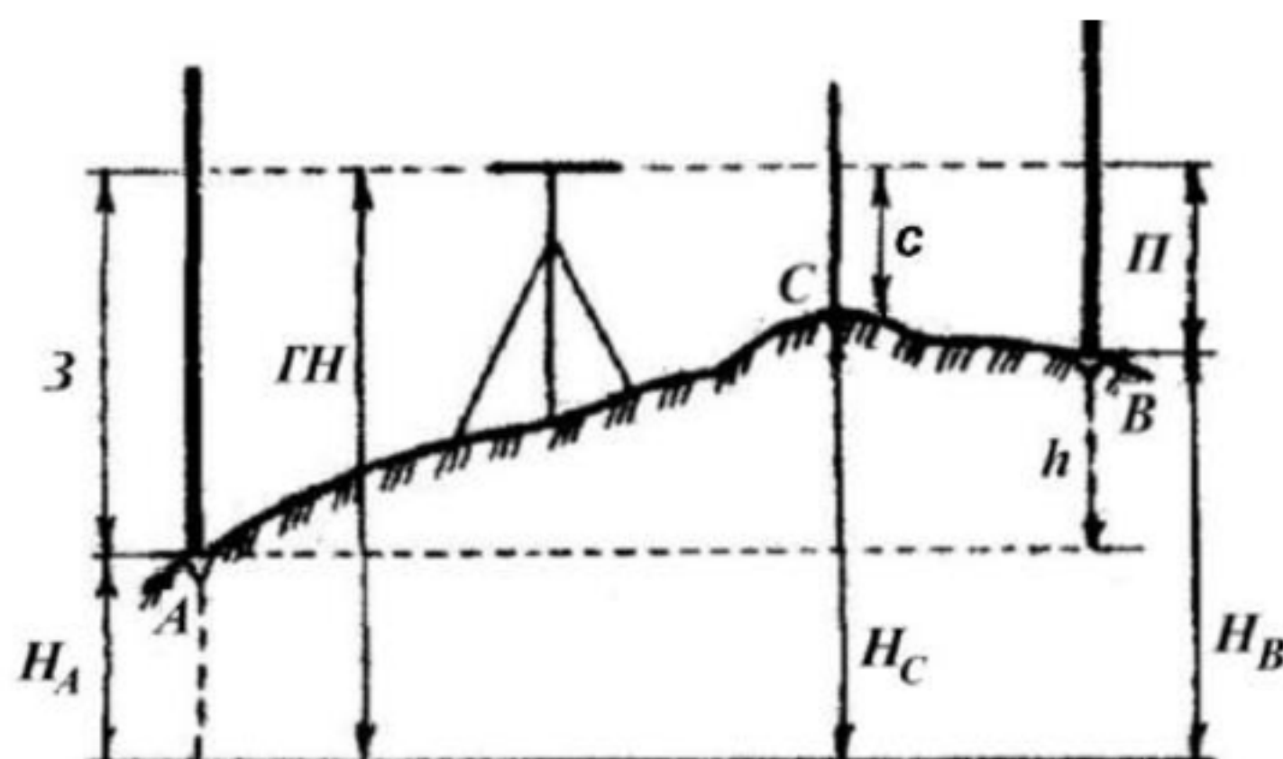
Рисунок 8 – Геометрическое нивелирование из середины
