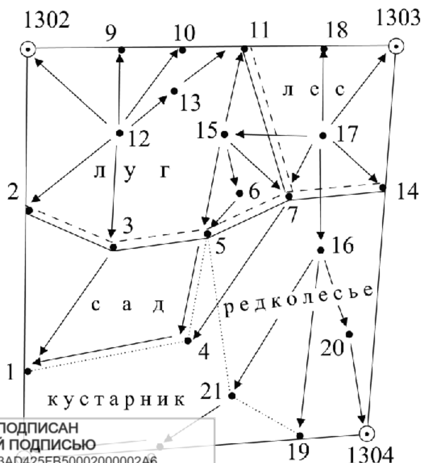
Абрис тахеометрической съемки.
