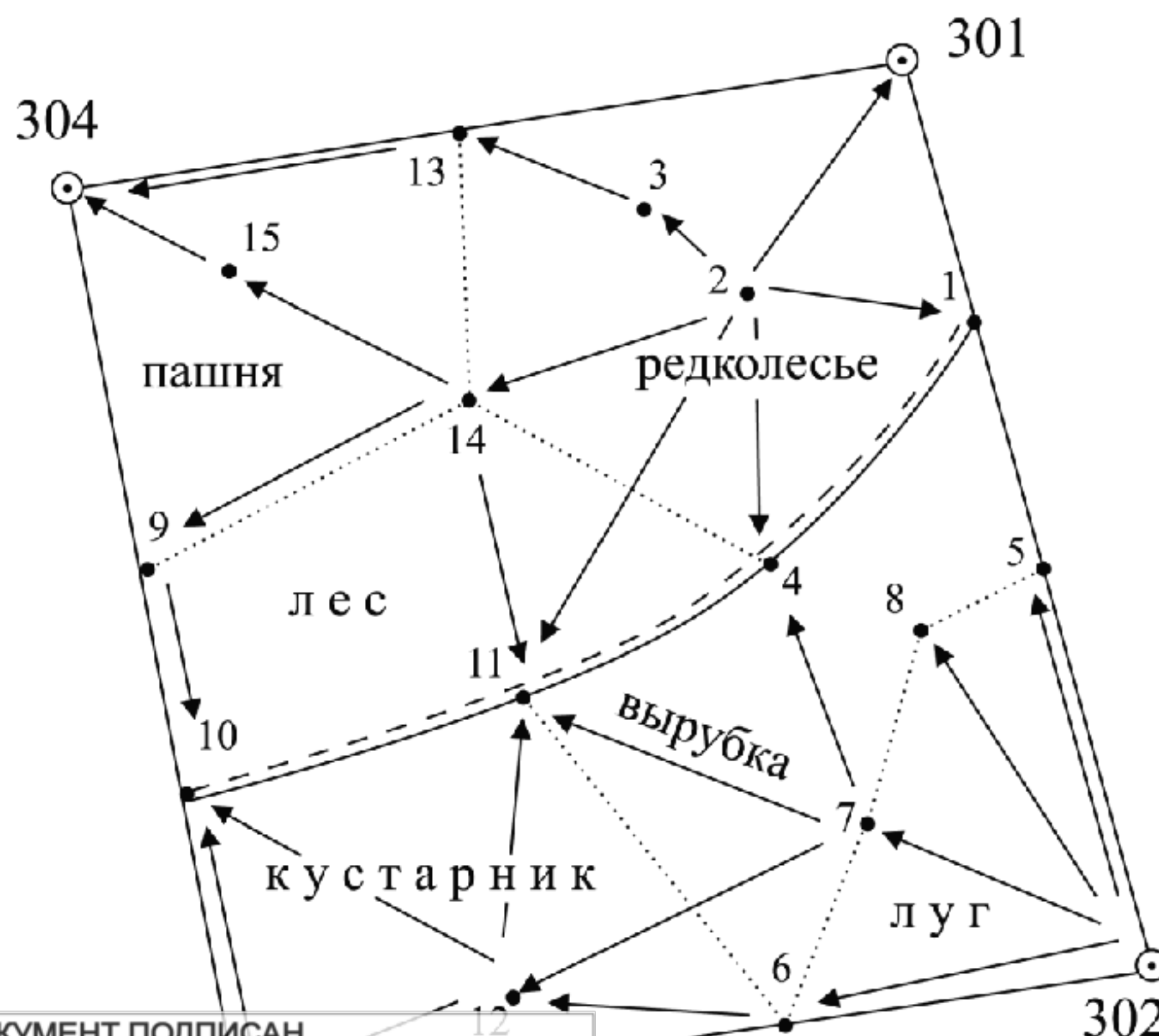
Абрис тахеометрической съемки.
