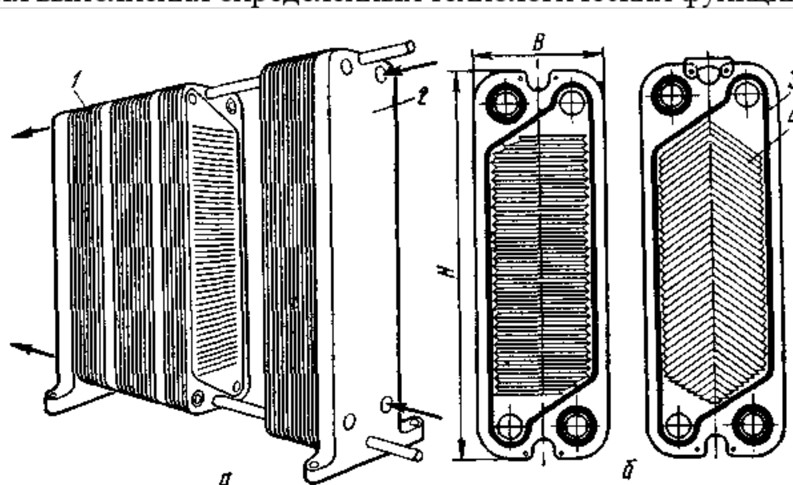
Рисунок. 11.1 - Пластинчатый теплообменник:
