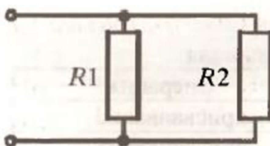
Рис. 1.4. Параллельное включение резисторов
