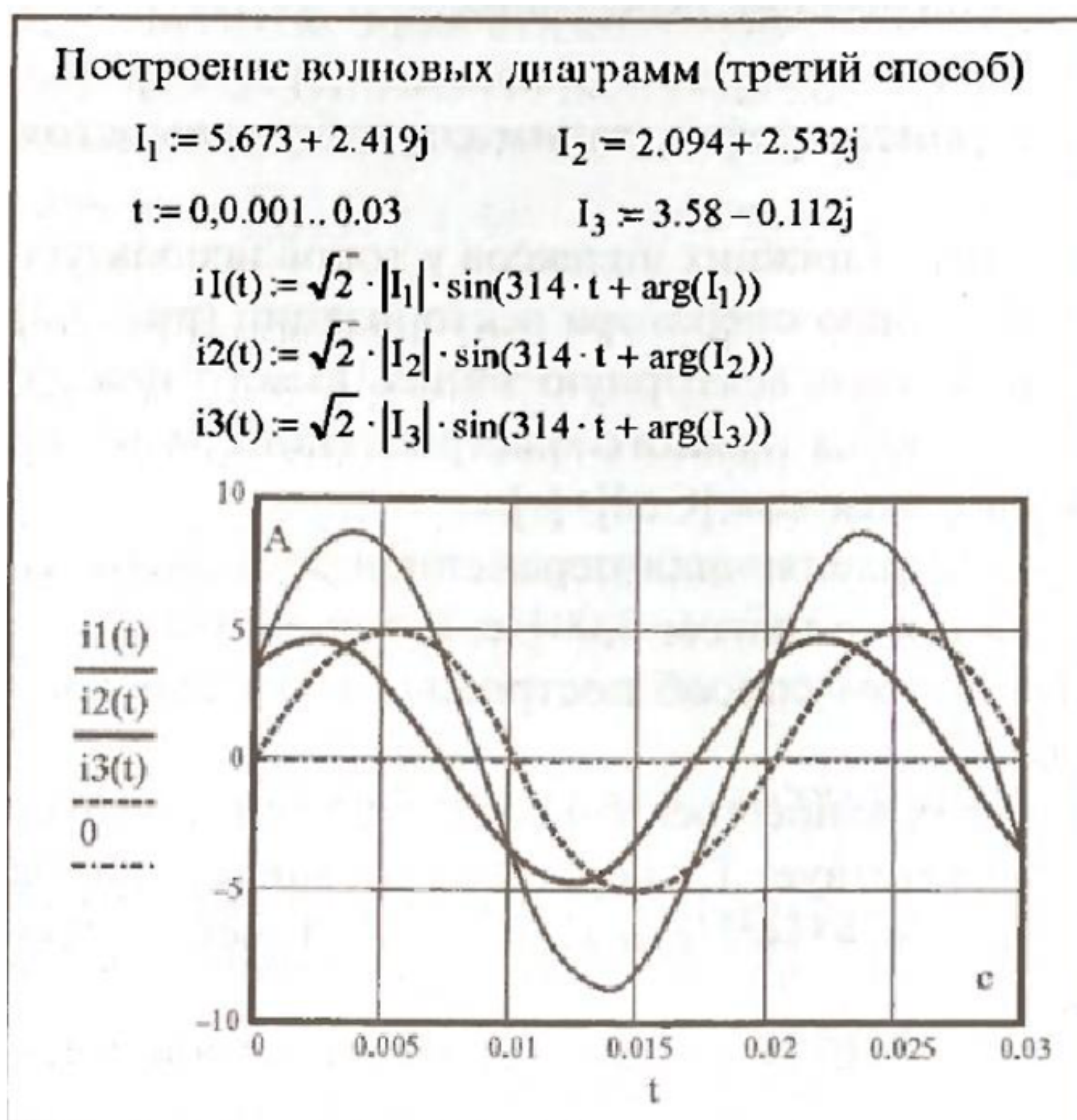
Рис. 3.3. Построение волновых диаграмм с использованием функций дискретного аргумента
