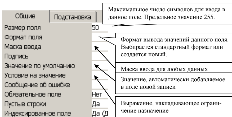
Рисунок 2. Свойства текстового поля
