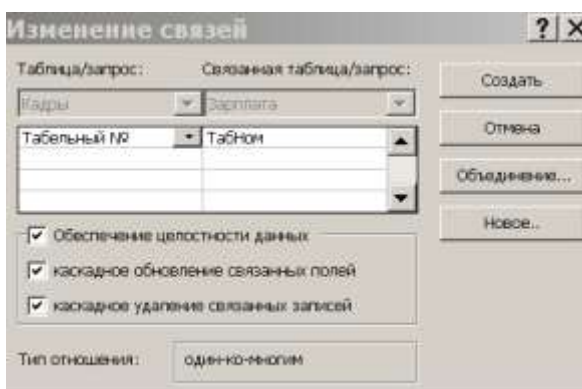
Рисунок 3. Окно установки и изменения связей
