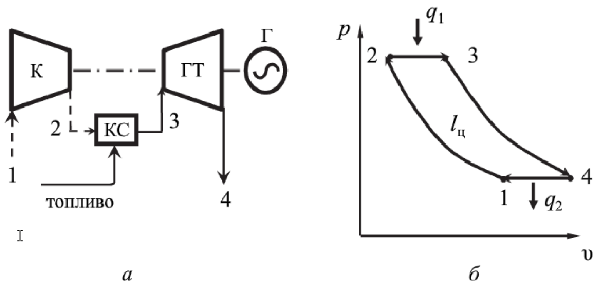
Рисунок 2.1. Схема (а) идеального цикла с изобарным подводом теплоты, (б) про-
