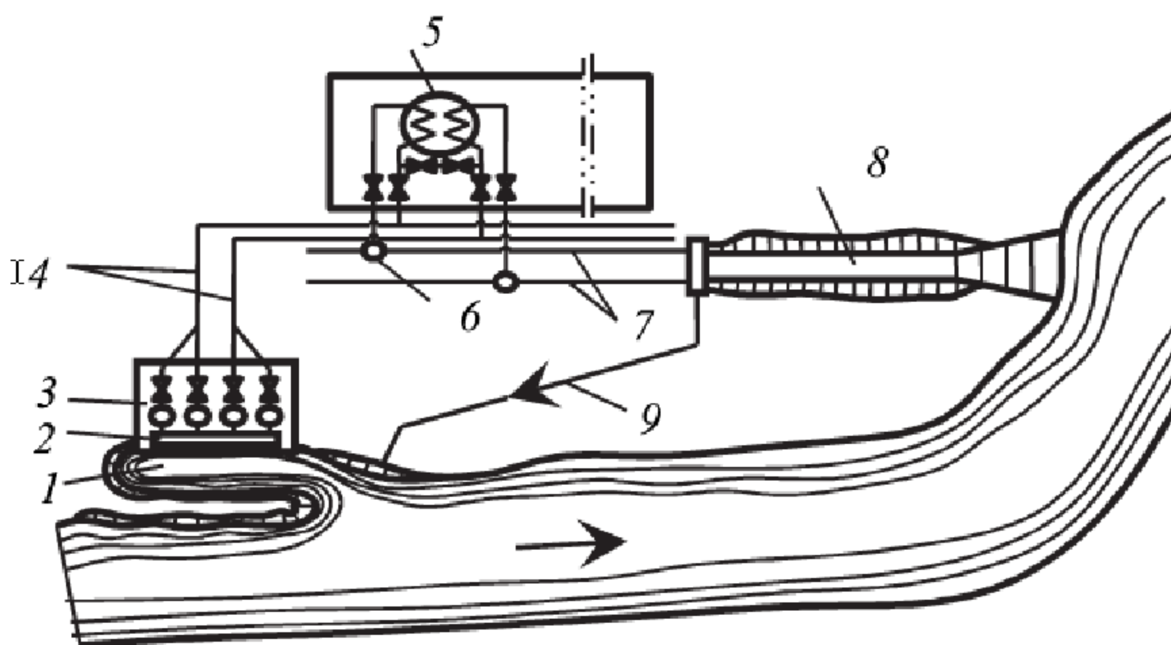
Рисунок 4.1 – Система проточного технического водоснабжения:
