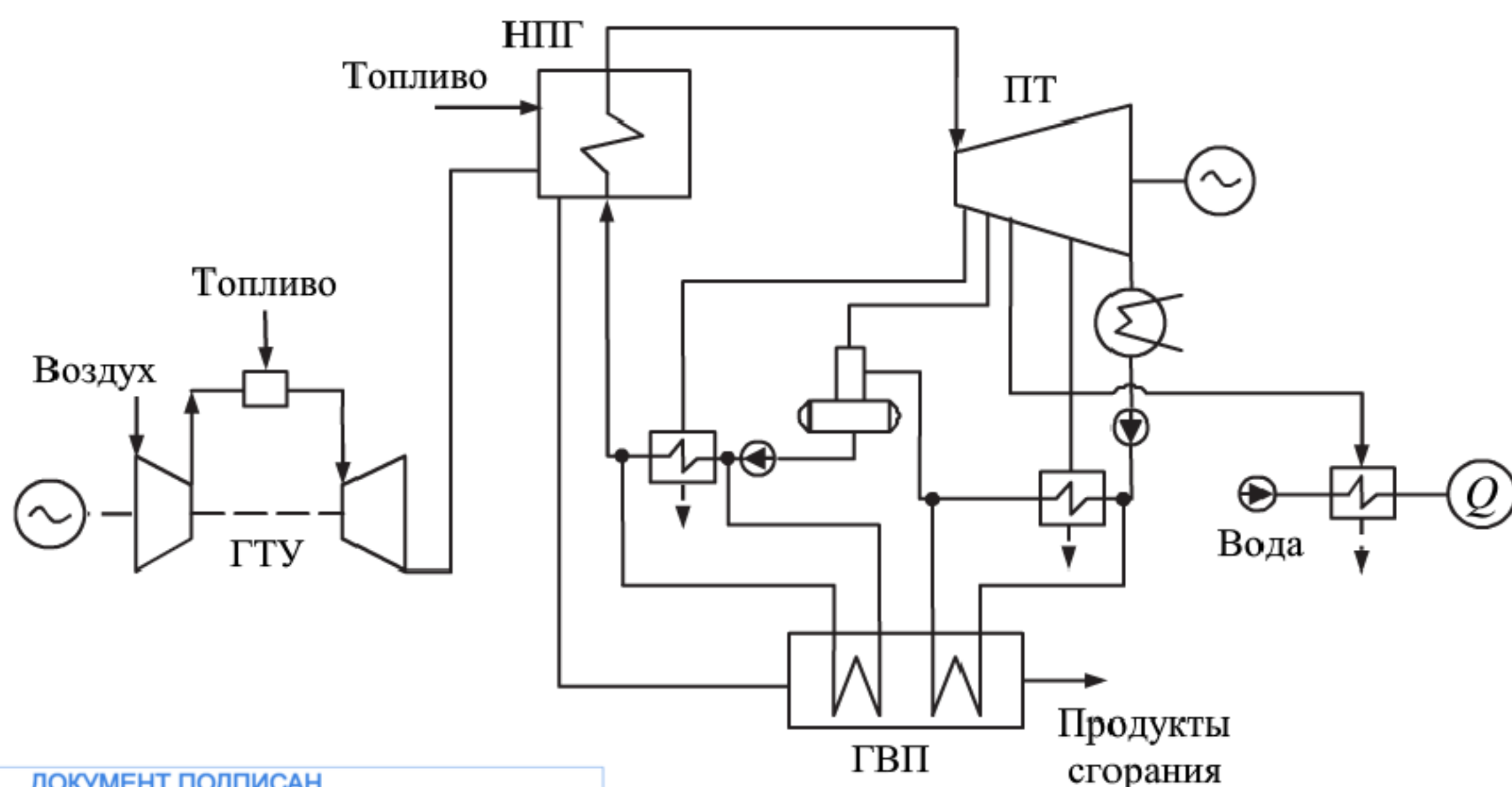
Рисунок 3.2 – Принципиальная тепловая схема ПГУ с НПП:
