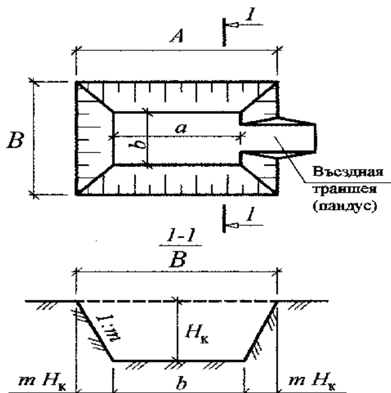
Рис. 5. Схема котлована
