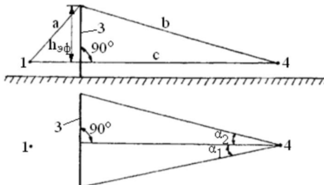
Рисунок 12.3 – Расчетная схема для определения уровня:
