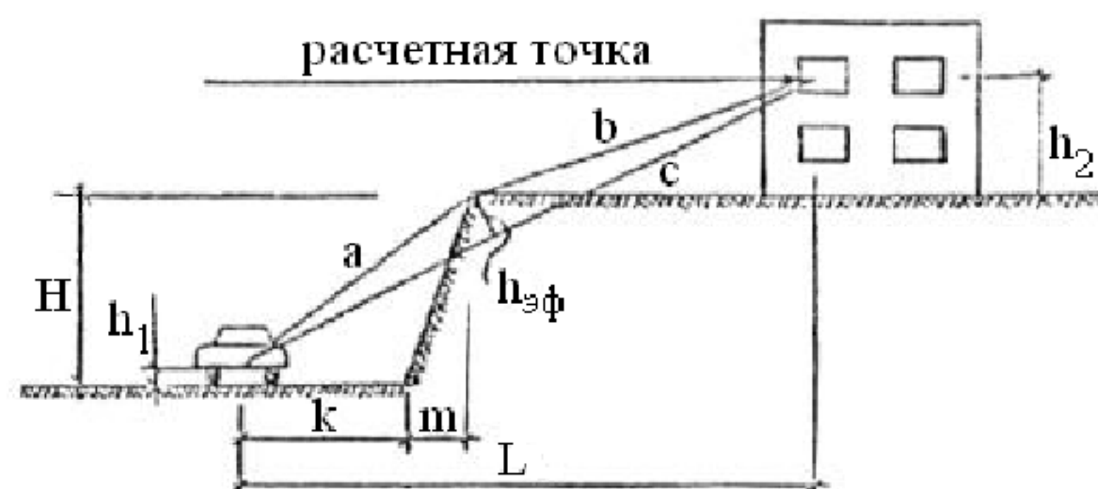
Рисунок 12.2 – Схема к расчету шумового воздействия:
