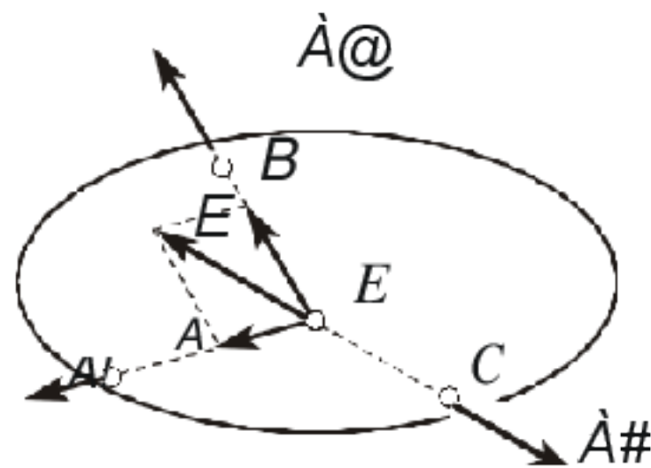
Рис. 1.11. К доказательству теоремы о трех силах
