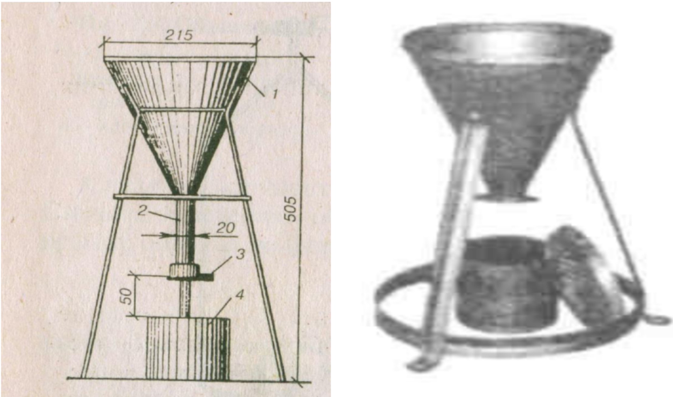
1 –корпус, 2 – трубка, 3 –задвижка, 4 – мерный цилиндр
