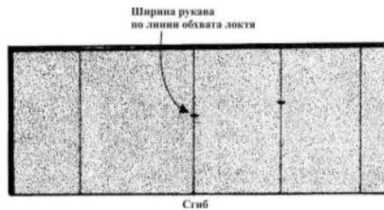
Рисунок 27 – По линии локтя отложить ширину рукава, равную половине обхвата руки в локте, плюс прибавка на свободу облегания 2 см
