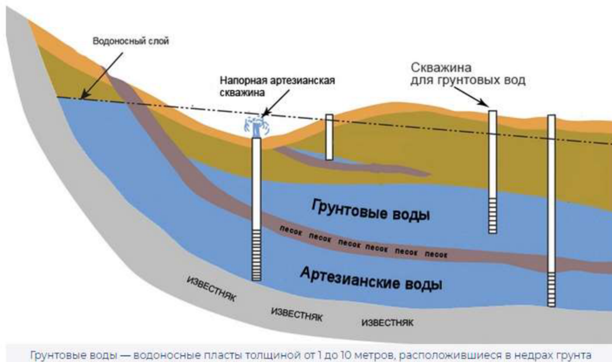
Рис.1. Схема расположения грунтовых вод
