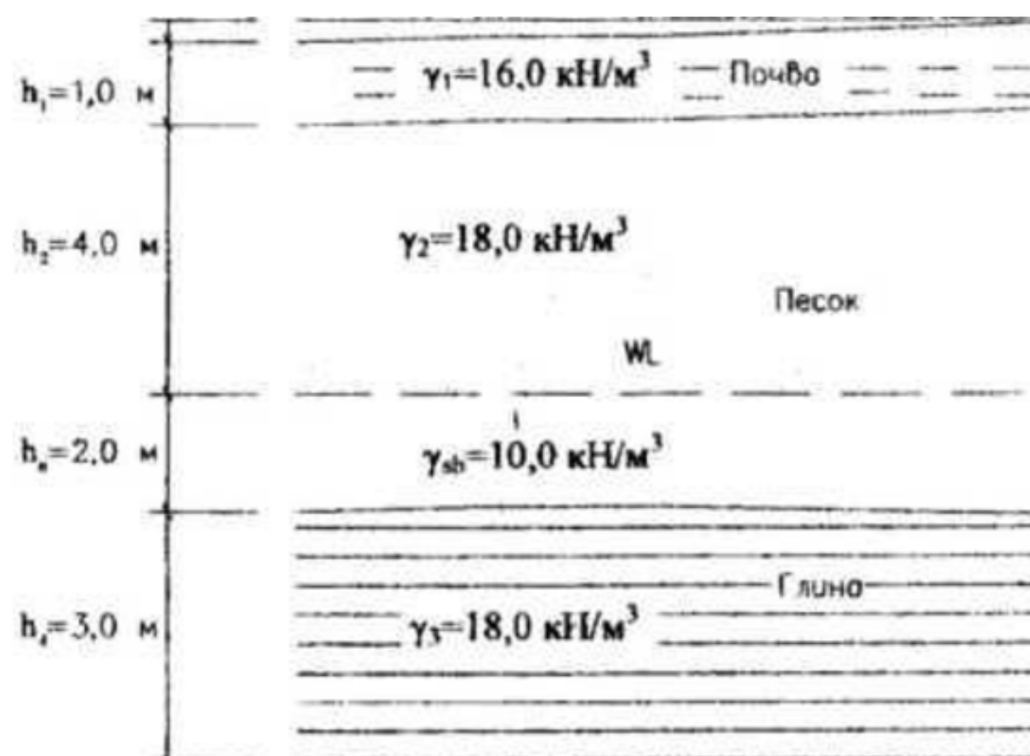
Рис. 2. Геологический разрез
