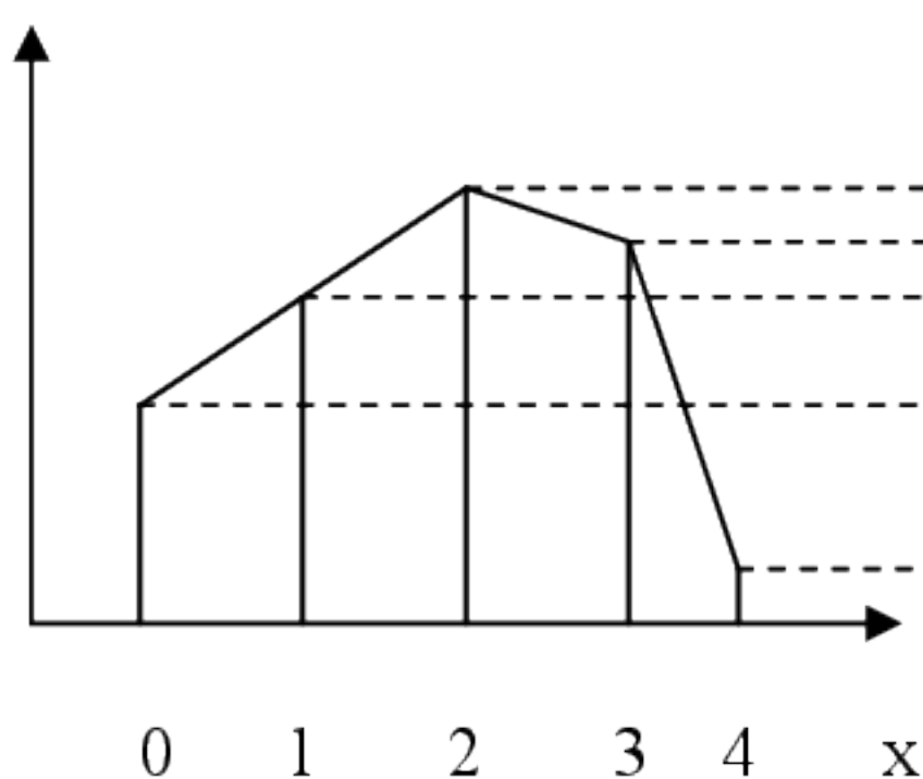
Полигон вариационного ряда
