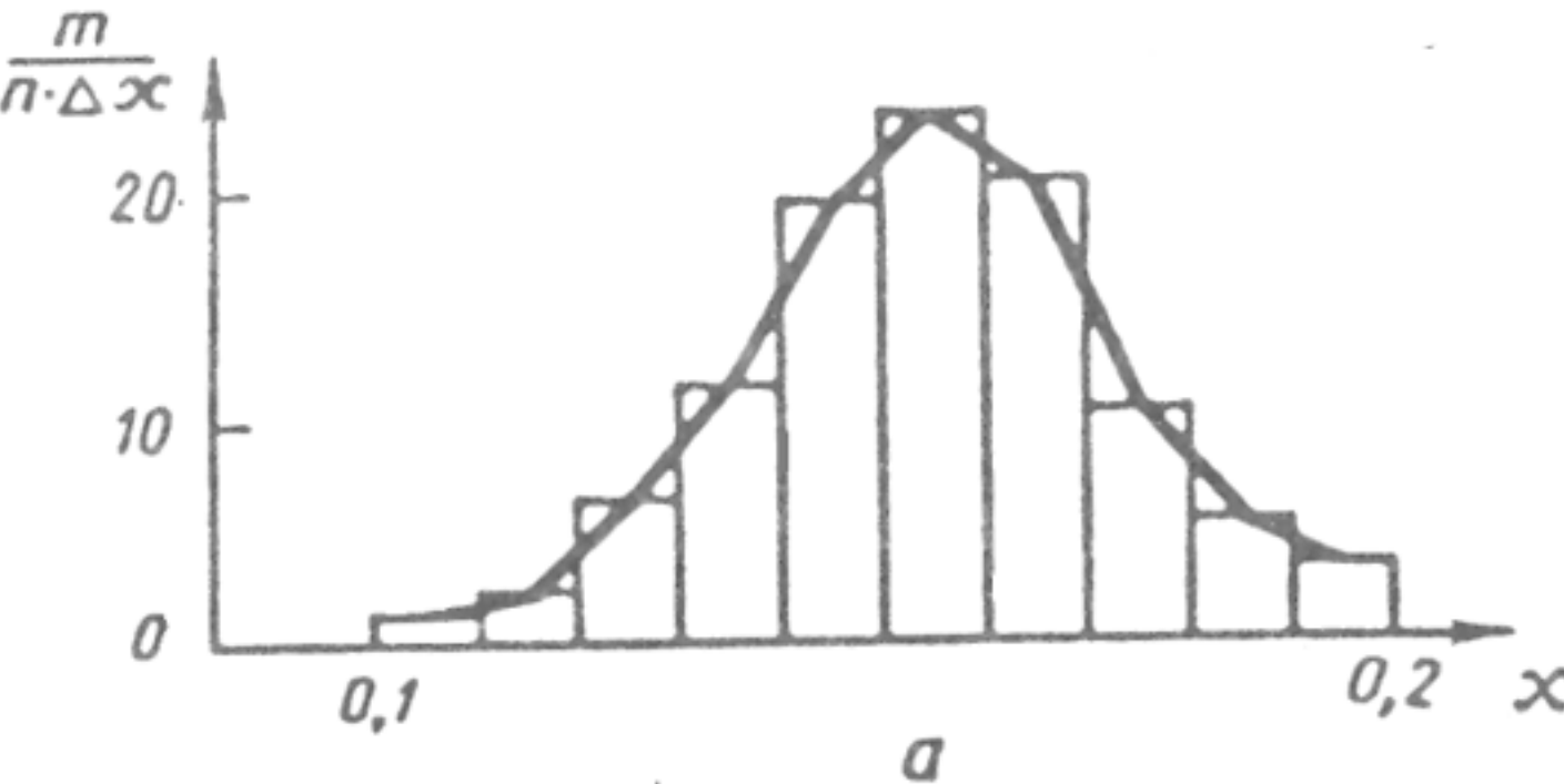
Рисунок 1 – Гистограмма и полигон аналогового измерительного прибора
