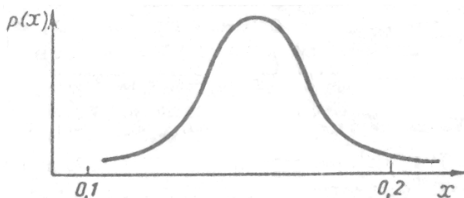
Рисунок 2 – Плотность распределения вероятности отсчета
