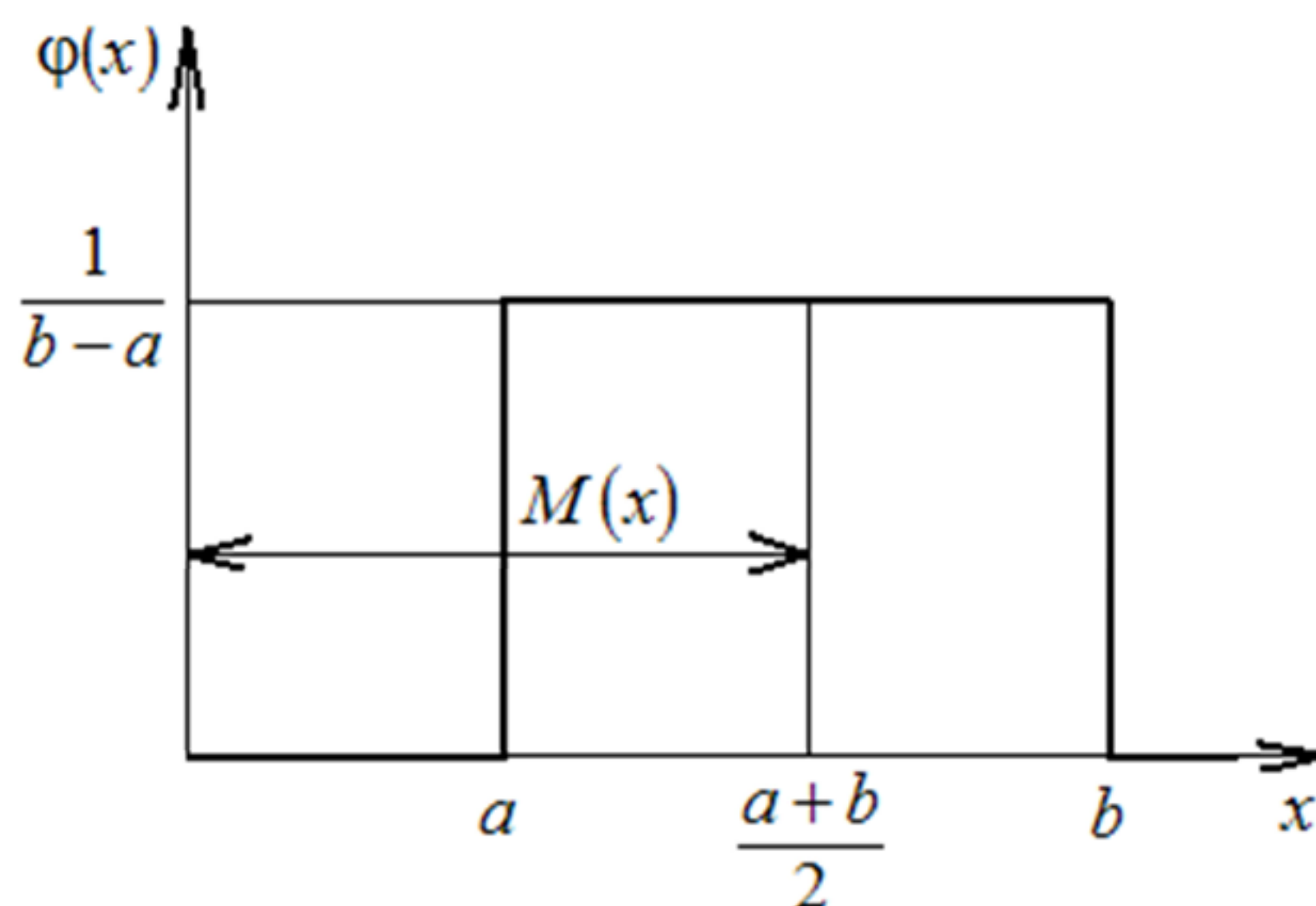
Рисунок 6 – Плотность вероятности (дифференциальная функция) равномерного распределения
