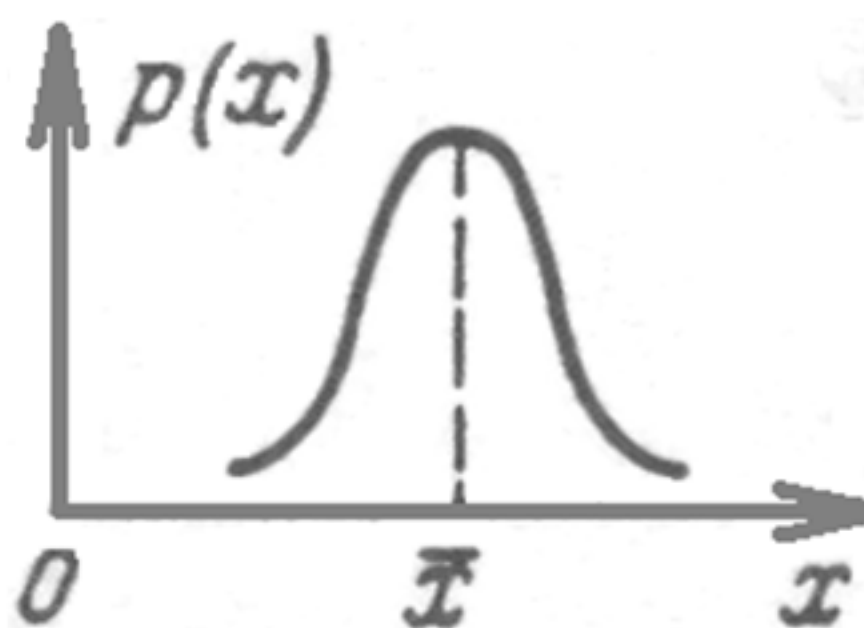
Рисунок 5 – Нормальный закон распределения
