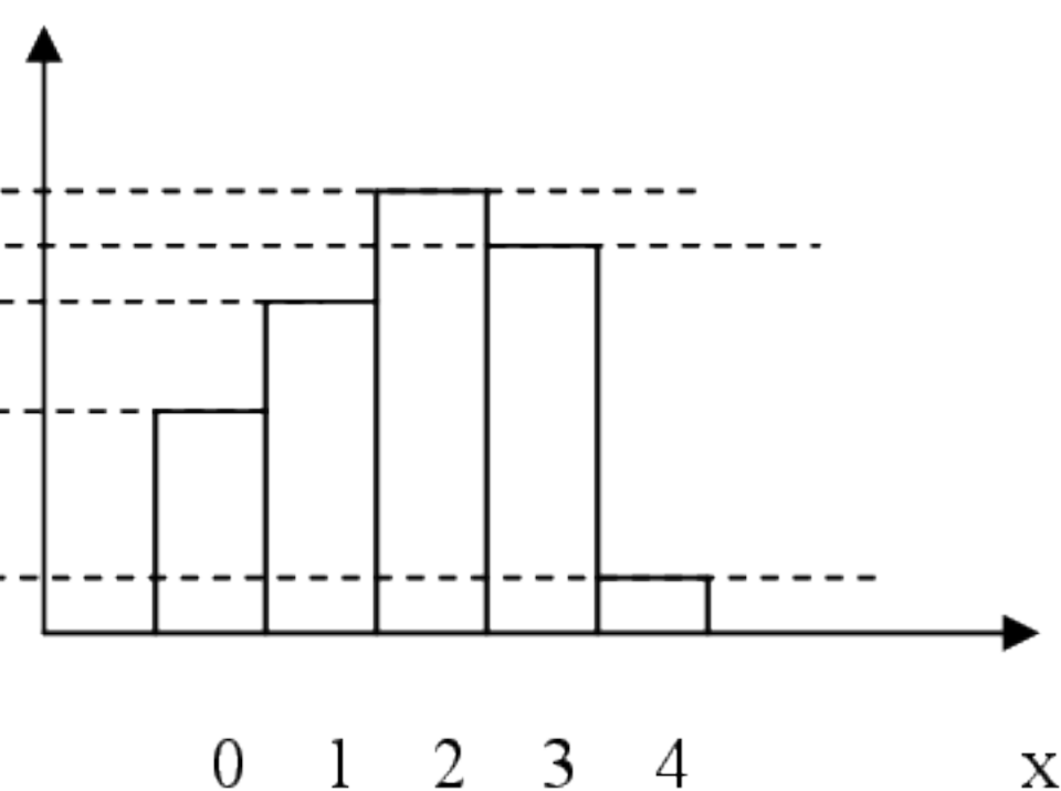
Гистограмма вариационного ряда
