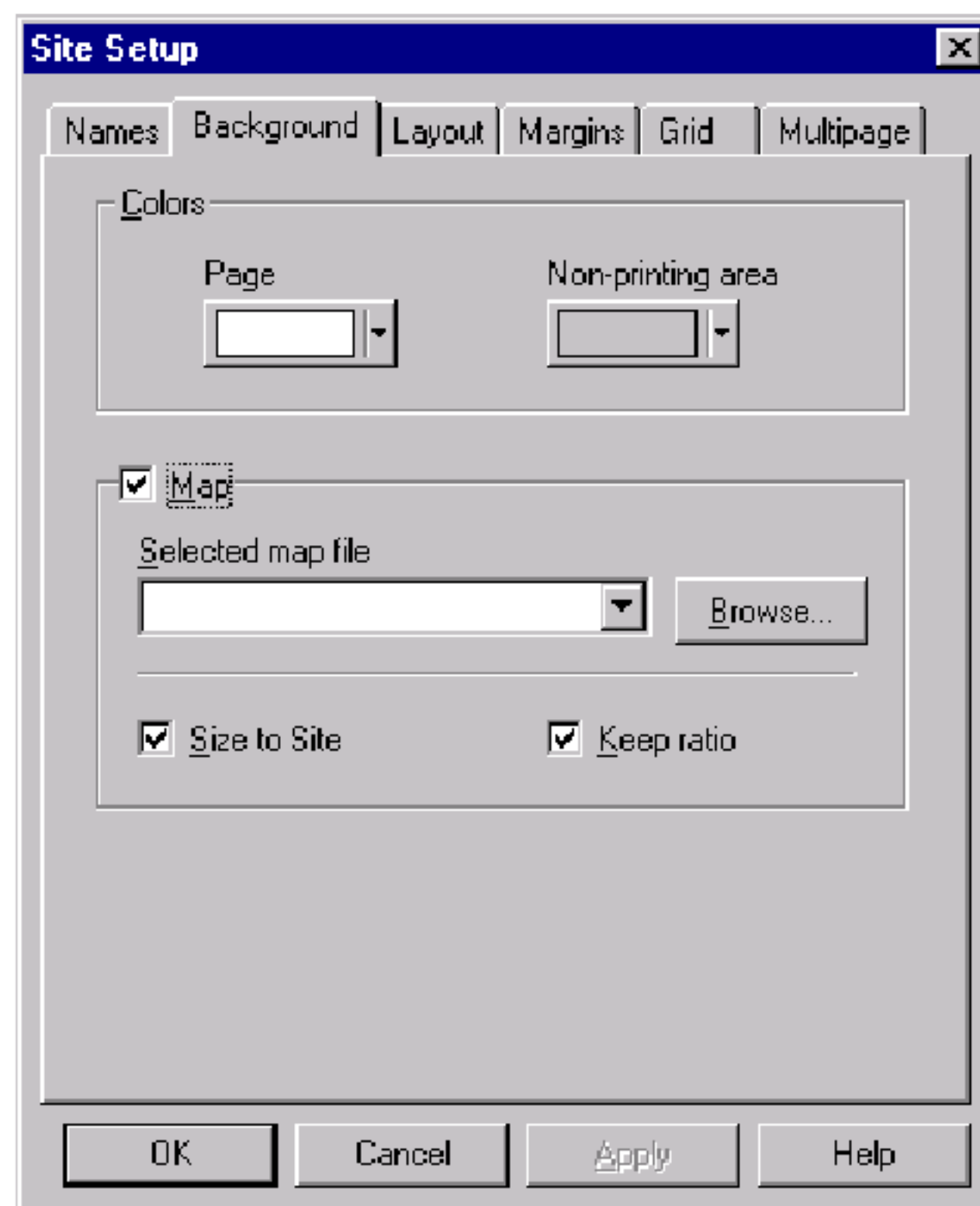
Рисунок 5.4- Диалог Установки
