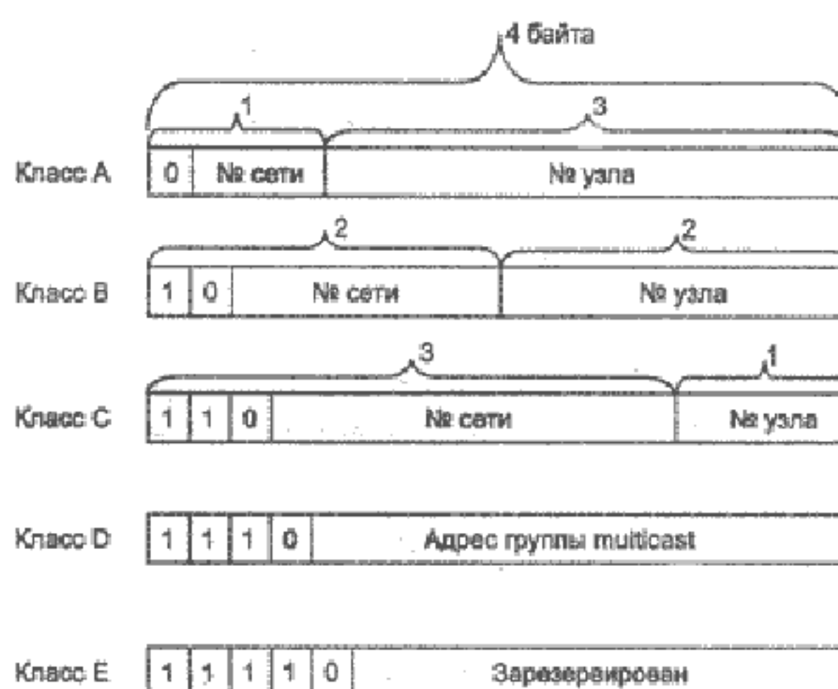
Рисунок 1.1 - Классы IP-адресов
