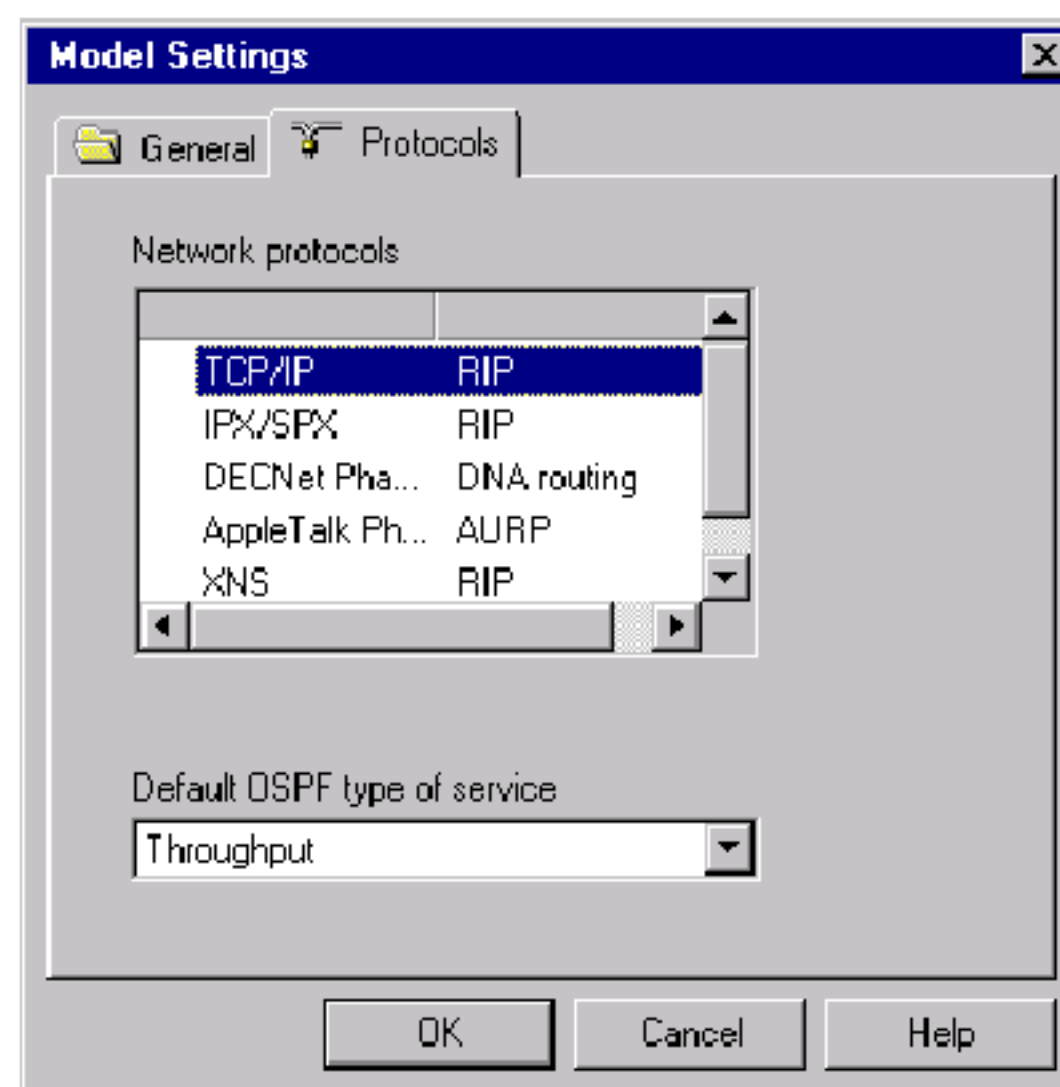
Рисунок 4.5 - Вкладка Protocols в окне-диалоге настроек модели
