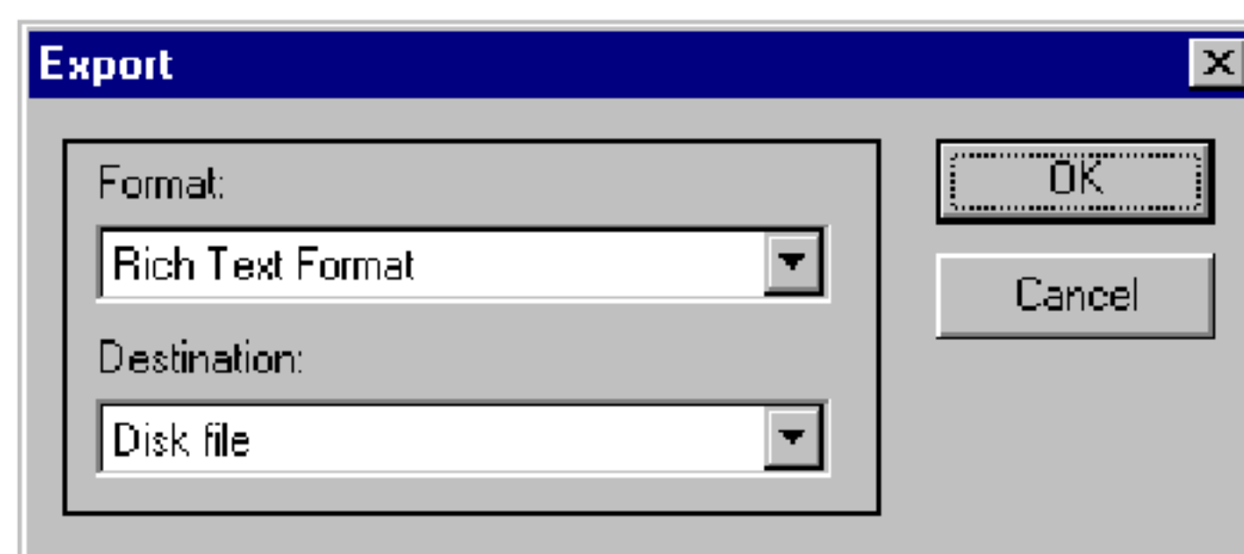
Рисунок 3.16 - Экспортный диалог
