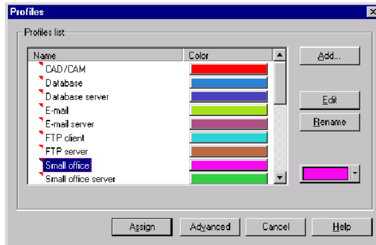
Рисунок 5.3 - Диалог конфигурации
