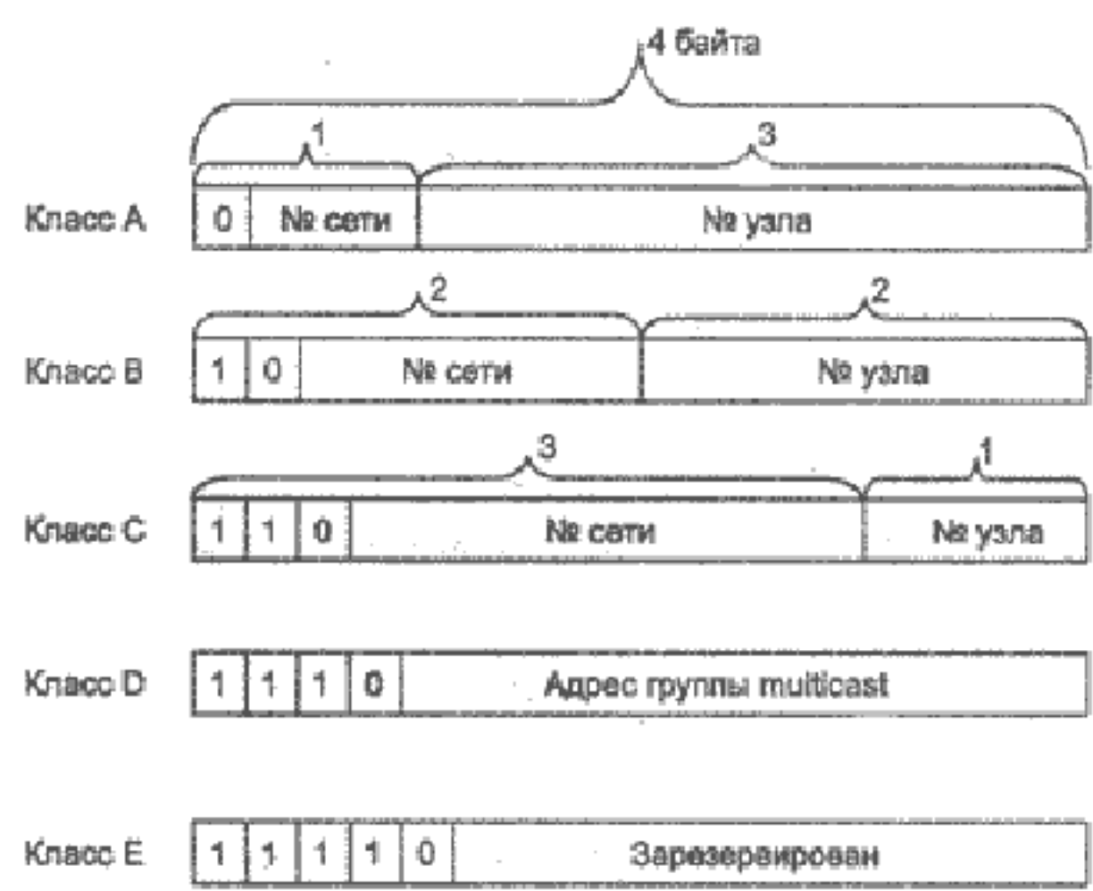
Рисунок 1.1 - Классы IP-адресов
