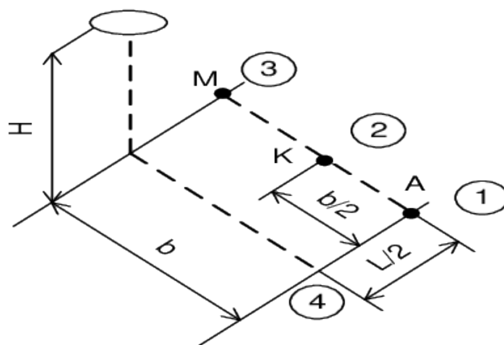
Рис.16. Иллюстрация к определению координат контрольных точек
