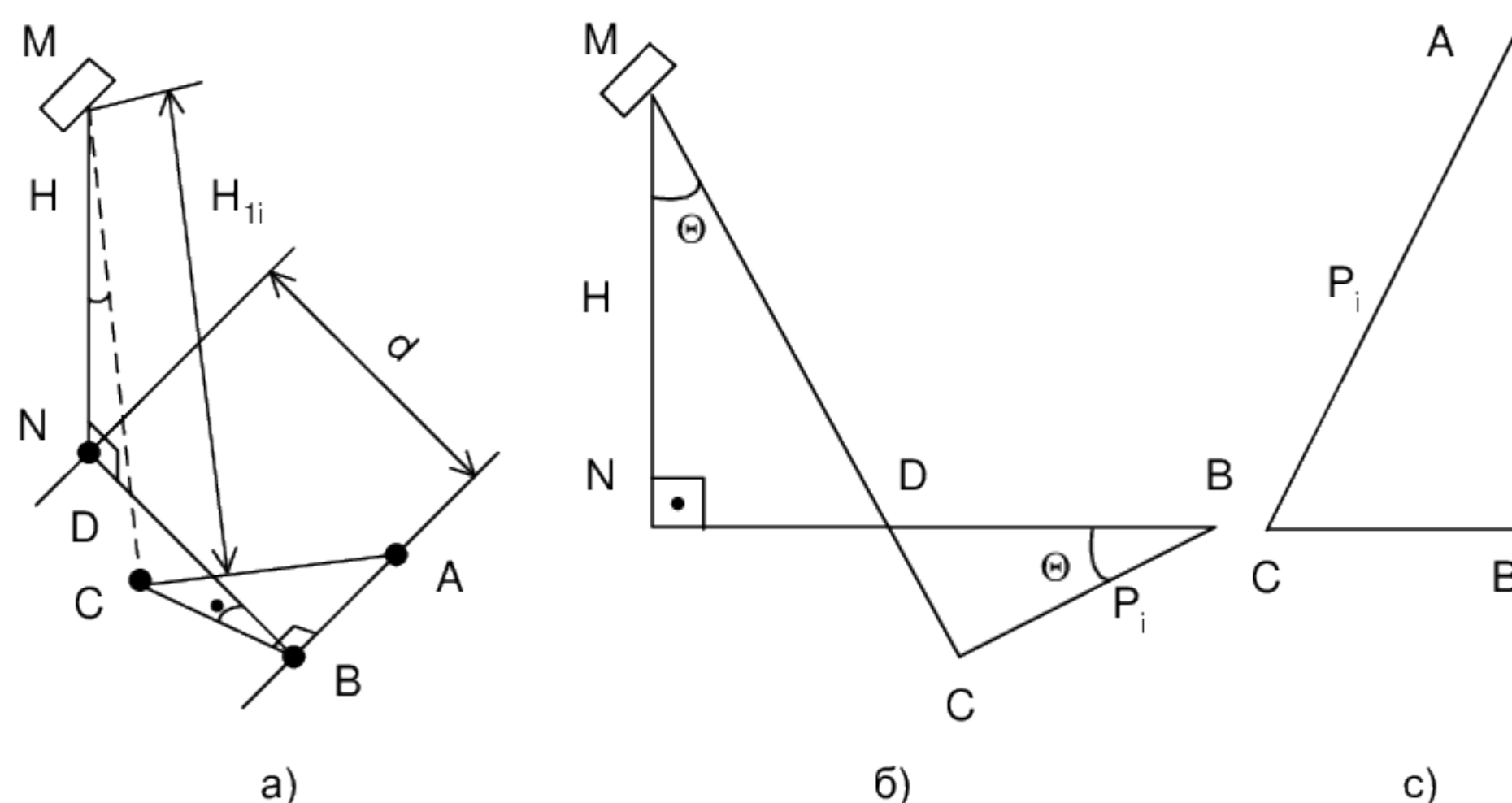
Рис.15. К определению освещенности от консольного светильника
