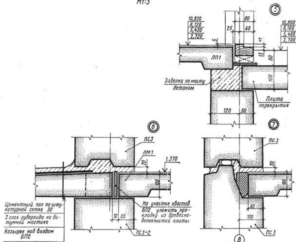
Узлы лестницы М1:5
