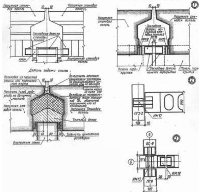
Соединение наружных стеновых панелей с панелями перекрытия
