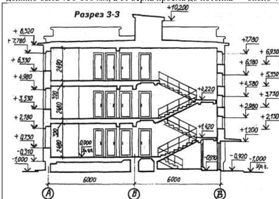
Рисунок 10.1 Архитектурный разрез
