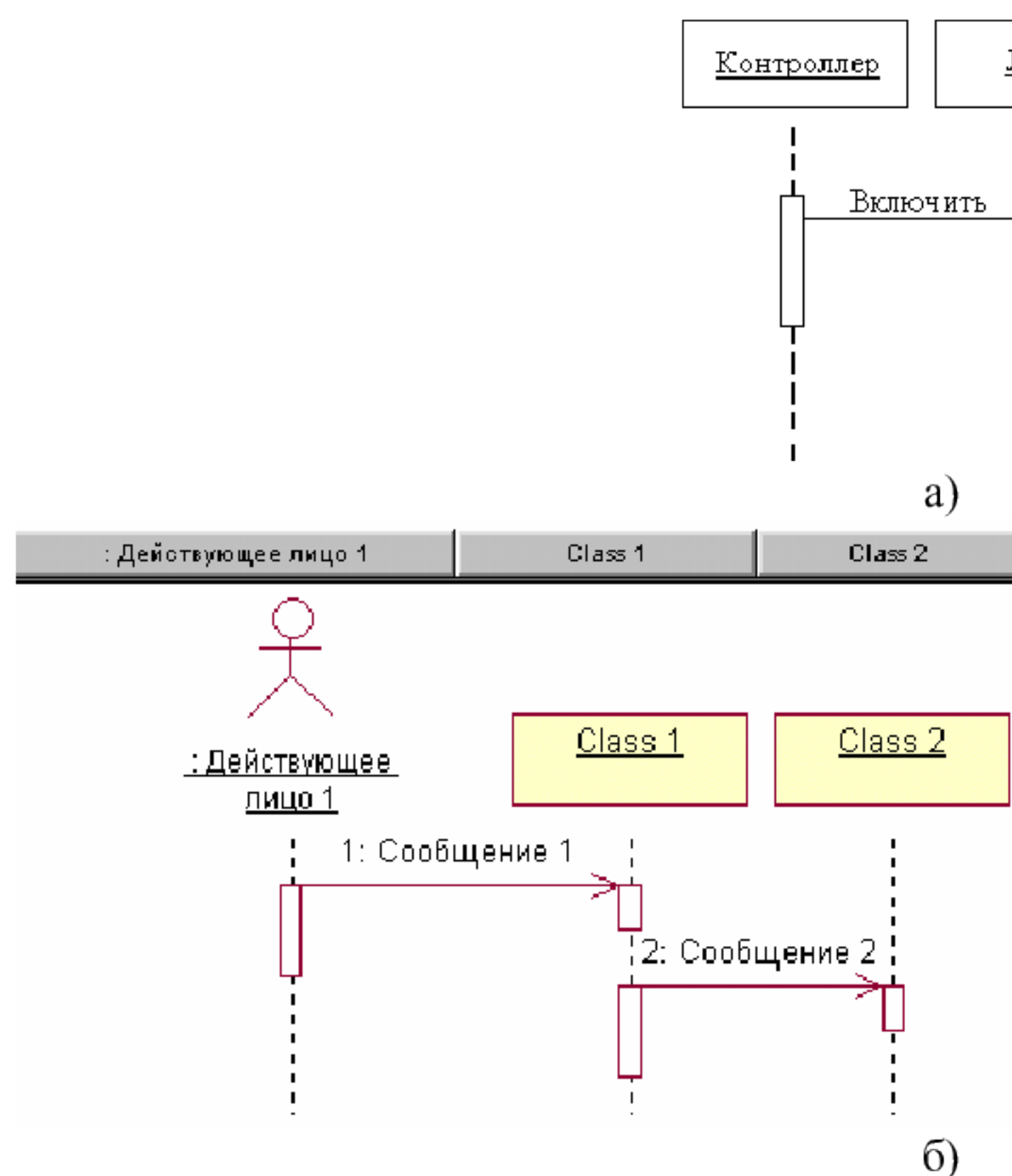
Рисунок 1 – Примеры Sequence диаграмм
